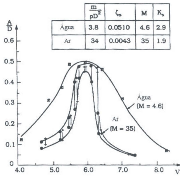
Figura 2.19: Efeito da razão de massa, m^* , na variação da amplitude de oscilação com a velocidade reduzida (Sumer e Fredsøe, 1997 [31]).
