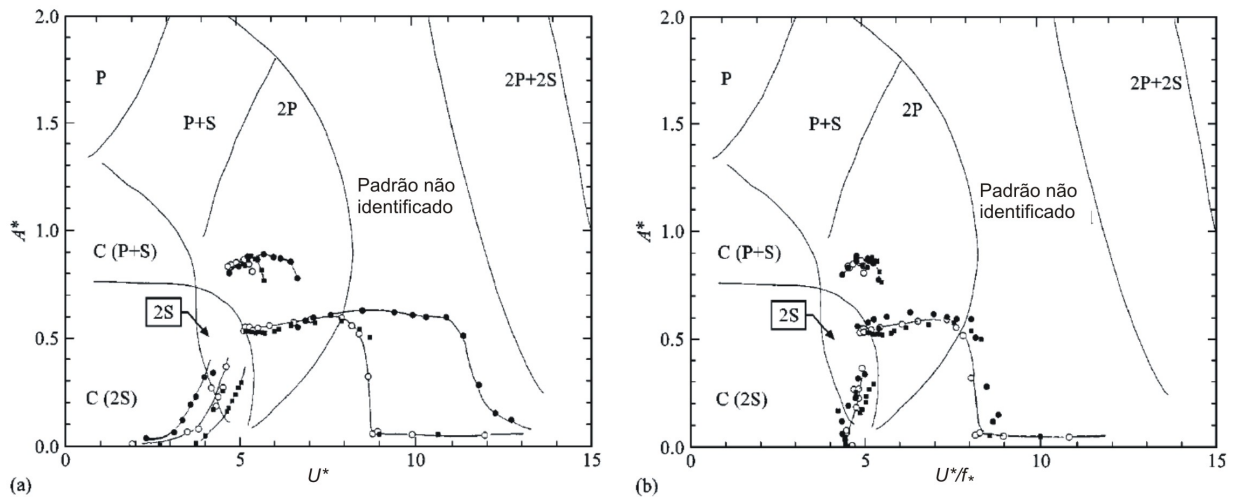
Figura 2.21: Resultados de Khalak e Williamson (1999[13]) para valores de m^*\zeta entre 0,014 e 0,019, e m^* variando de 2,4 (●); 10,3 (○); e 20,6 (■). (a) Variação da amplitude máxima em função da velocidade normalizada. (b) Variação da amplitude máxima em função da velocidade reduzida.
