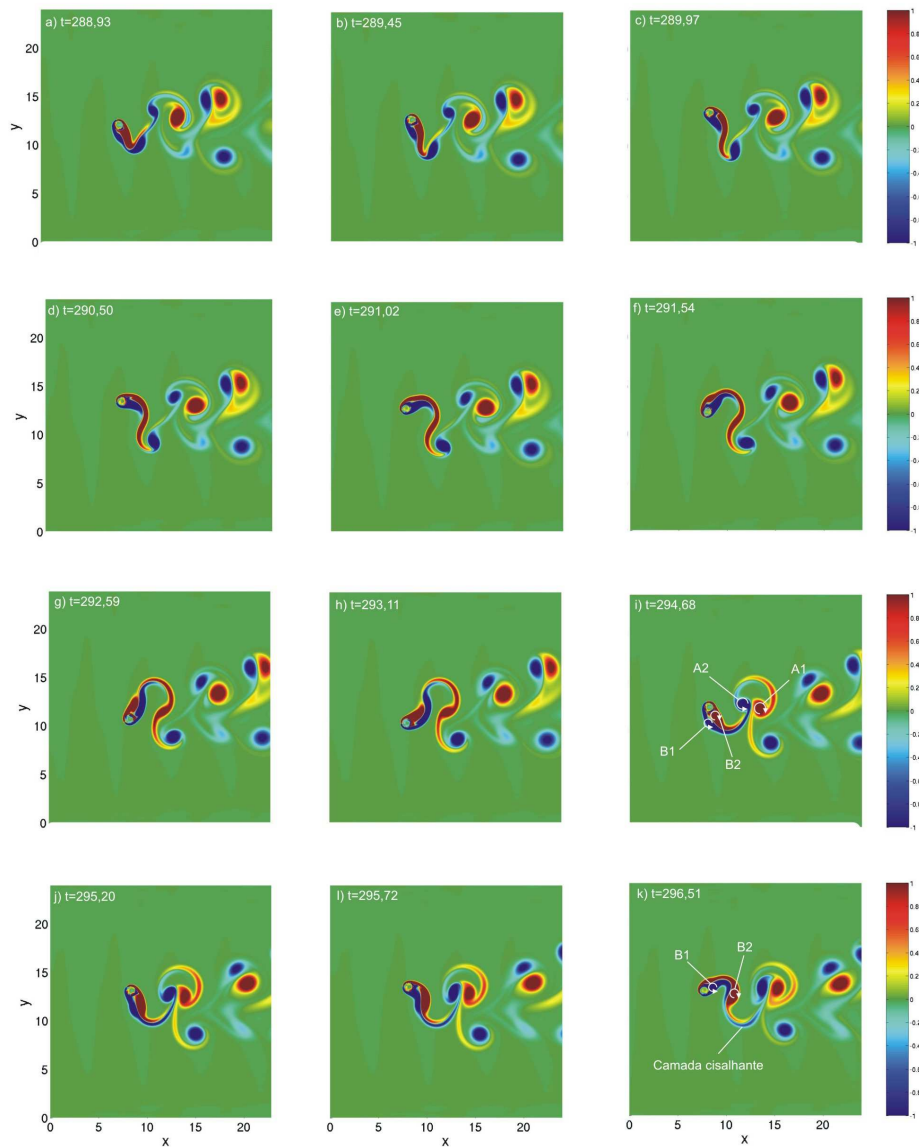
Figura 6.8: Campos instantâneos de vorticidade para um ciclo de oscilação da Simulação O-I (Trajetória sobre curva em oito).
