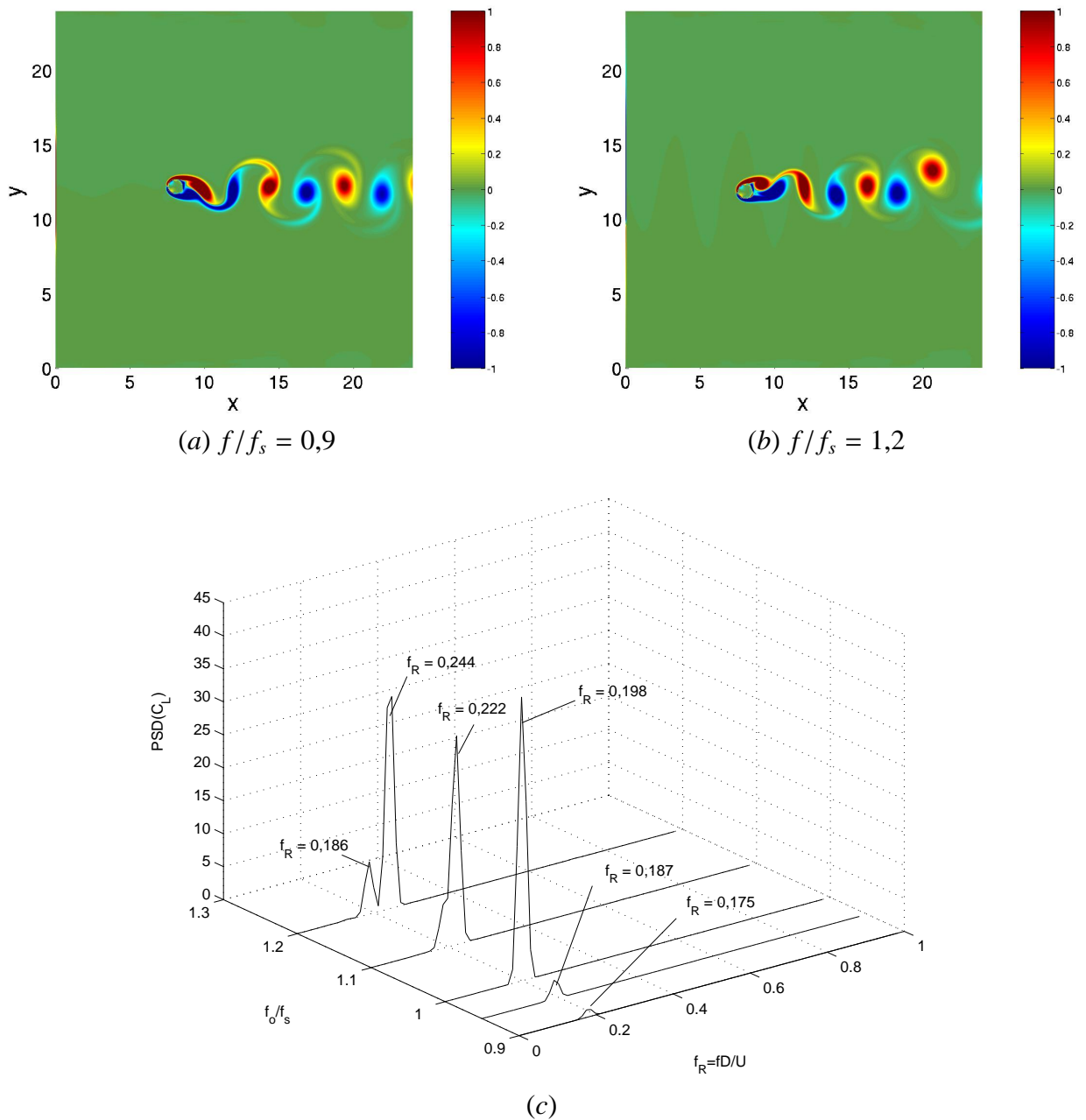
Figura 4.9: (a) Campo instantâneo de vorticidade para a simulação II ( f/f_s = 0,9 ); (b) Campo instantâneo de vorticidade para a simulação VI ( f/f_s = 1,2 ); (c) Densidade espectral de potência para o sinal do coeficiente de sustentação das simulações de I à VI.
