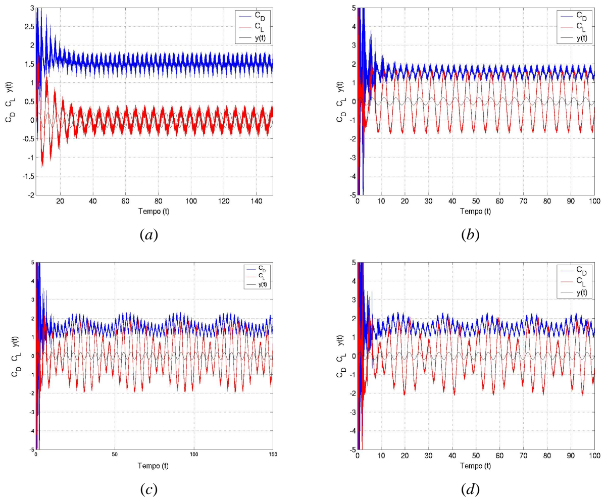
Figura 4.8: Sinais de C_D , C_L e deslocamento do cilindro y(t) ; (a) f_o/f_s = 0,9 ; (b) f_o/f_s = 1,0 ; (c) f_o/f_s = 1,1 ; (d) f_o/f_s = 1,2 .
