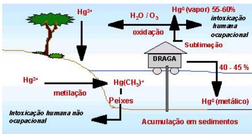
Figura 1. Processos ambientais envolvendo o Hg após sua emissão para o meio ambiente
