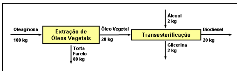
Figura 22. Balanço de Massa do Processo de Produção de Biodiesel.
