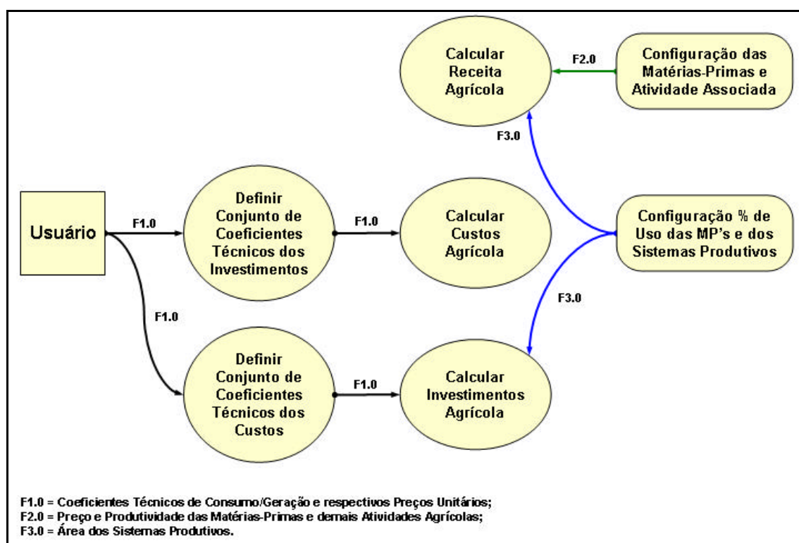
Figura 27. Diagrama de Fluxo de Dados da Orçamentação do Elo Agrícola.
