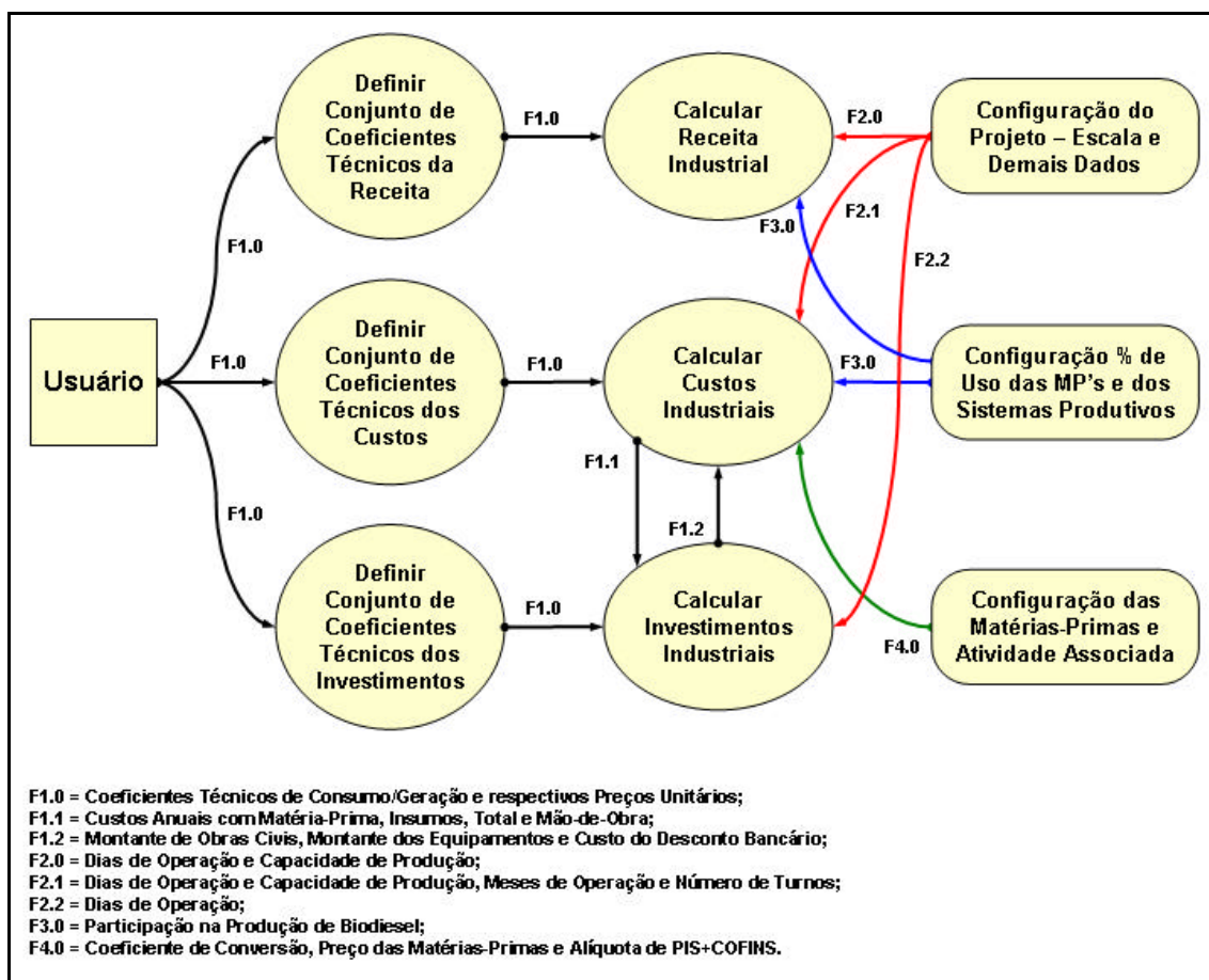
Figura 23. Diagrama de Fluxo de Dados da Orçamentação do Elo Industrial.
