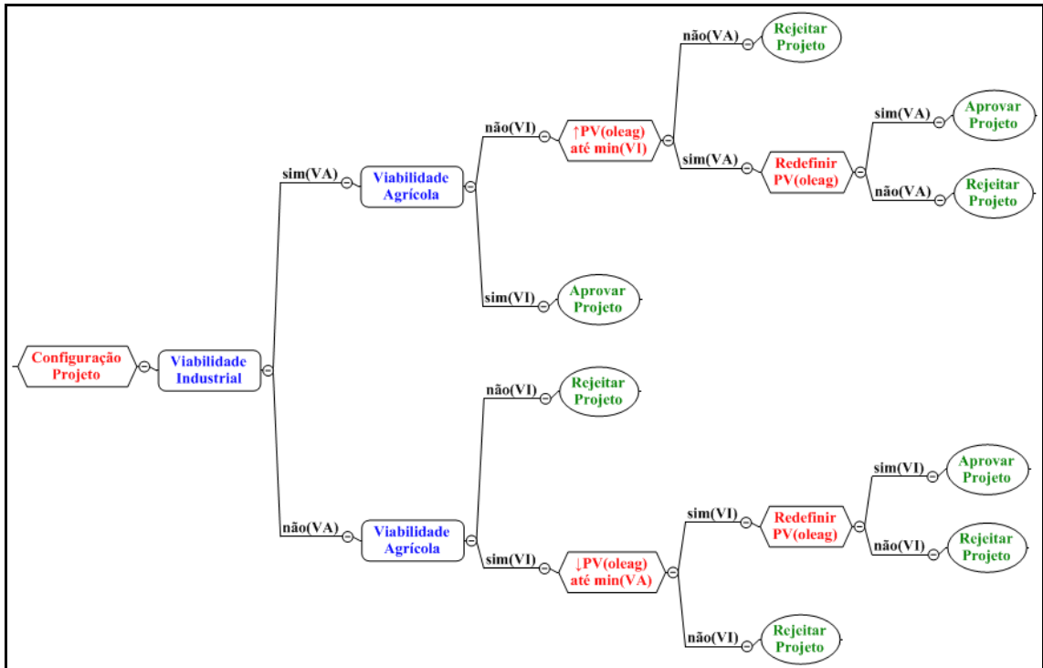
Figura 10. Árvore de Decisão de Projetos Agroindustriais de Biodiesel.
