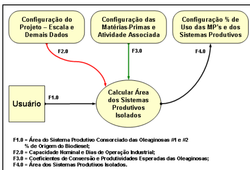
Figura 17. Diagrama de Fluxo para Definir o Tamanho do Elo Agrícola.
