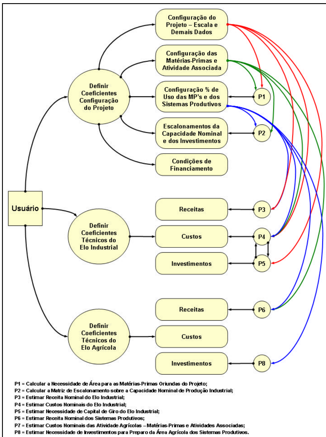
Figura 11. Diagrama de Fluxo de Dados das Planilhas de Configuração do Projeto.
