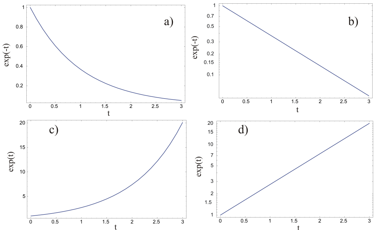
Figura 1.1: Em a), vemos a representação do decrescimento exponencial em escala linear e, em b), o mesmo decrescimento em um gráfico mono-log. Em c), o crescimento exponencial com escala linear é exibido, e em d), com escala mono-log.
