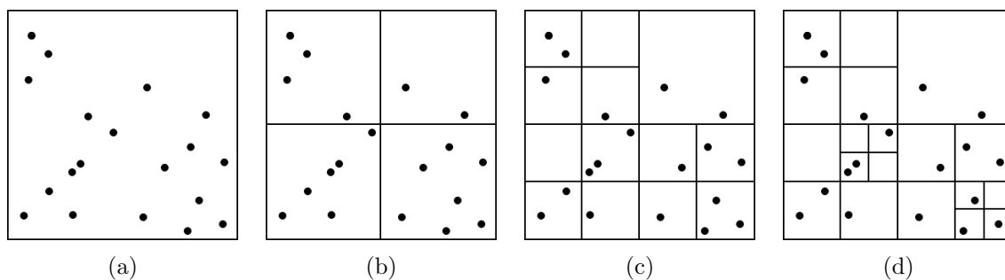
Figura 2.6: Exemplo de uma divisão do plano por uma quadtree; (a) Dados de entrada. (b) Primeiro nível, note que somente o segundo quadrante satisfaz o critério de parada, isto é, possui no máximo dois pontos. (c) Segundo nível. (d) Terceiro nível, todo plano está dividido em regiões com o máximo dois pontos.
