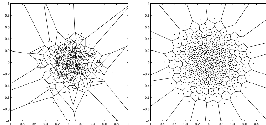
Figura 2.4: Diagrama de Voronoi Centroidal com função de densidade e^{-10x^2 - 10y^2} para um conjunto de pontos escolhidos de maneira aleatória em [-1, 1]^2 ; a esquerda, o Diagrama de Voronoi; à direita o Diagrama de Voronoi Centroidal; 256 geradores [8].
