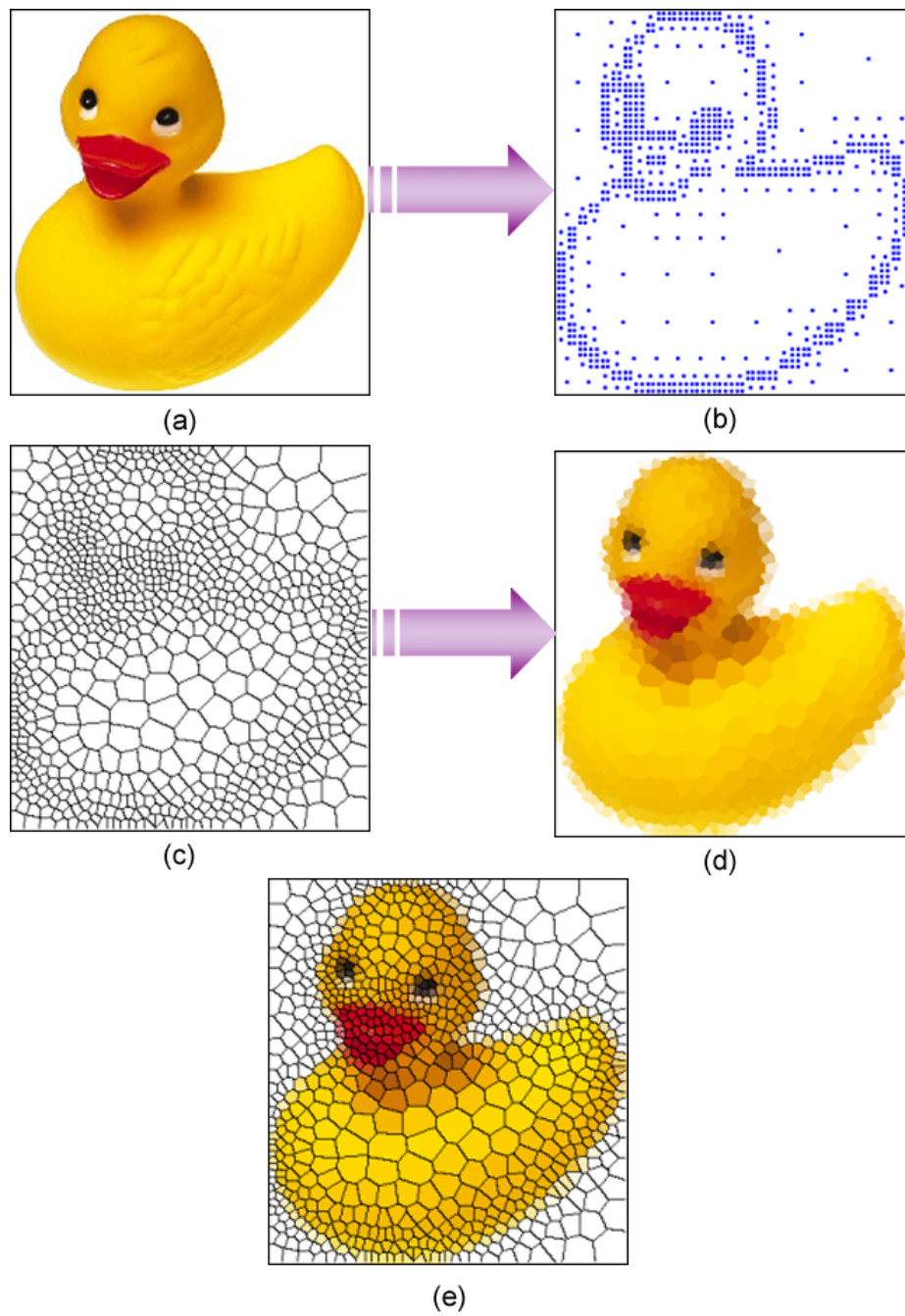
Figura 3.1: O algoritmo. (a) Imagem original, (b) Pontos amostrados, (c) Diagrama de Voronoi Centroidal (d) Imagem colorida de acordo com a área de cada região Voronoi, (e) Imagem final.
