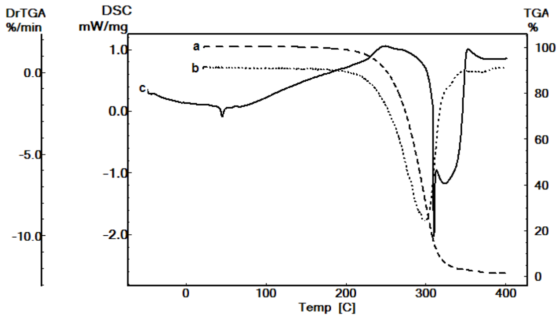
Figura 9. Curvas referentes ao polímero PLA (a) TG, (b) DTG e (c) DSC.
