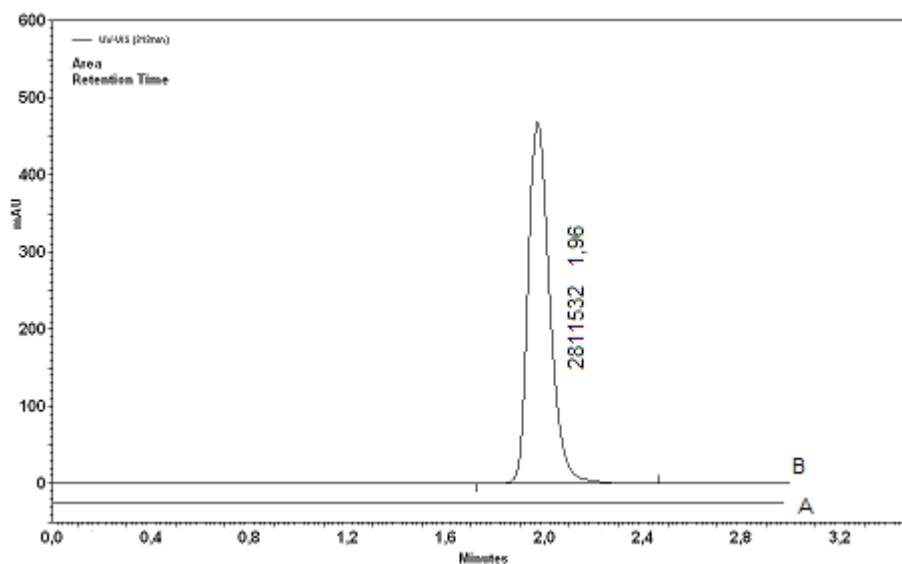
Figura 8. Cromatogramas típicos obtidos por CLAE. (A) Nanocápsulas brancas de PLA-PEG. (B) Nanocápsulas de PLA-PEG contendo 30 \mu\text{g/mL} de MTX.
