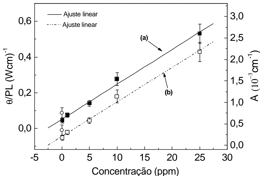
Figura 2.13 - (a) Amplitude da LT normalizada pela espessura da amostra pela potência do feixe de excitação ( \theta/PL ) em função da concentração de ferro sob forma de cloreto para \lambda_e=476\text{nm} ; (b) coeficiente de absorção óptica ( A ) em função da concentração. O símbolo (o) representa os dados da solução branco. Medidas realizadas na configuração otimizada.
