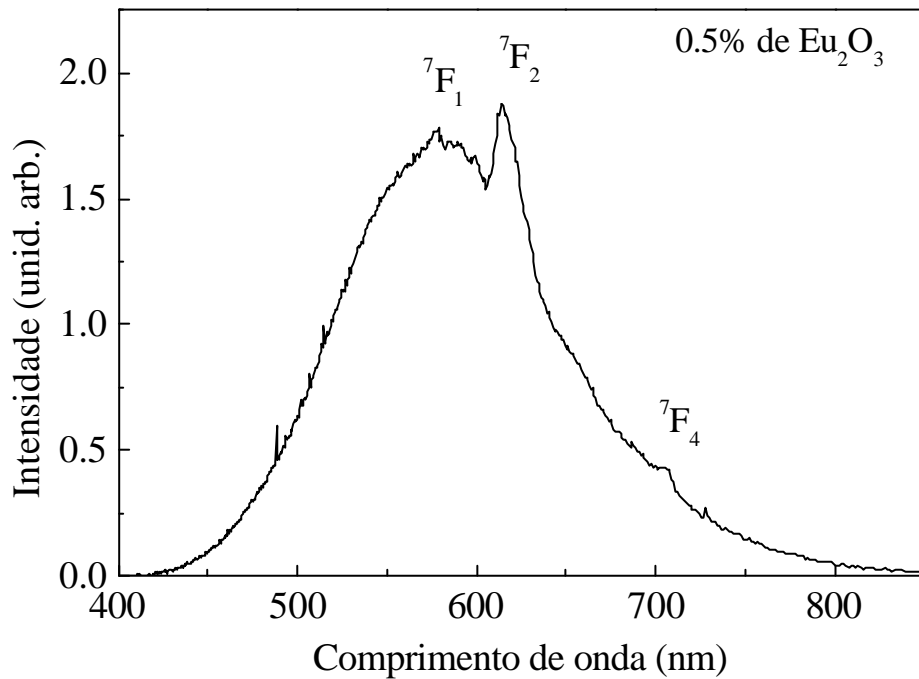
Figura 3.3 – Espectro de emissão do vidro LSCAS dopado com 0,5% de \text{Eu}_2\text{O}_3 .
