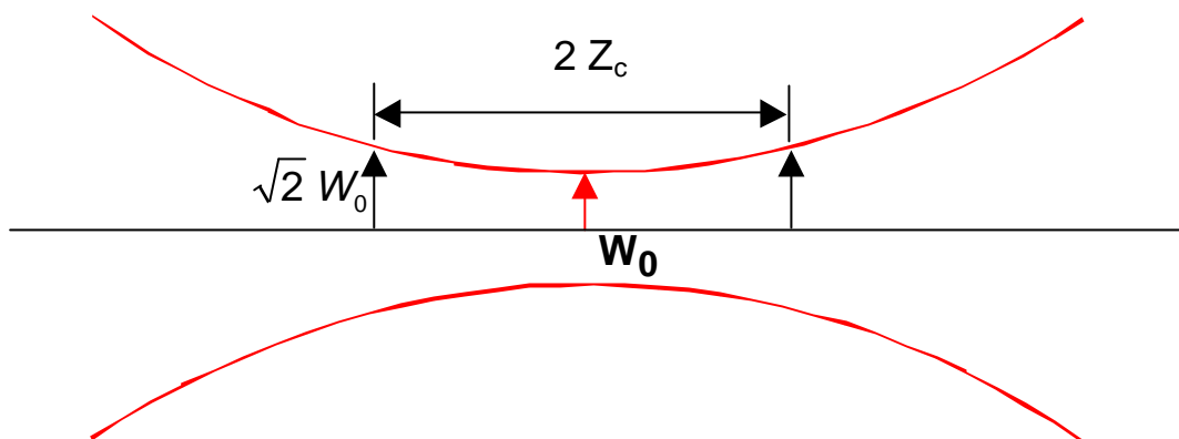
Figura 1.9- Parâmetro confocal em um feixe laser.
