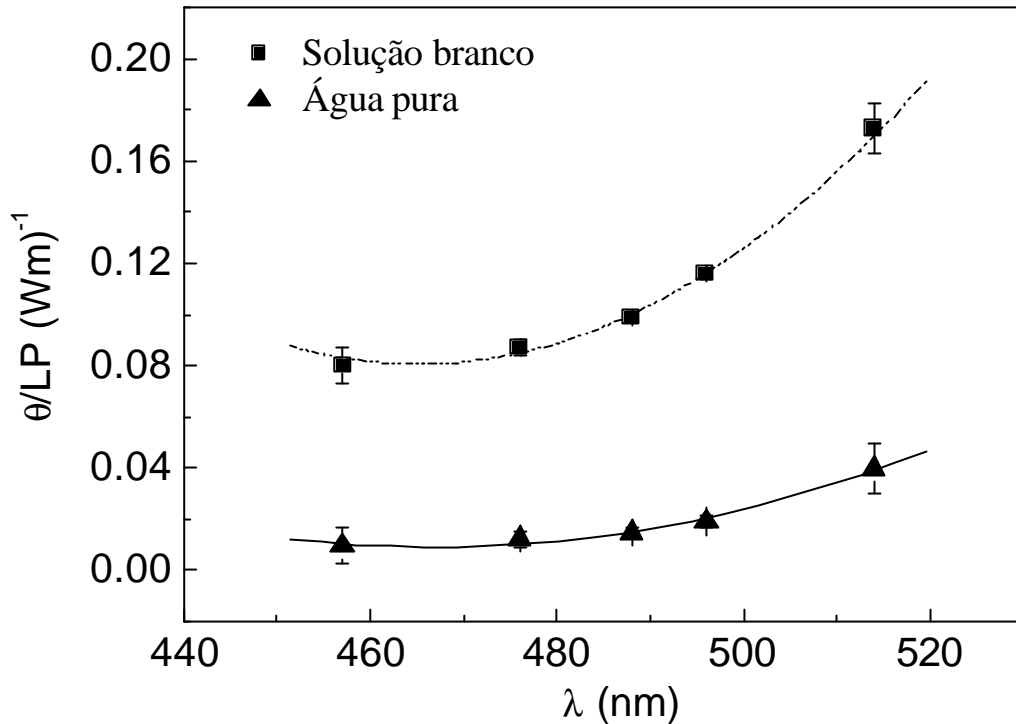
Figura 2.14 - Sinal de LT em função dos comprimentos de onda do laser de argônio. Os comprimentos de ondas das medidas foram \lambda = 457\text{nm} , 476\text{nm} , 488\text{nm} , 496\text{nm} e 514\text{nm} . Medidas realizadas na cubeta de 1cm utilizando a configuração otimizada.
