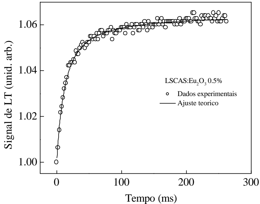
Figura 3.4 - Curva de TL para o vidro LSCAS dopado com 0.5% de \text{Eu}_2\text{O}_3 . Potência do feixe de excitação 16 mW e comprimento de onda de excitação 457.9 nm.
