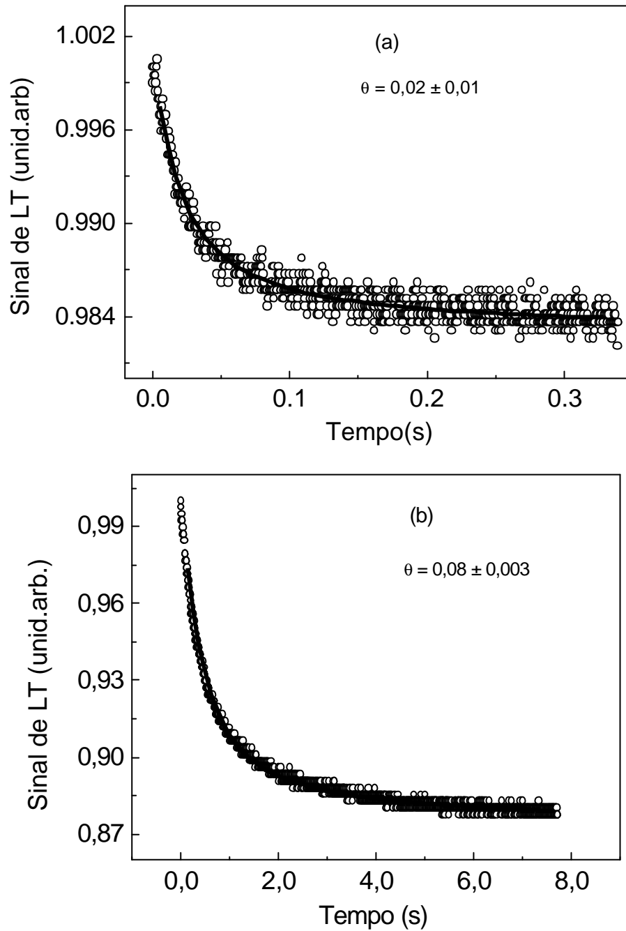
Figura 2.11 – Transientes de LT obtidos nas configurações (a) cruzada e (b) otimizada para a concentração de 10ppm na potência de 148mW. As espessuras das amostras nas configurações cruzada e otimizada foram L=0,2\text{cm} e L=1\text{cm} , respectivamente.
