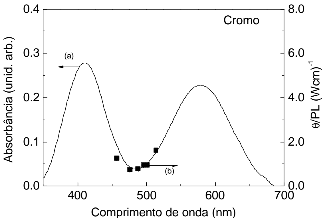
Figura 2.15 - (a) Espectro de absorbância da solução com 1000 ppm de cromo e (b) sinal \theta /PL em função do comprimento de onda da solução com 25 ppm de cromo.
