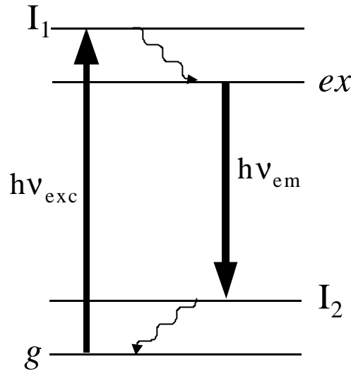
Figura 3.1 - Defeito quântico. Onde g é o estado fundamental, I_1 e I_2 estados intermediários e ex o estado excitado.
