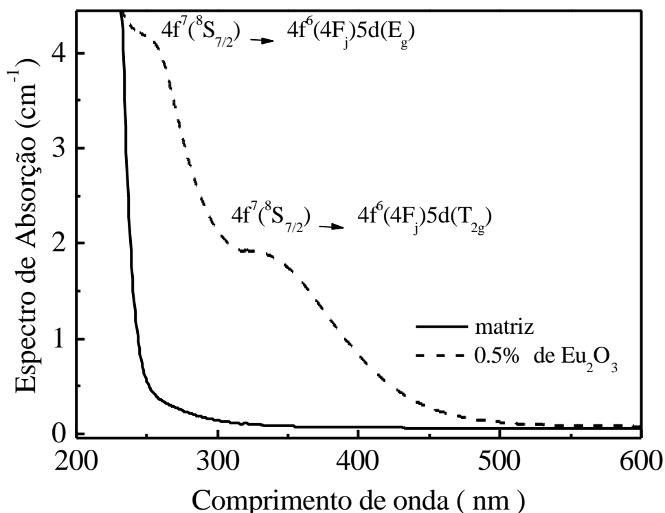
Figura 3.2 - Espectro de Absorção do vidro LSCAS não dopado e dopado com 0,5% de Eu_2O . As respectivas bandas atribuídas ao Eu^{3+} estão identificadas.
