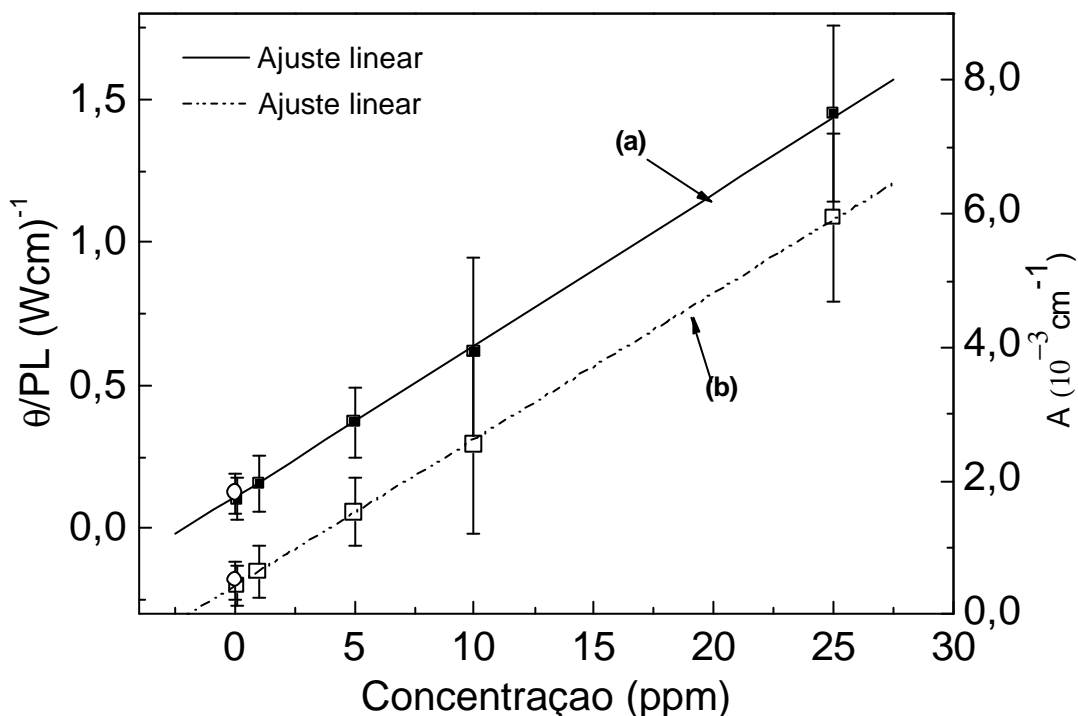
Figura 2.8 – (a) Amplitude do sinal de LT normalizada pela espessura da amostra e pela potência do feixe de excitação ( \theta/PL ) em função da concentração de cromo sob forma de cloreto para \lambda_e=514nm ; (b) coeficiente de absorção óptica ( A ) em função da concentração. O símbolo (o) representa os dados da solução branco. As medidas foram realizadas na configuração cruzada.
