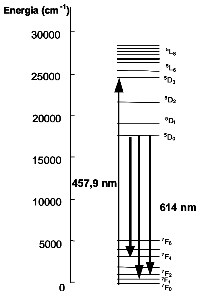
Figura 1.2 - Diagrama de níveis de energia do \text{Eu}^{3+} .
