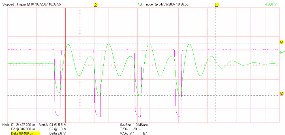
Fig. 4.4 - Ciclo completo de detecção.
