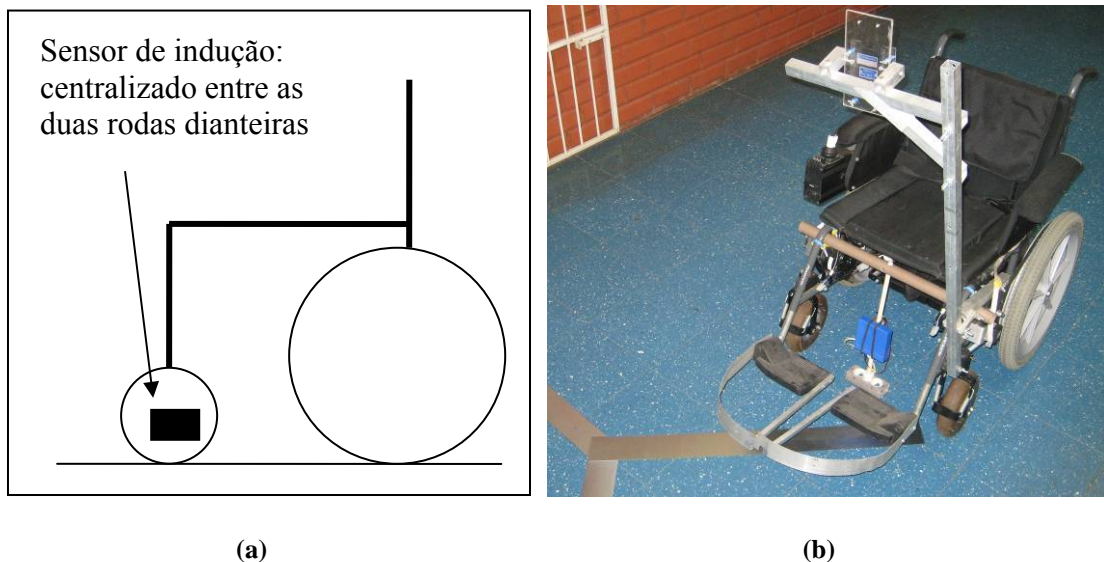
Fig. 6.1 - Posicionamento do sensor de indução na cadeira de rodas robótica.
