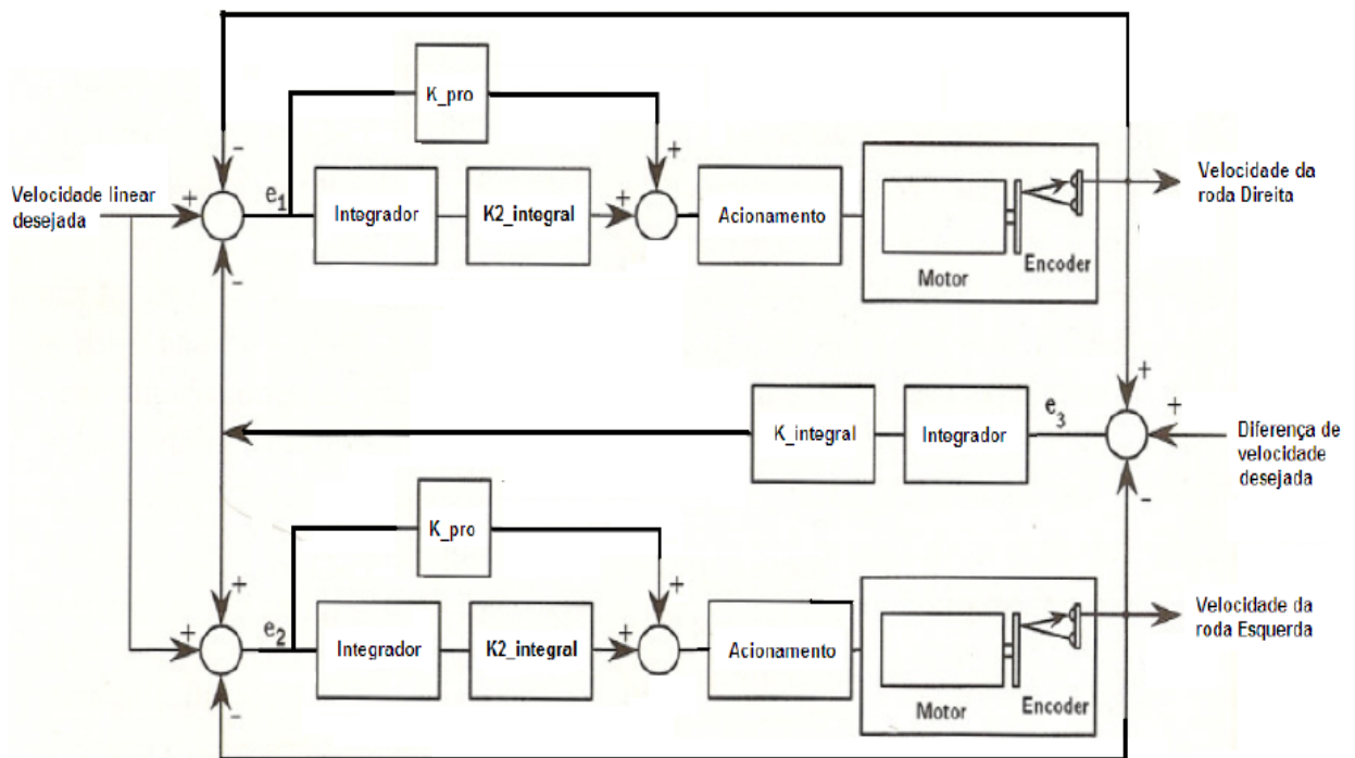
Fig. 3.5 – Diagrama de blocos do controlador PI utilizado no projeto. (Filgueira, 2007)
