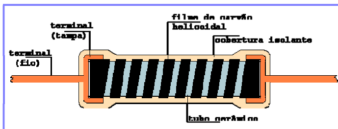
Figura 22 – Resistor de carbono e seus componentes
