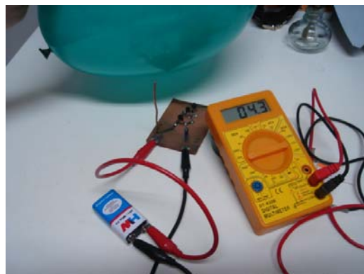
Fotografia 13 – Conexão do eletroscópio a bateria e o multímetro. Fonte: o autor (2006)
