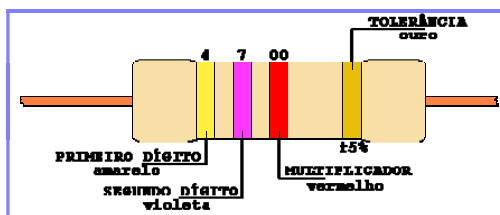
Figura 25 – Resistor identificado com o código de cores.
