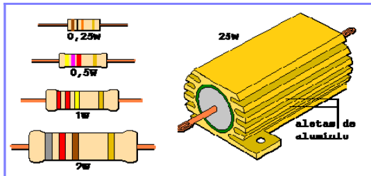
Figura 26 – Resistores classificados conforme potência.
