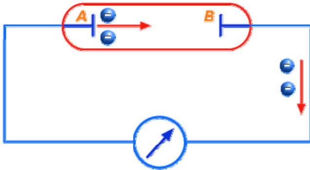
Figura 41 - Esquema de Edison do efeito termoiônico.
