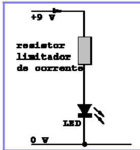
Figura 38 – Circuito: resistor e LED.
