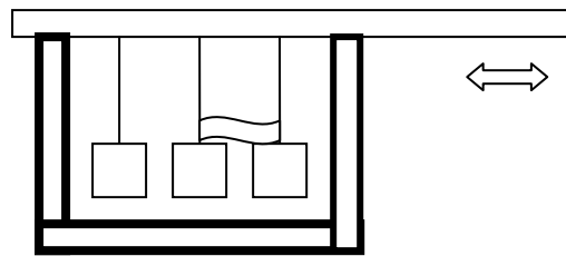
Figura 2 – Pêndulos Acoplados - visão completa do sistema. Fonte: o autor (2006).
