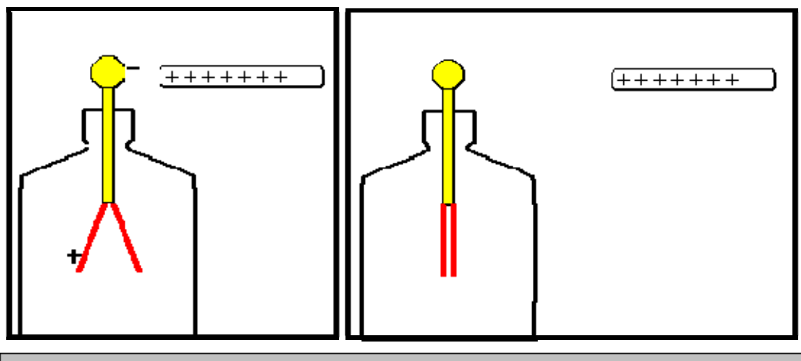
Figura 20 – Ilustração do fenômeno elétrico no eletroscópio de folhas.
