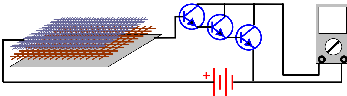
Figura 14 – Esquema de ligações entre a célula fotoelétrica e os demais componentes. Fonte: Revista Brasileira de Ensino de Física (2006).
