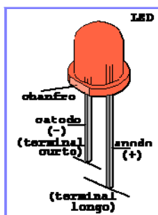
Figura 37 – Componentes do LED.
