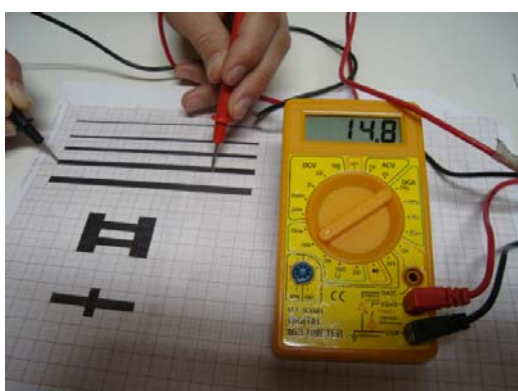
Fotografia 26 – Resistores de grafite. Fonte: o autor (2006)
