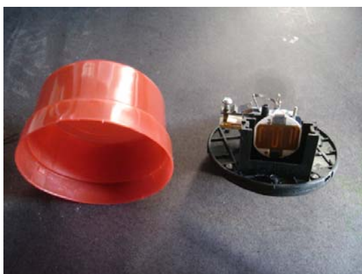
Fotografia 17 – Relé fotoelétrico aberto Fonte: o autor (2006).
