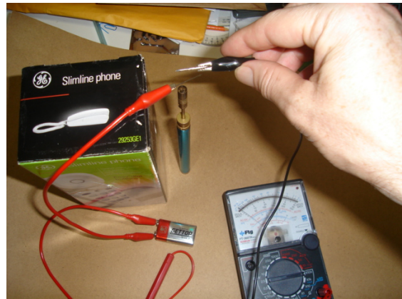
Fotografia 34 – Efeito termoiônico, componentes. Fonte: o autor (2006)
