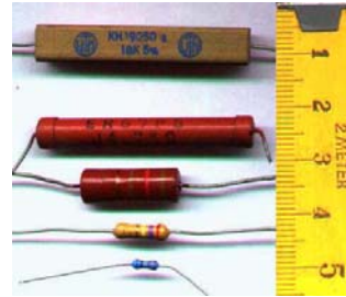
Figura 27 – Diferentes tamanhos de resistores.
