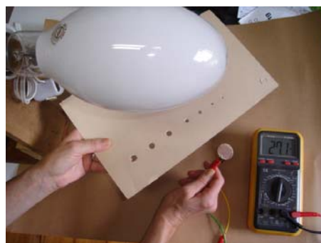
Fotografia 25 – Componentes para medição da resistência do LDR. Fonte: o autor (2006)
