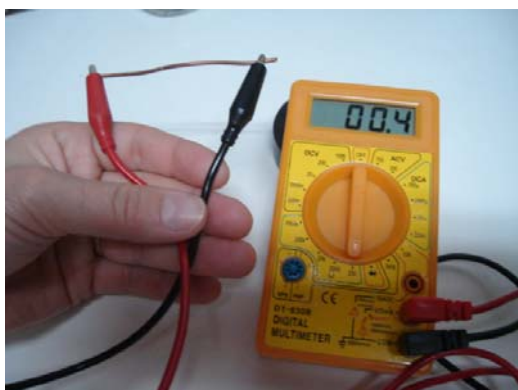
Fotografia 22 – Resistência elétrica do cobre a temperatura ambiente Fonte: o autor (2006)
