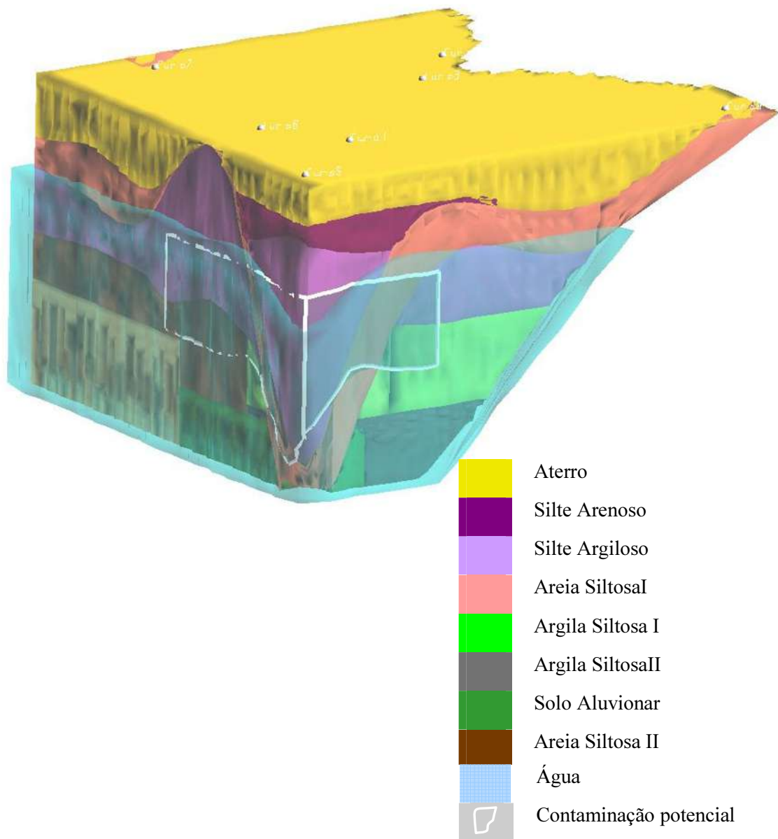
Figura 5.6 – Modelo tri-dimensional da estrutura geológica e contaminação (Araruna e outros, 2004)
