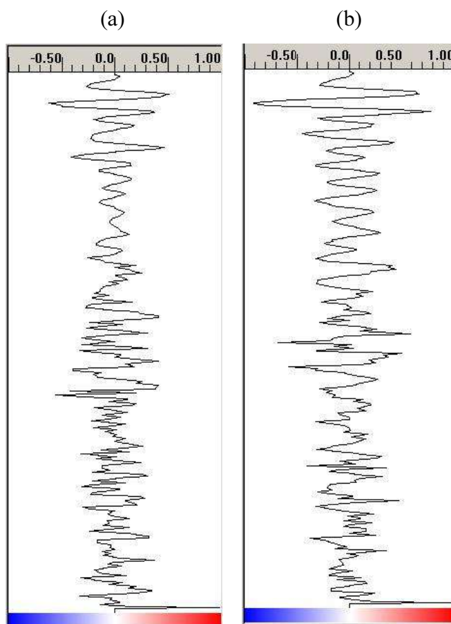
Figura 5.9 – Scans do perfil 1: (a) Região atenuada (b) Região não atenuada
