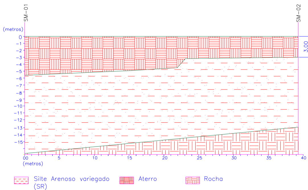
Figura 6.7 – Seção geológica na área do Parque Gráfico obtida com resultados de sondagem a percussão
