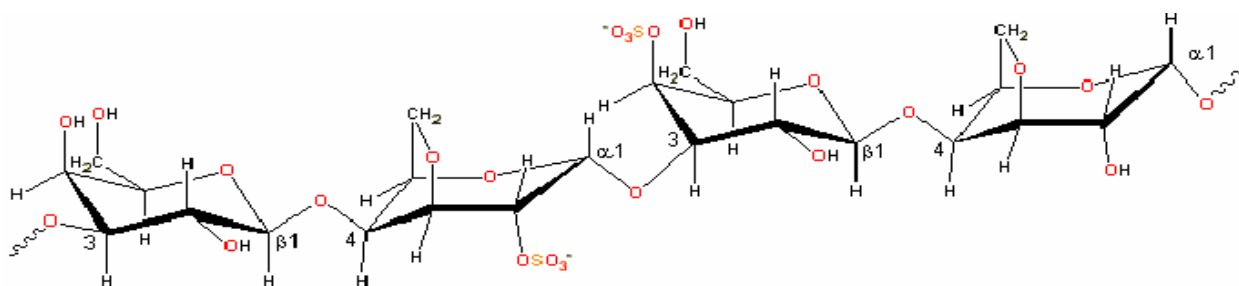
Figura 2.10 Estrutura química da \kappa -carragenana.
