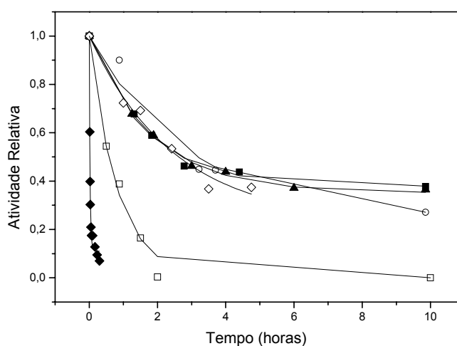
Figura 4.1 Inativação térmica de derivados ativados com glutaraldeído e com imobilização a pH 7,0 e 4^\circ\text{C} por 2h, com carga oferecida de 5 \text{mg enzima liofilizada} \cdot g^{-1} \text{gel} ( 55^\circ\text{C} e pH 8,0) de (◆) quimotripsina solúvel, (□) quitosana 2,5%; (◇) quitosana 5,0%; (○) quitosana 4,0%-gelatina 3,0%; (■) quitosana 2,5%-alginato 2,5%; (▲) quitosana 2,5%-carragenana 2,5%. As linhas indicam ajuste do modelo de inativação de Sadana-Henley aos pontos experimentais.
