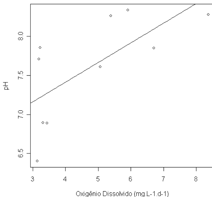
Figura 15- Variação do pH em relação à Concentração de Oxigênio Dissolvido ( P > 0,05 ). Apesar de possuírem relação não significativa, observou-se que sistemas que possuem maiores concentrações de OD apresentam pH mais elevados.
