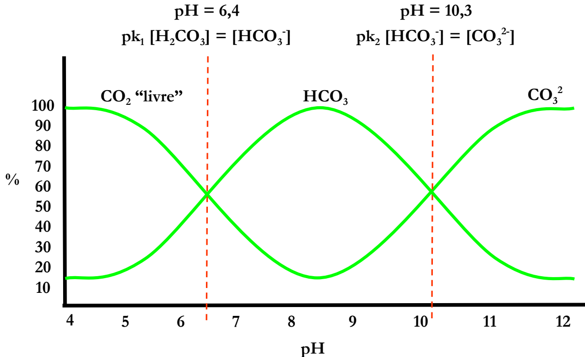
Figura 1- Relação entre pH e as proporções relativas das espécies de carbono inorgânico: CO 2 livre (CO 2 + H 2 CO 3 ), HCO 3 - e CO 3 2- na solução. O pK é o coeficiente de dissolução. No pH 6,4 o pK do ácido carbônico é igual a do bicarbonato significando que neste ponto as duas formas carbonatadas estão em equilíbrio no sistema. No pH 10,3 o pK do bicarbonato é igual a do carbonato significando que neste ponto ambas as formas carbonatadas estão presentes. (Retirado de Wetzel, 2001 e ligeiramente modificado de Golterman, 1969).
