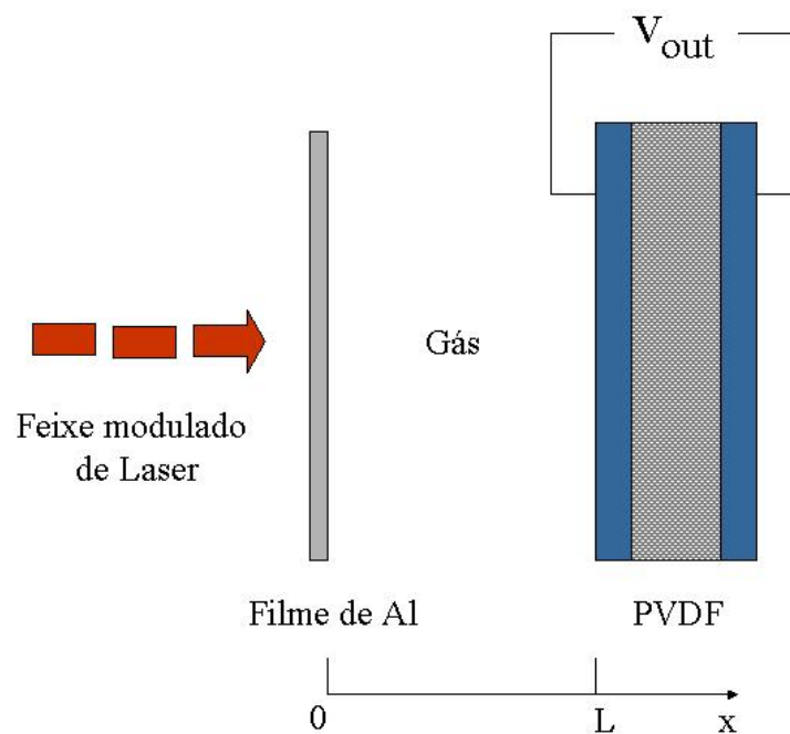
Figura 3.1: Esquema da cavidade para a interferometria de ondas térmicas.
