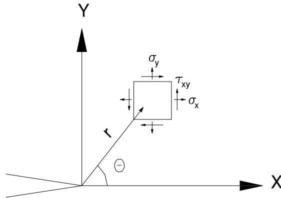
FIGURA 2.4 – Campo de Tensões na Ponta da Trinca
