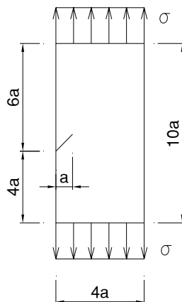
FIGURA 5.10 - Chapa retangular com trinca inclinada a 45^\circ na lateral
