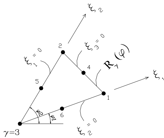
FIGURA 4.1 – Célula Triangular com Ponto Fonte no Vértice
