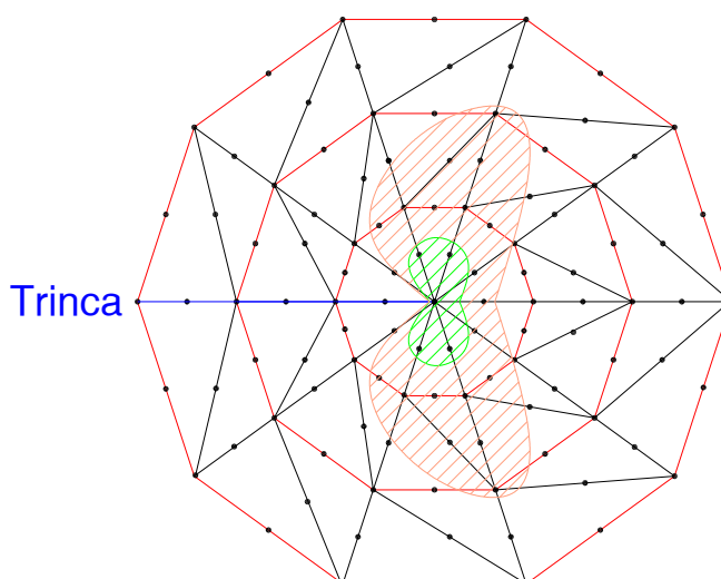
FIGURA 5.12 - Detalhe da Plastificação
