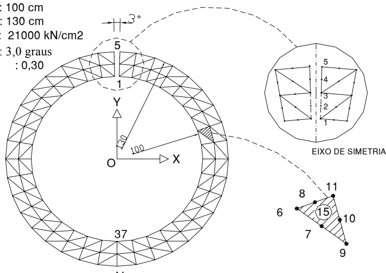
FIGURA 4.6 - Anel Circular com Tensão Inicial
