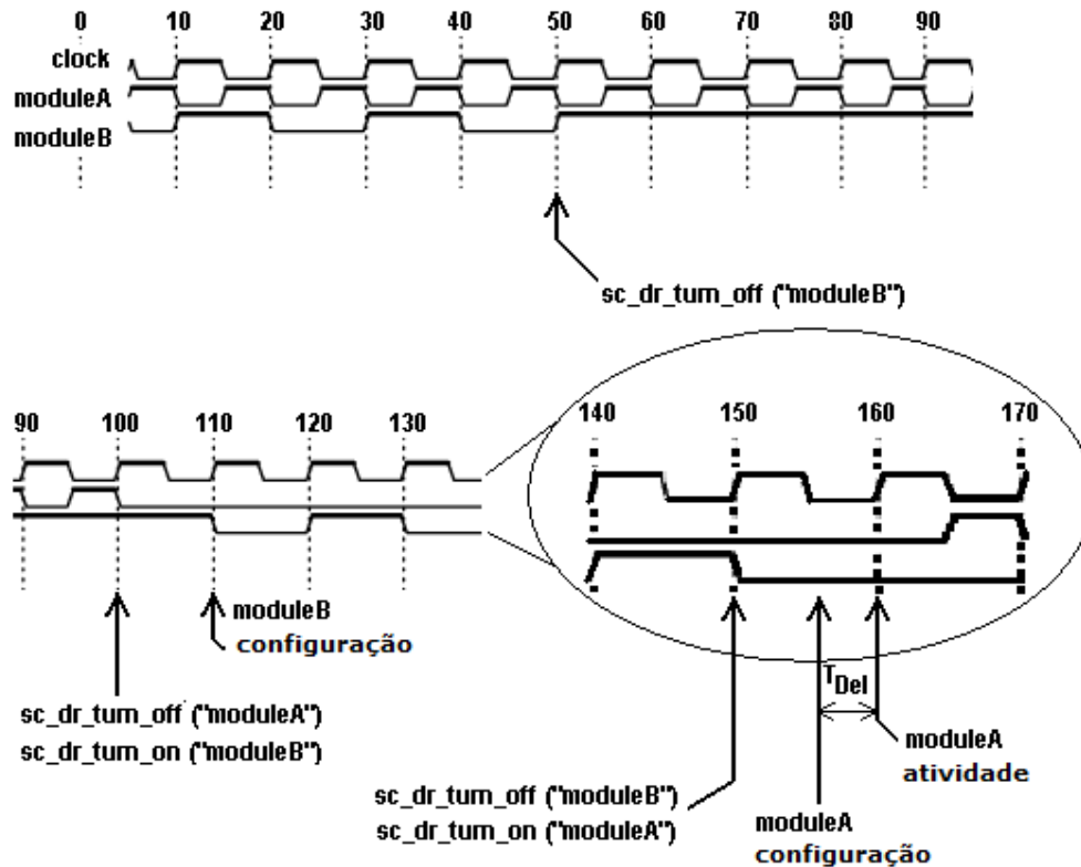
Figura 4-20: forma de onda do exemplo de prova do conceito.
