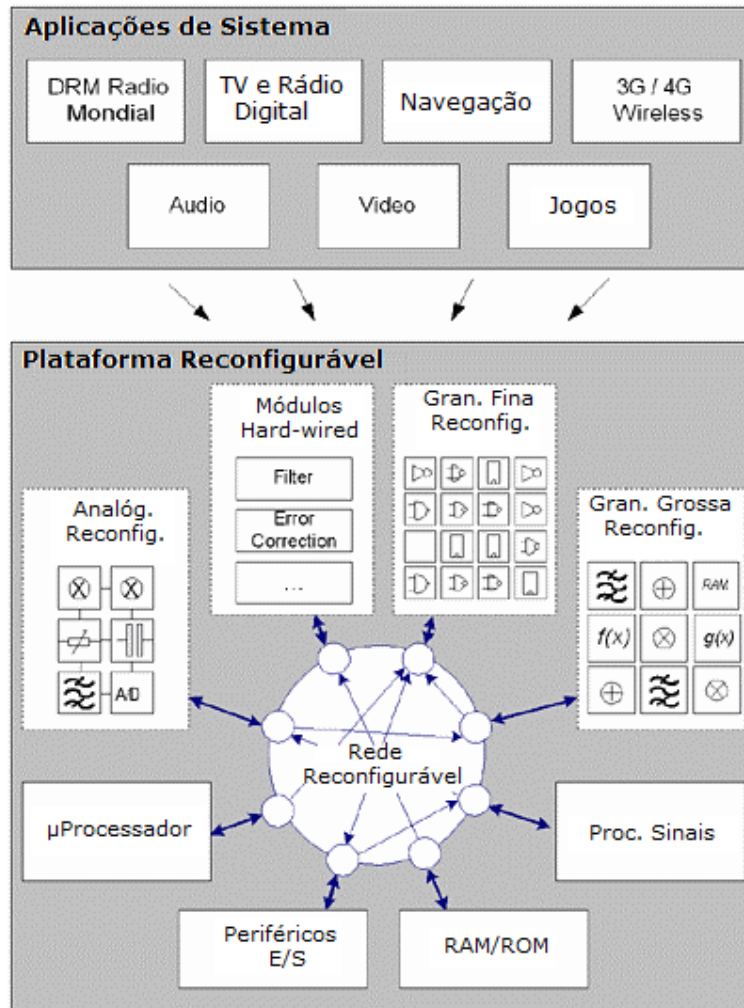
Figura 2-3: visão geral do projeto 4S
