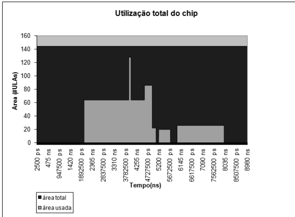
Figura 5-39: área total de chip utilizada no tempo
