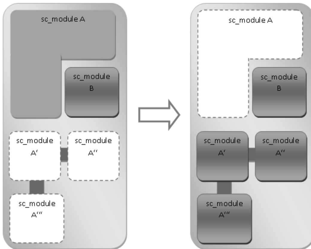
Figura 4-26: implementação do terceiro tipo de reconfiguração dinâmica.
