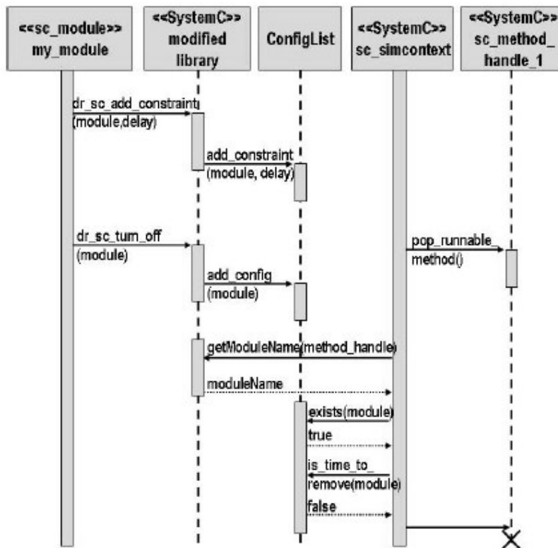
Figura 4-14: diagrama de seqüência que mostra passos para a desativação de um módulo.
