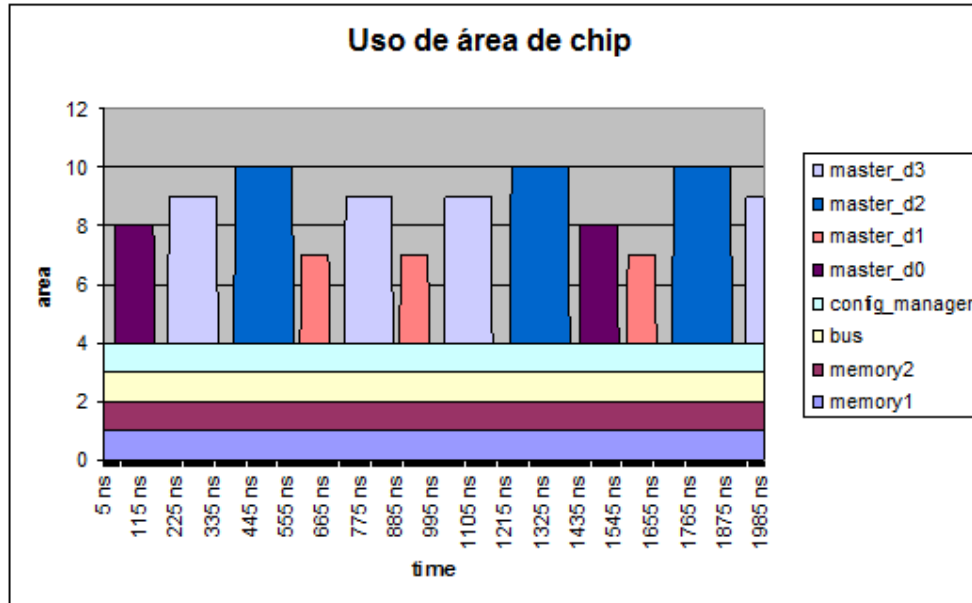
Figura 4-23: gráfico de uso de área de chip gerado a partir de uma tabela de histórico de execução.
