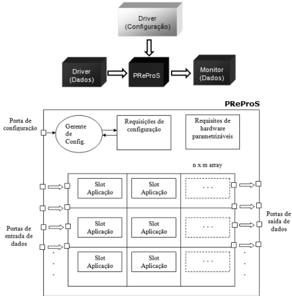
Figura 5-36: visão geral do PreProS
