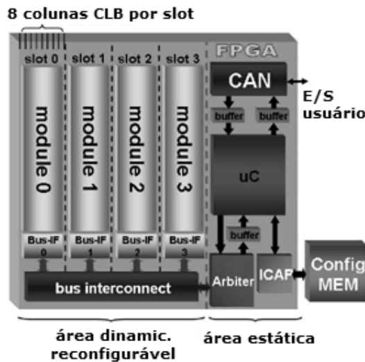
Figura 5-33: arquitetura da aplicação automotiva modelada.
