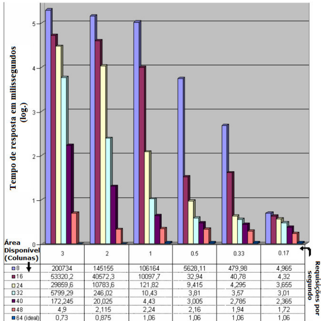
Figura 5-34: tempo de resposta do sistema em milissegundos para diferentes áreas reconfiguráveis disponíveis.
