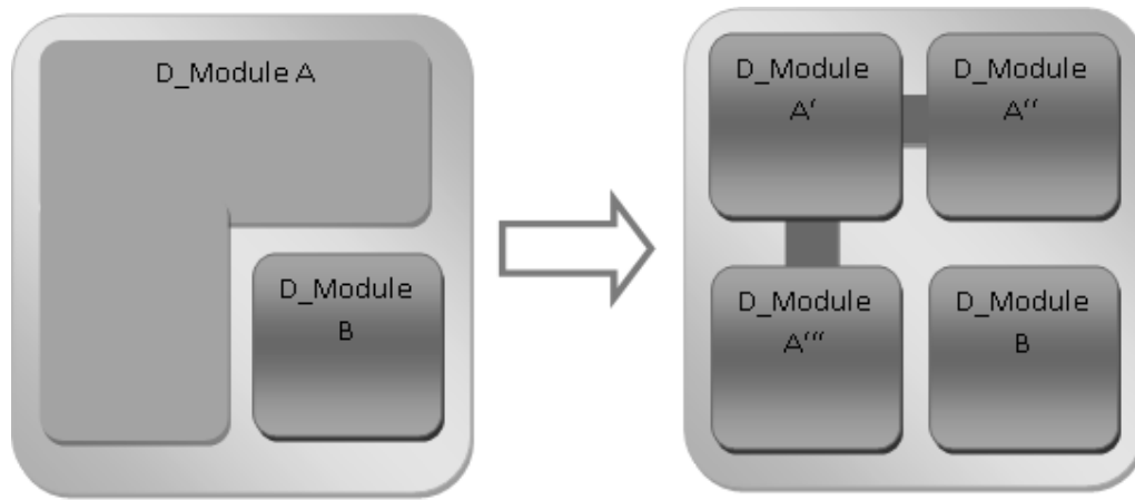
Figura 4-11: terceiro tipo de reconfiguração dinâmica. Particionamento de módulo configurável.
