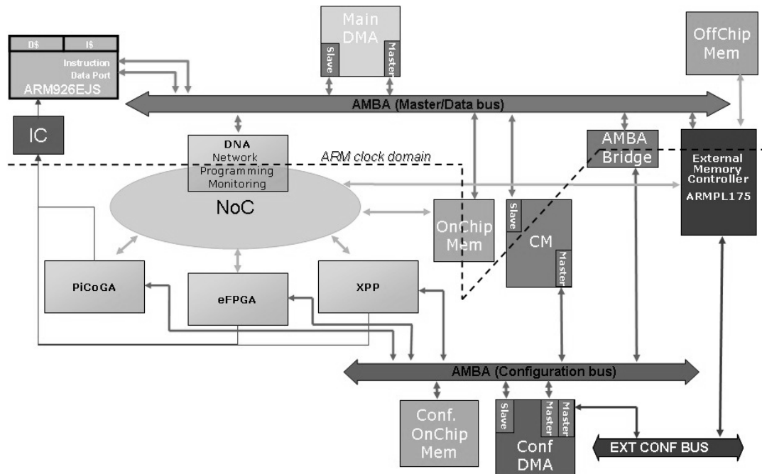
Figura 2-4: arquitetura da Plataforma MORPHEUS
