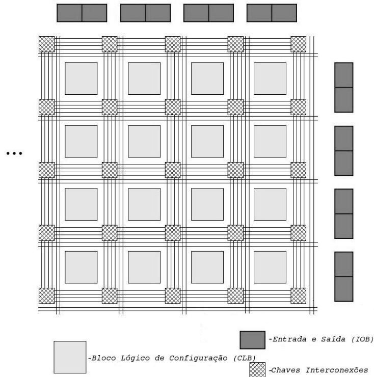
Figura 2-2: estrutura básica de um FPGA.
