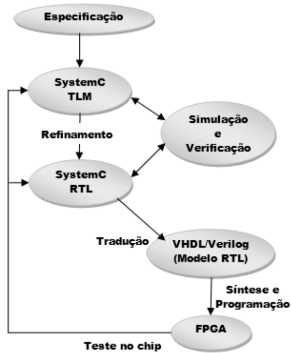
Figura 4-7: ciclo de projeto baseado em SystemC
