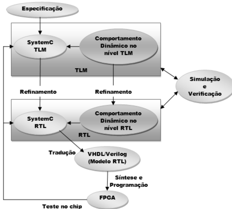
Figura 4-8: ciclo de projeto baseado em SystemC com suporte à reconfiguração dinâmica.
