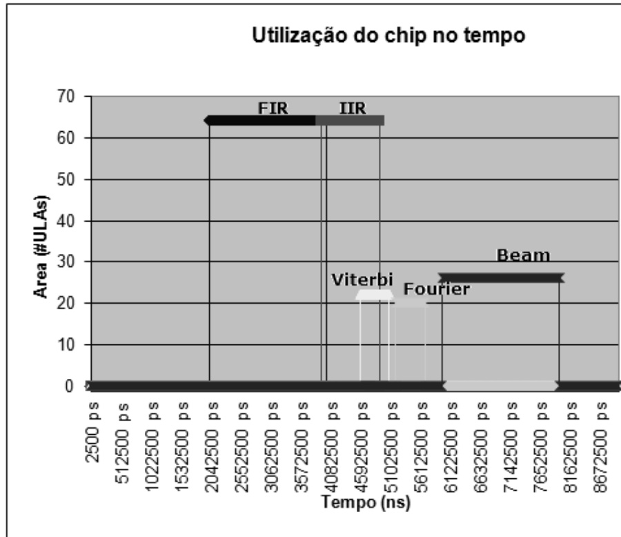
Figura 5-38: utilização de área por cada aplicação
