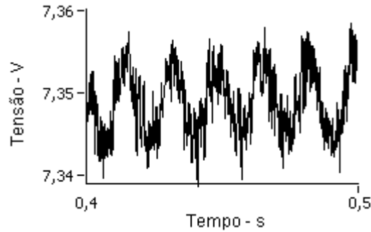
Figura 7 – Sinal de saída de um transmissor usado para medir a pressão de descarga do compressor
