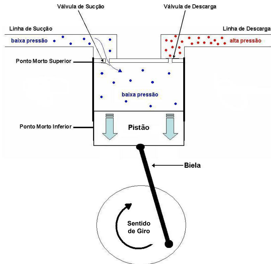
Figura 5 – Ciclo de sucção do compressor [19]
