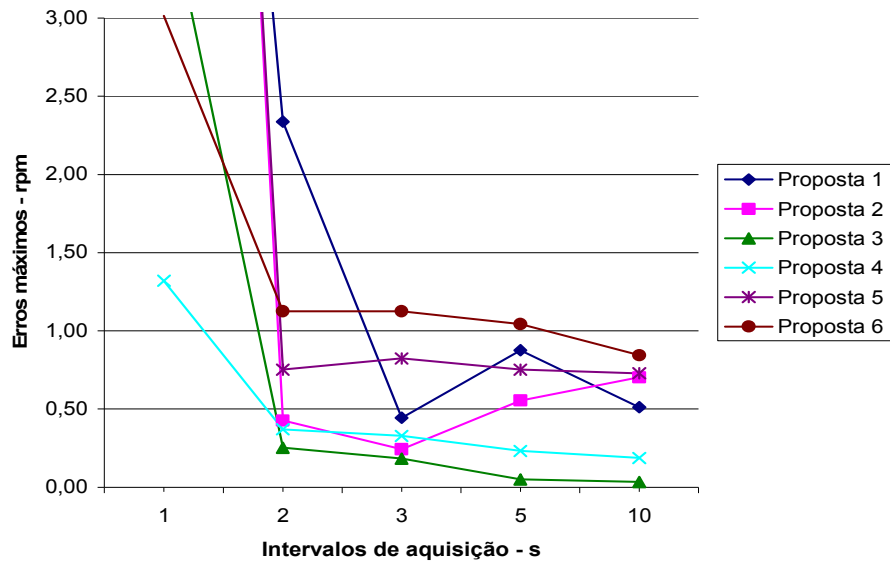
Figura 24 – Valores de erro máximo apresentados por métodos de medição baseados em detecção de componentes de excentricidade para diferentes intervalos de aquisição, em 59 Hz.
