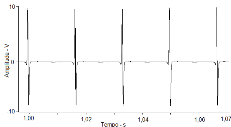
Figura 22 – Sinal de sincronismo
