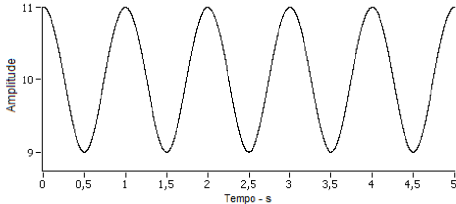
Figura 18 – Ilustração do comportamento do módulo B(t) para x(t)=10\text{sen}(2\pi 10t)+1\text{sen}(2\pi 11t)
