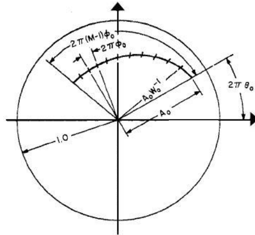
(a) Algoritmo de alocação de pontos no plano complexo pela CZT.
