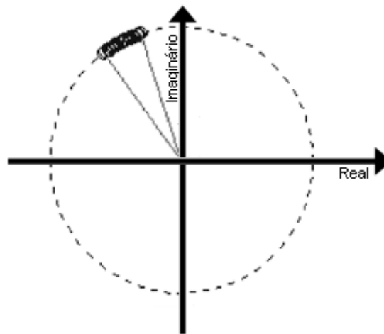
Figura 14 – A janela de freqüências da CZT [37]
