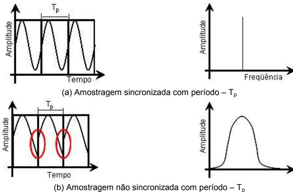
Figura 9 – Dispersão espectral inerente à transformada de Fourier
