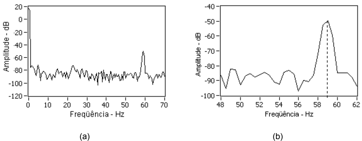
Figura 8 – Análise em frequência do sinal de pressão de descarga (a) de um compressor alimentado a 60 Hz. (b) Em visão ampliada.
