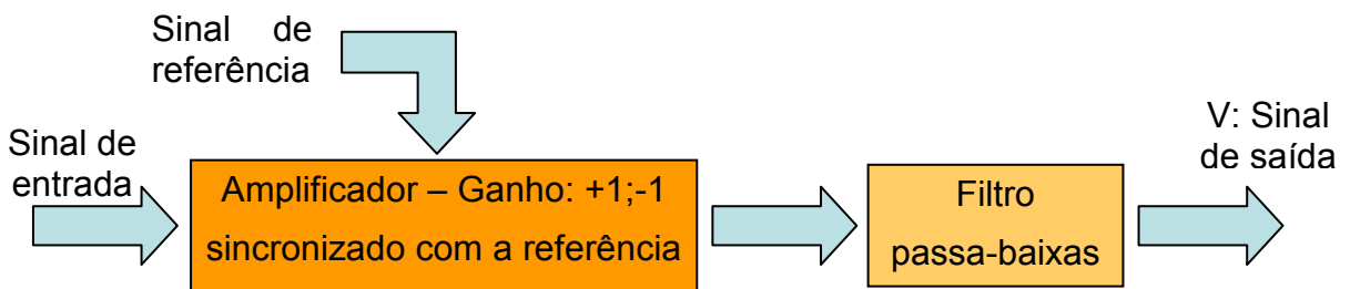
Figura 15 – Amplificador lock-in
