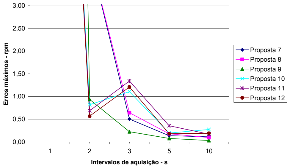
Figura 26 – Valores de erro máximo apresentados por métodos de medição baseados em detecção de frequência de escorregamento para diferentes intervalos de aquisição, em 59 Hz.
