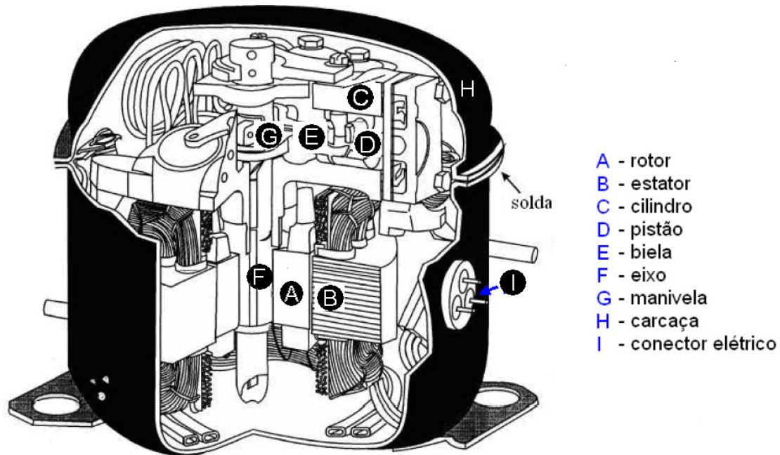
Figura 1 – Compressor hermético alternativo [8]
