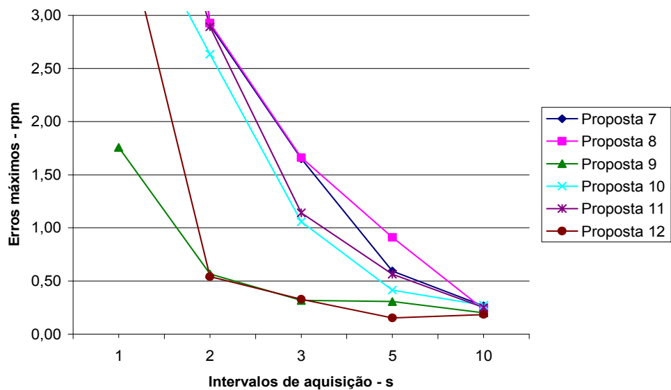
Figura 27 – Valores de erro máximo apresentados por métodos de medição baseados em detecção de frequência de escorregamento para diferentes intervalos de aquisição, em 58 Hz.
