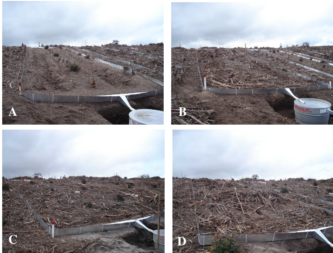
Figura 5. Aspecto gerais das parcelas; A - Subsolagem sem resíduo (SSR); B - Subsolagem interrompida (SIR); C - Coveamento mecanizado (CME); D - Subsolagem contínua com resíduo (SCR).
