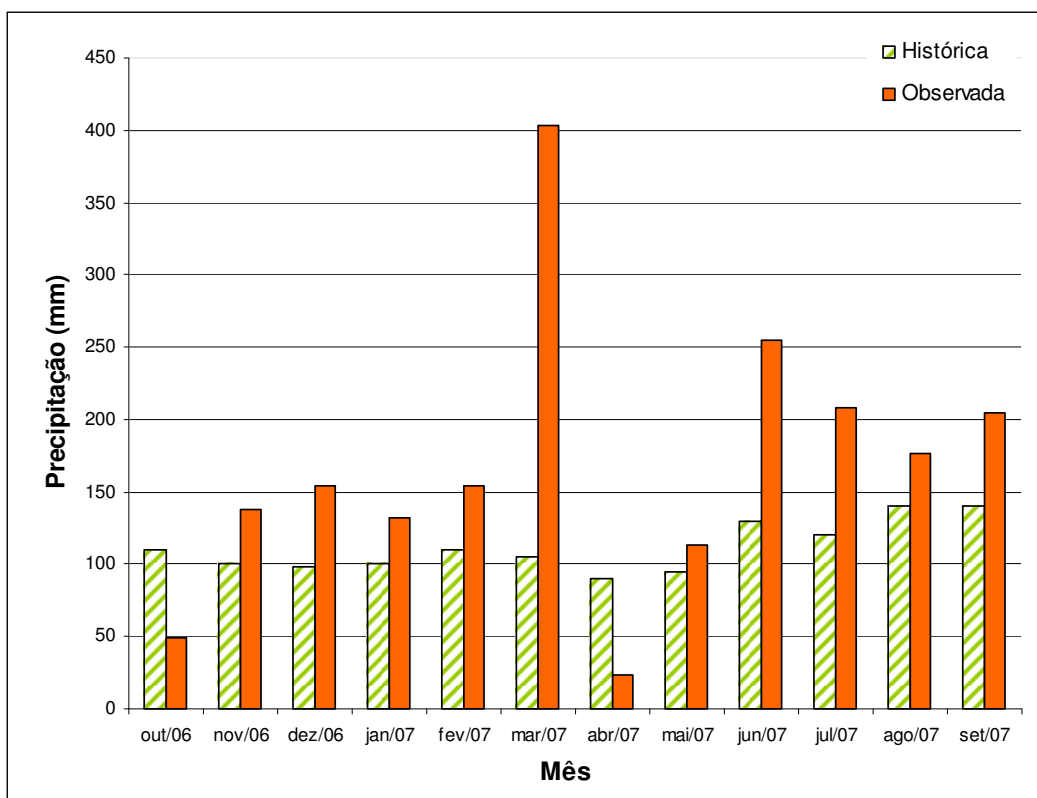
Figura 2. Precipitação mensal na área experimental durante o período de avaliação e precipitação histórica.
