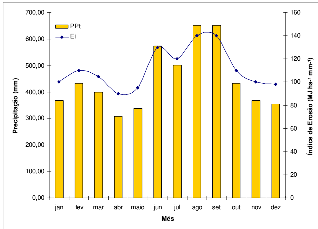
Figura 3. Índice de erosão médio mensal e precipitação mensal para o período de estudo na região de Arroio dos Ratos.
