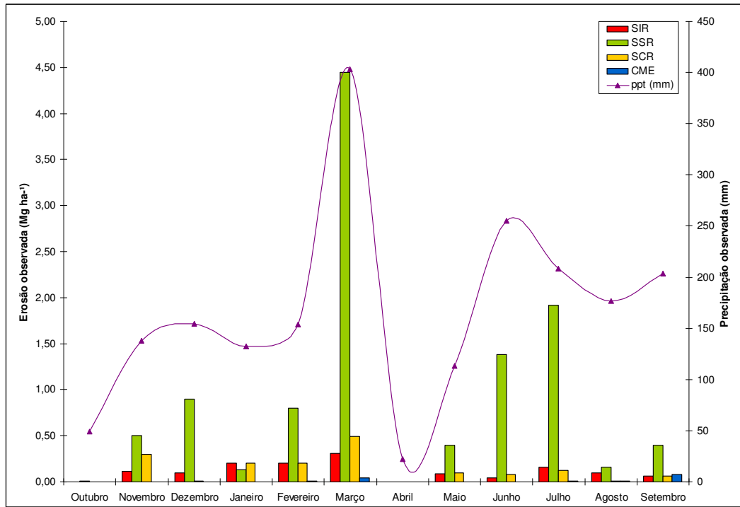
Figura 10. Erosão mensal observada dos eventos registrados.
