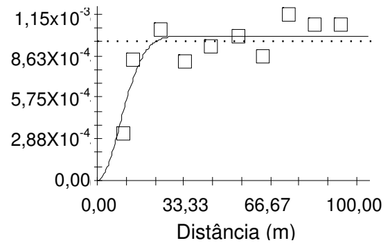
Figura 7. Semivariograma para velocidade de deslocamento (v)
