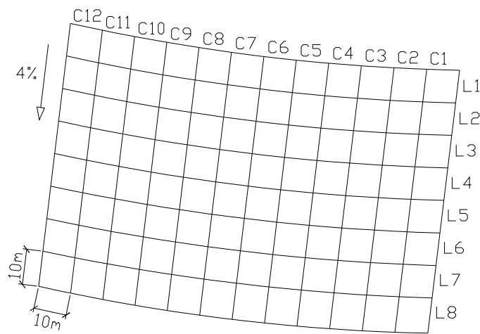
Figura 1. Croqui da área experimental
