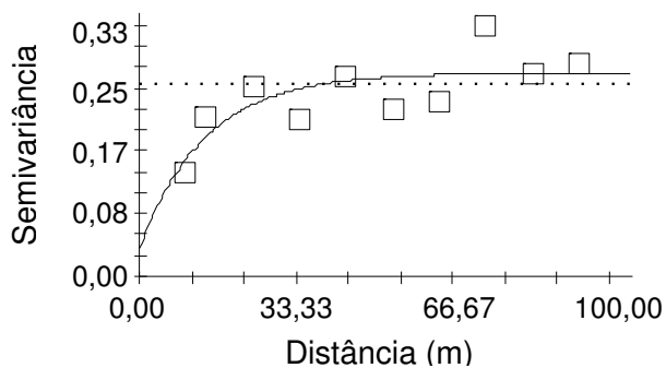
Figura 10. Semivariograma para consumo volumétrico ( C_{VOL} )
