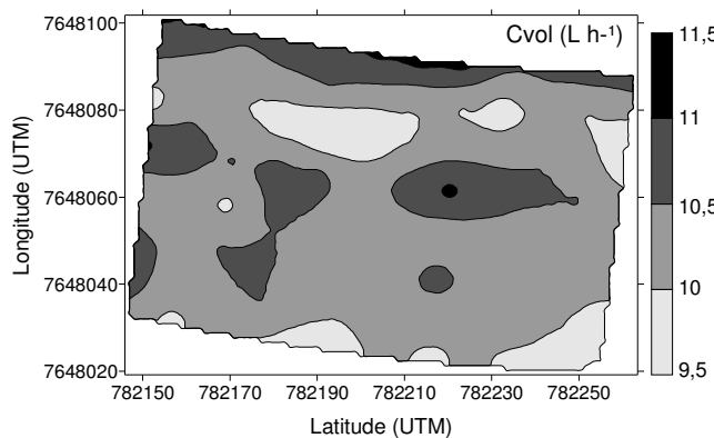
Figura 20. Mapa de isolinhas para consumo volumétrico (L h -1 )
