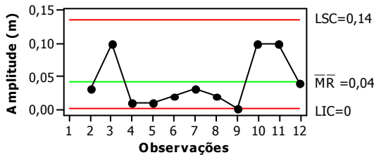
Figura 43. Carta de controle para espaçamento E9
