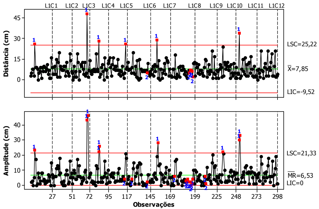
Figura 26. Carta de controle para distribuição longitudinal nas parcelas DL1
