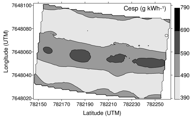
Figura 22. Mapa de isolinhas para consumo específico ( \text{g kWh}^{-1} )
