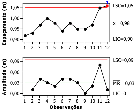
Figura 41. Carta de controle para espaçamento E7
