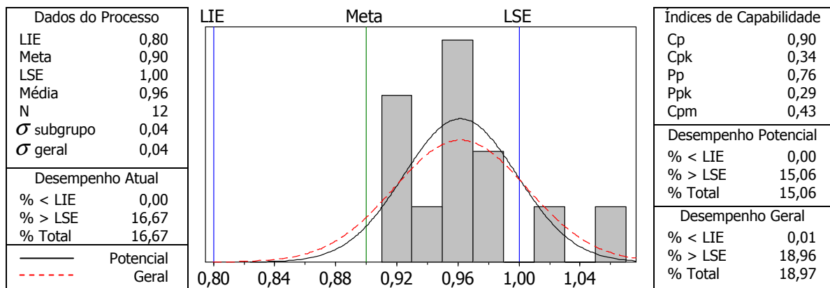
Figura 55. Análise de capacidade para espaçamento E9
