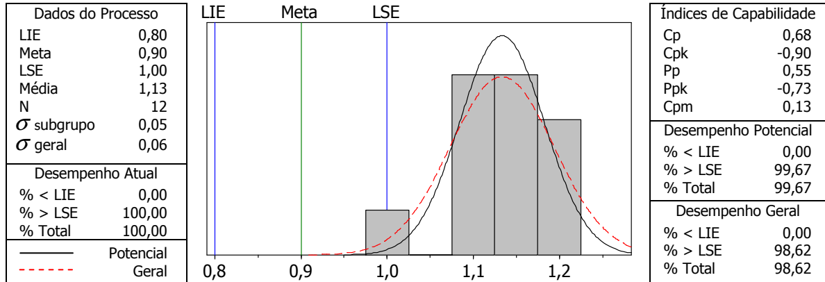
Figura 56. Análise de capacidade para espaçamento E10
