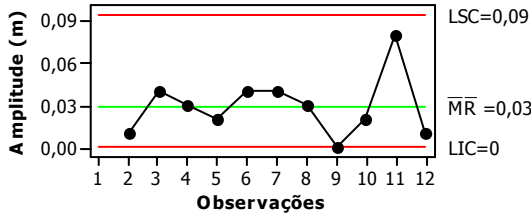
Figura 41. Carta de controle para espaçamento E7
