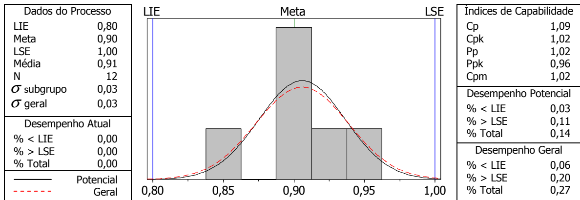
Figura 59. Análise de capacidade para espaçamento E14
