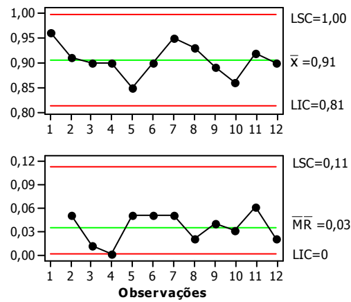
Figura 48. Carta de controle para espaçamento E14
