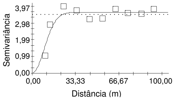
Figura 8. Semivariograma para potência na barra de tração (P)
