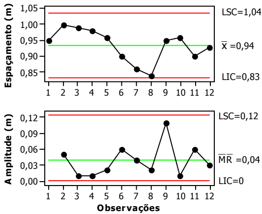
Figura 47. Carta de controle para espaçamento E13
