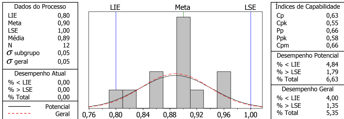
Figura 53. Análise de capacidade para espaçamento E4
