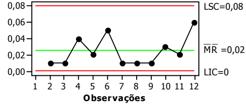
Figura 42. Carta de controle para espaçamento E8
