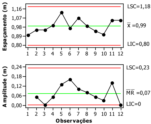
Figura 51. Carta de controle para espaçamento E17
