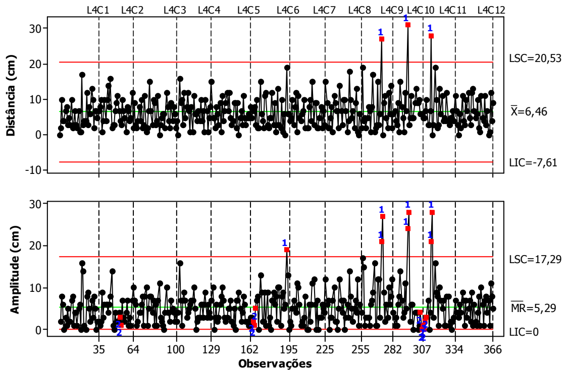
Figura 29. Carta de controle para distribuição longitudinal nas parcelas DL4
