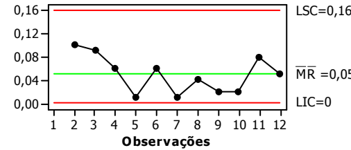
Figura 46. Carta de controle para espaçamento E12
