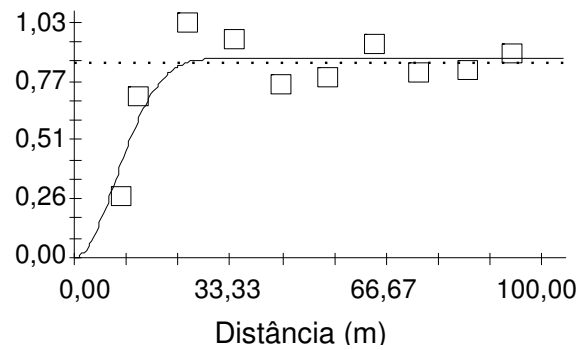
Figura 13. Semivariograma para consumo de energia ( C_e )
