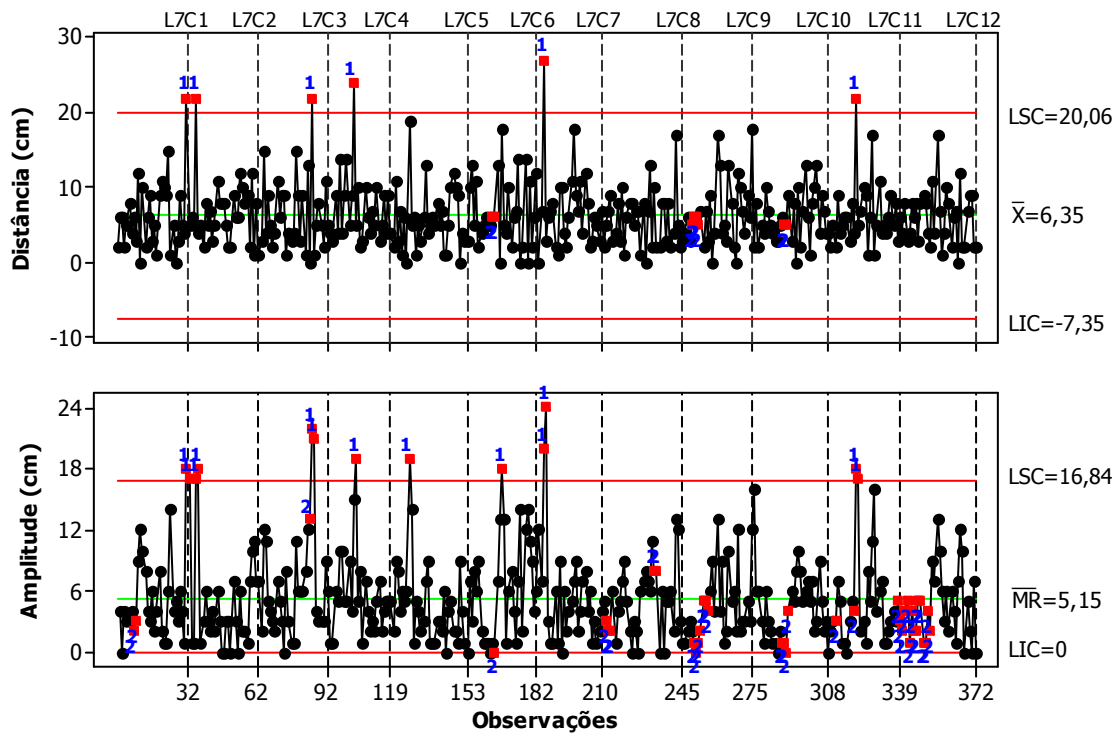
Figura 32. Carta de controle para distribuição longitudinal nas parcelas DL7
