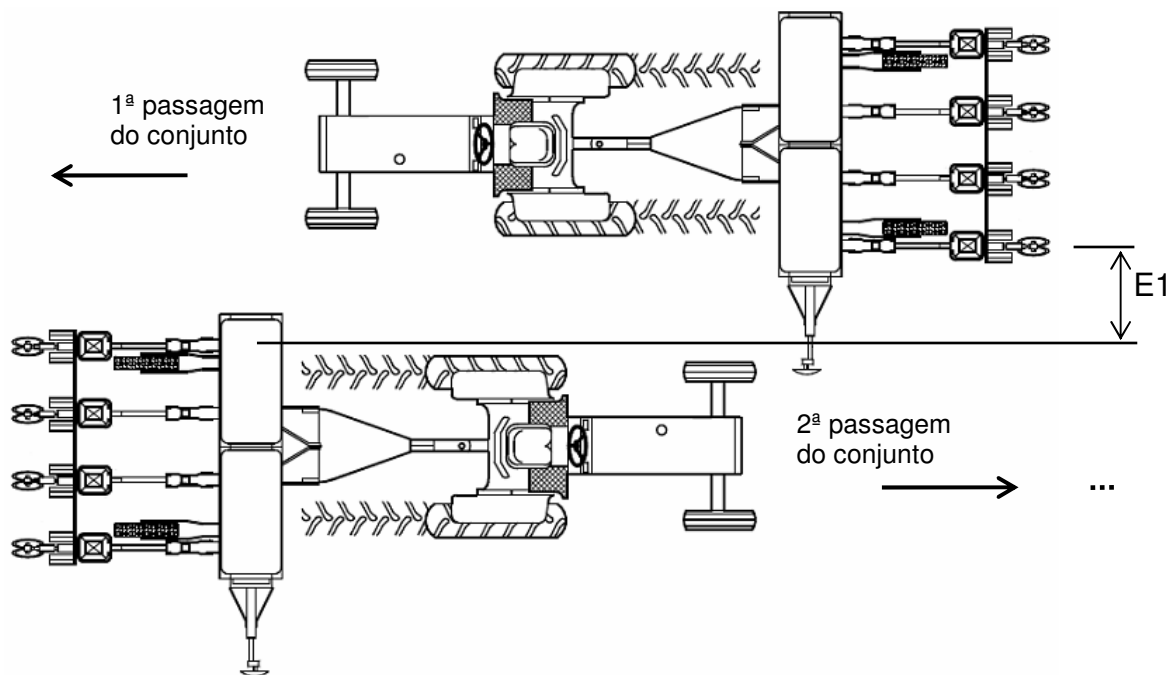
Figura 4. Esquema representativo das passagens do conjunto trator-semeadora
