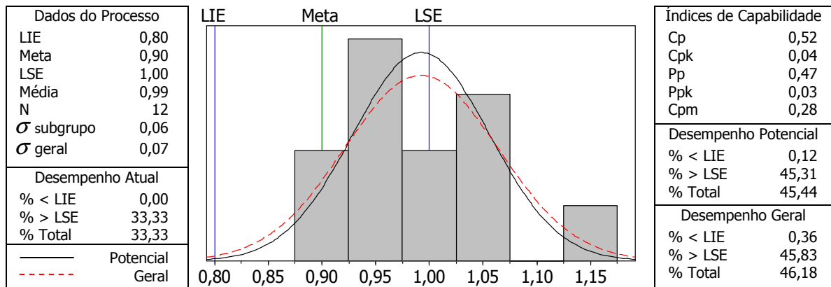
Figura 62. Análise de capacidade para espaçamento E17
