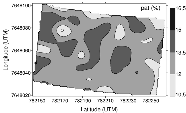
Figura 24. Mapa de isolinhas para patinação (%)
