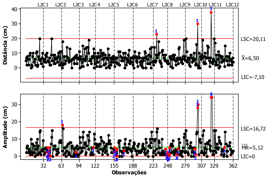
Figura 27. Carta de controle para distribuição longitudinal nas parcelas DL2
