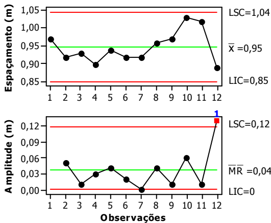
Figura 37. Carta de controle para espaçamento E3
