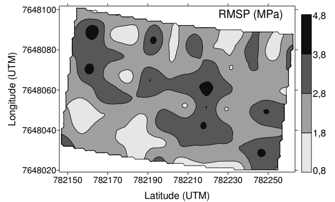
Figura 25. Mapa de isolinhas para RMSP (MPa)
