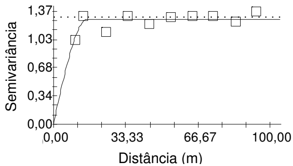
Figura 14. Semivariograma para patinação (pat)
