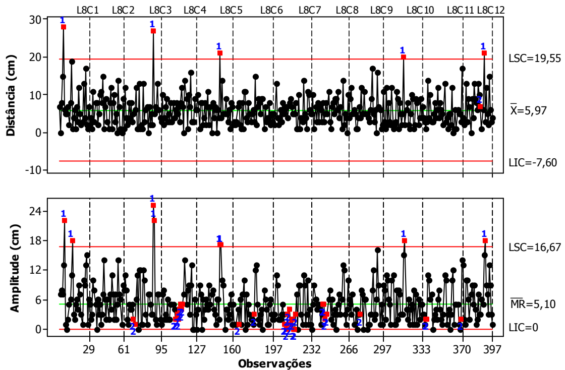
Figura 33. Carta de controle para distribuição longitudinal nas parcelas DL8
