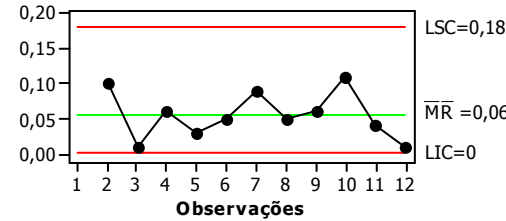
Figura 44. Carta de controle para espaçamento E10
