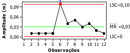
Figura 45. Carta de controle para espaçamento E11
