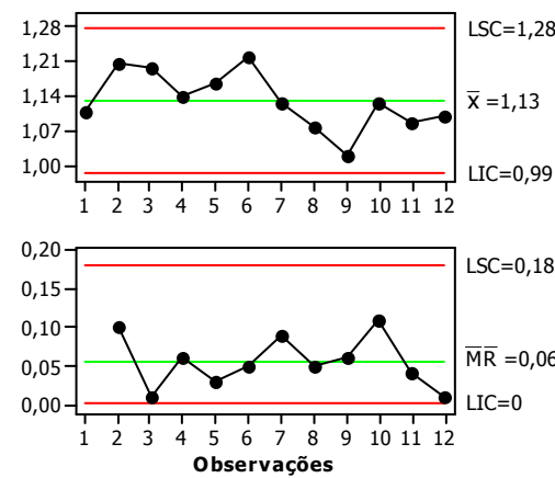
Figura 44. Carta de controle para espaçamento E10
