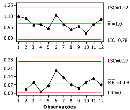
Figura 50. Carta de controle para espaçamento E16
