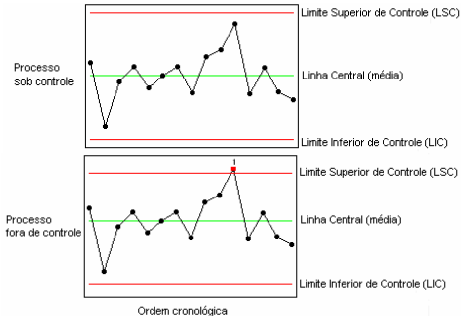
Figura 5. Estrutura das cartas de controle
