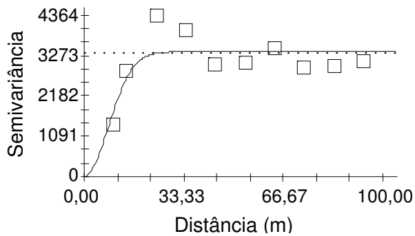
Figura 12. Semivariograma para consumo específico ( C_{ESP} )
