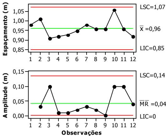
Figura 43. Carta de controle para espaçamento E9
