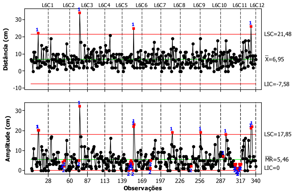
Figura 31. Carta de controle para distribuição longitudinal nas parcelas DL6
