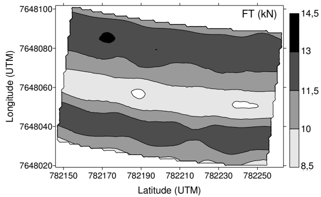
Figura 16. Mapa de isolinhas para força de tração (kN)
