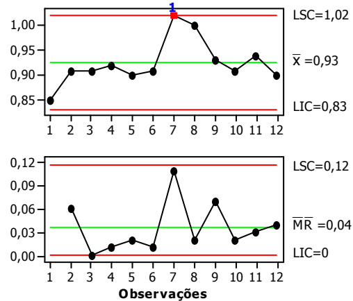
Figura 36. Carta de controle para espaçamento E2
