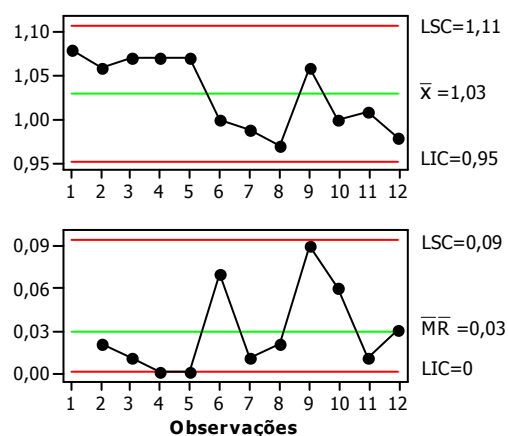
Figura 40. Carta de controle para espaçamento E6
