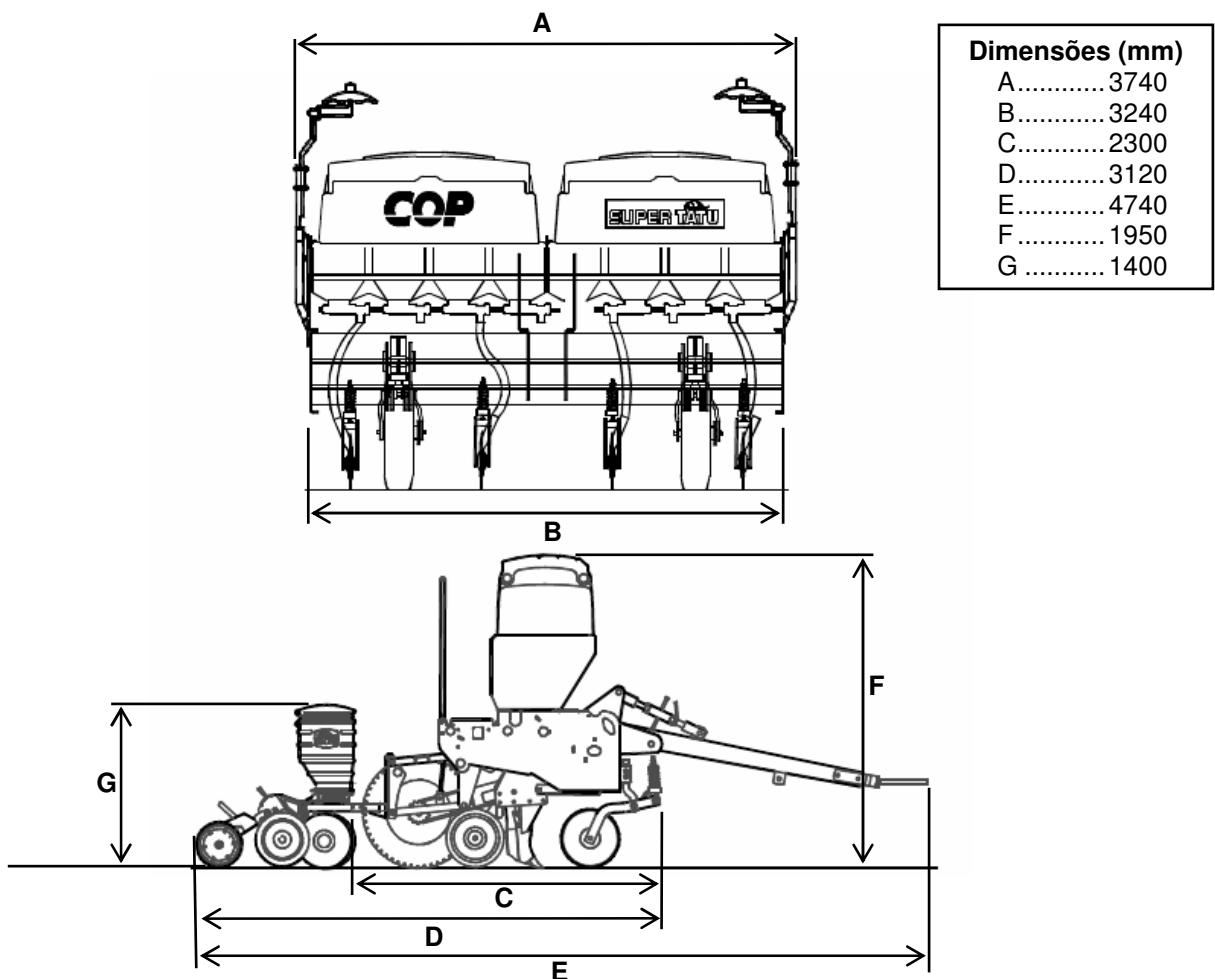
Figura 1A. Principais dimensões da semeadora-adubadora
