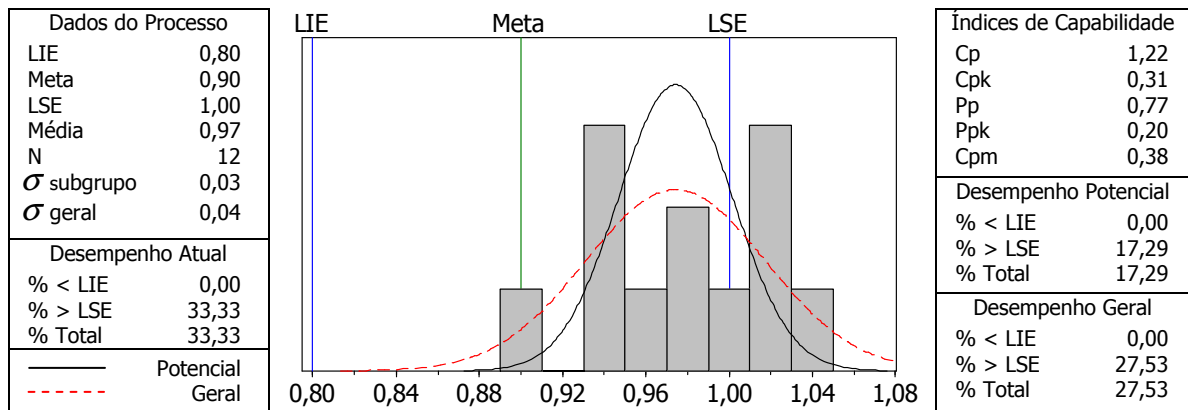
Figura 54. Análise de capacidade para espaçamento E5
