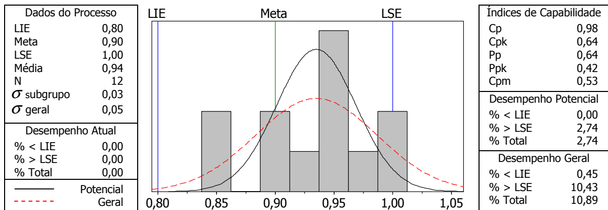
Figura 58. Análise de capacidade para espaçamento E13
