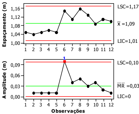
Figura 45. Carta de controle para espaçamento E11
