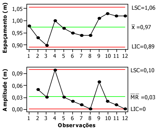
Figura 39. Carta de controle para espaçamento E5
