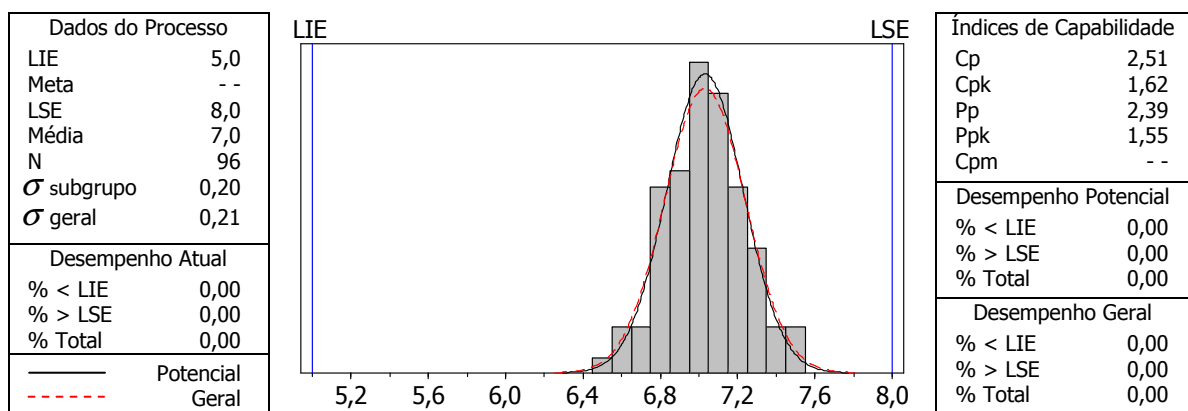
Figura 63. Análise de capacidade para número de dias para emergência (NDE)
