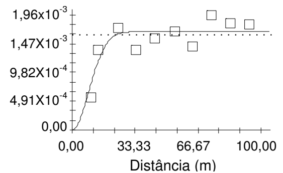
Figura 9. Semivariograma para capacidade de campo efetiva (CCe)
