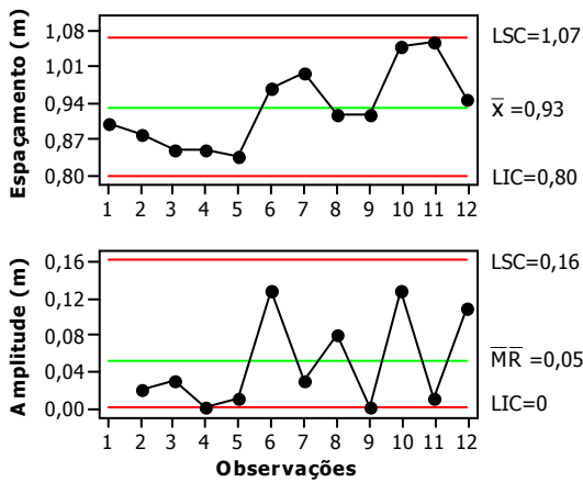
Figura 49. Carta de controle para espaçamento E15
