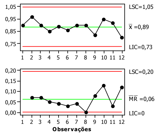
Figura 38. Carta de controle para espaçamento E4
