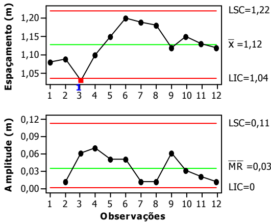
Figura 35. Carta de controle para espaçamento E1
