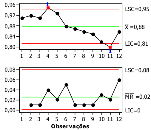
Figura 42. Carta de controle para espaçamento E8
