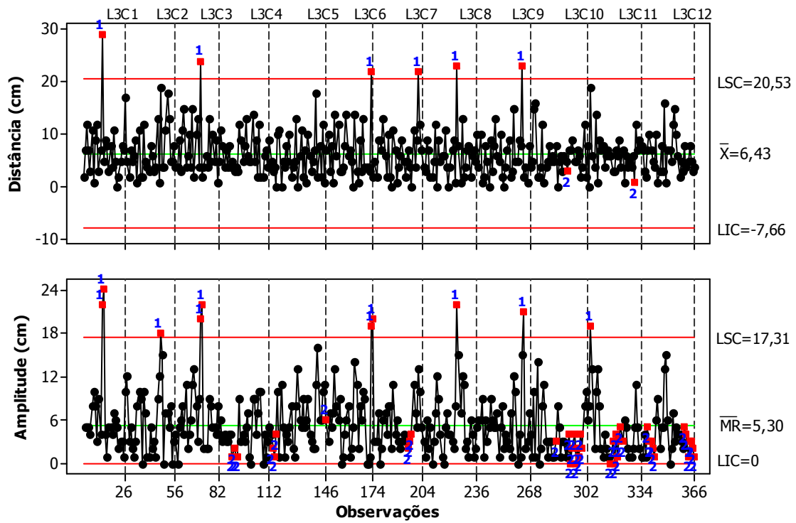
Figura 28. Carta de controle para distribuição longitudinal nas parcelas DL3
