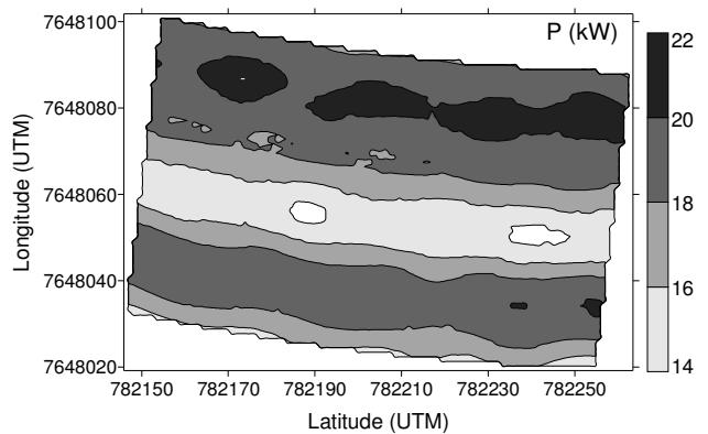
Figura 18. Mapa de isolinhas para potência na barra de tração (kW)
