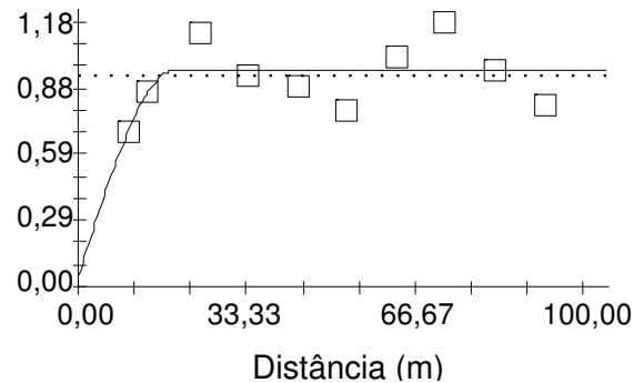
Figura 15. Semivariograma para resistência mecânica do solo à penetração (RMSP)
