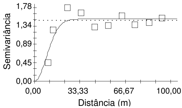
Figura 6. Semivariograma para força de tração (FT)
