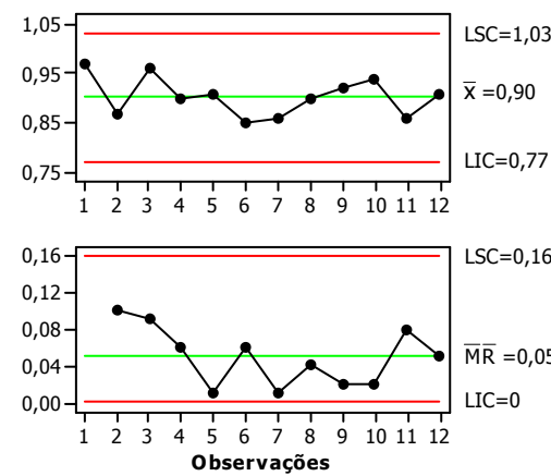
Figura 46. Carta de controle para espaçamento E12
