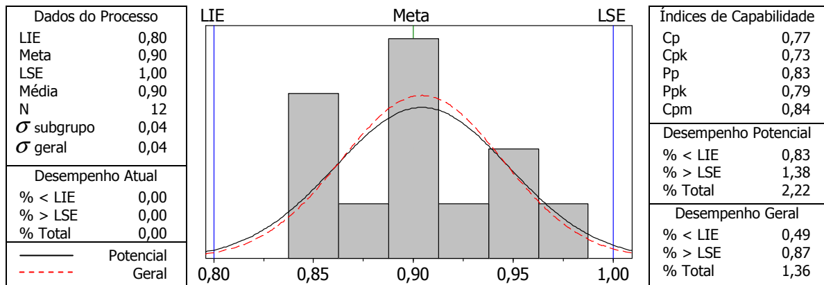
Figura 57. Análise de capacidade para espaçamento E12
