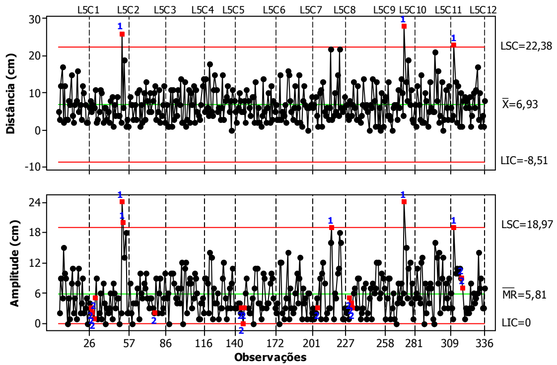
Figura 30. Carta de controle para distribuição longitudinal nas parcelas DL5
