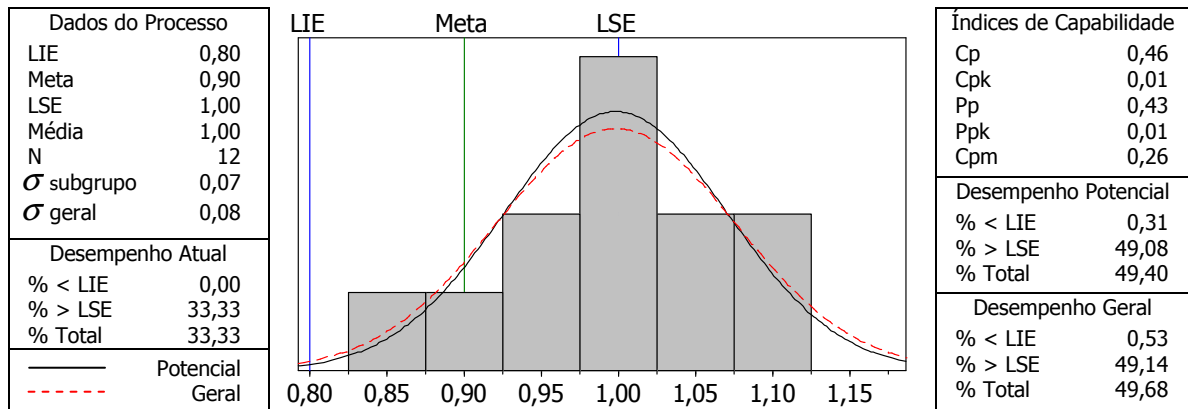
Figura 61. Análise de capacidade para espaçamento E16
