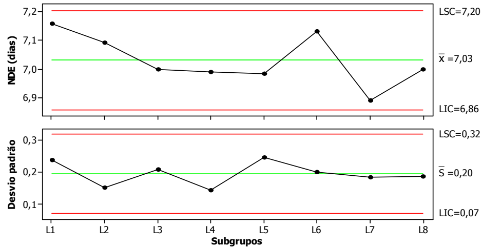
Figura 52. Carta de controle para número de dias para emergência (NDE)
