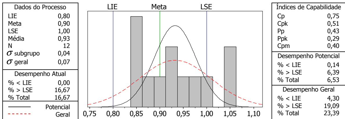
Figura 60. Análise de capacidade para espaçamento E15
