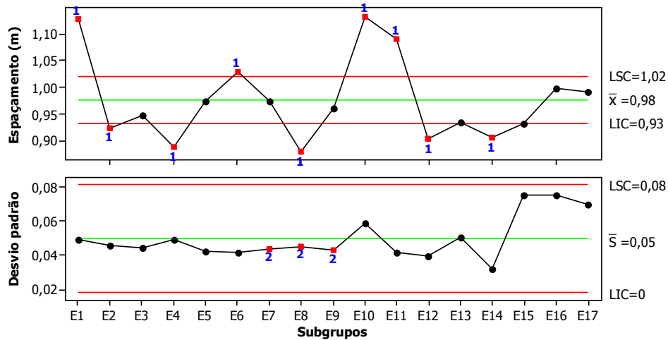
Figura 34. Carta de controle para espaçamento entre fileiras (E)
