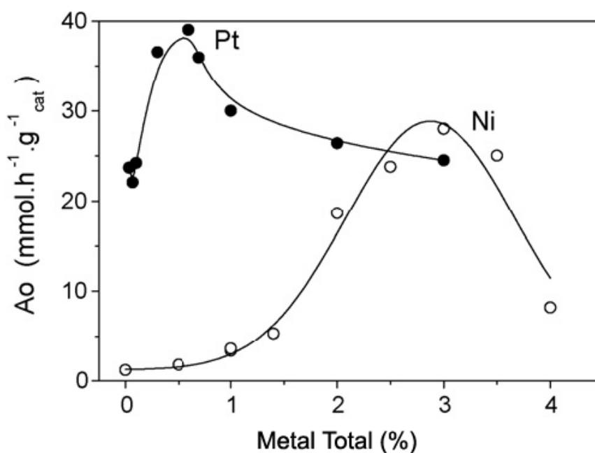
Figura 2.24. Atividade inicial (Ao) em função do teor de metal nos catalisadores Ni/HUSY e Pt/HUSY. [81].
