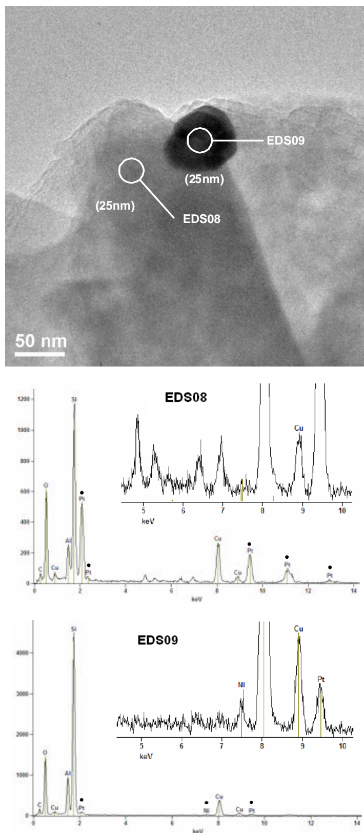
Figura 4.26. Micrografia do catalisador bimetálico 50Pt50Ni com 130 \mu\text{mol M/g}_{\text{cat}} utilizando a ativação rápida a 450^\circ\text{C} e magnificação de 50.000X e seus respectivos EDS.
