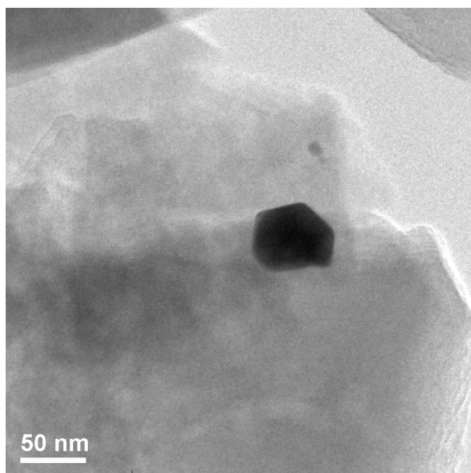
Figura 4.29. Micrografia do catalisador bimetálico 50Pt50Ni com 130 \mu\text{mol M/g}_{\text{cat}} utilizando a ativação rápida a 500^\circ\text{C} e magnificação de 50.000X.
