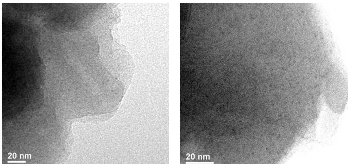
Figura 4.30. Micrografia do catalisador bimetálico 50Pt50Ni/HUSY com 130 \mu\text{mol M/g}_{\text{cat}} utilizando a ativação rápida a 500^\circ\text{C} e magnificação de 100.000 e 150.000X.
