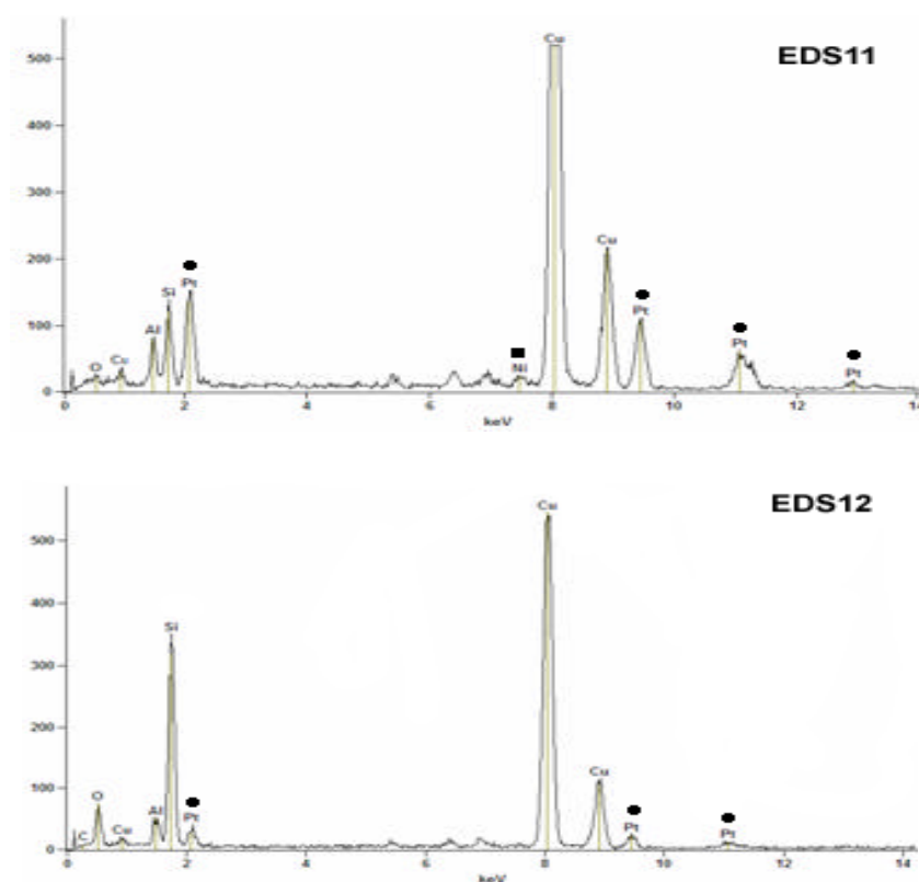
Figura 4.32. Micrografia do catalisador bimetálico 50Pt50Ni com 130 \mu\text{mol M/g}_{\text{cat}} utilizando a ativação rápida a 500^\circ\text{C} e magnificação de 300.000X e seus respectivos EDS.
