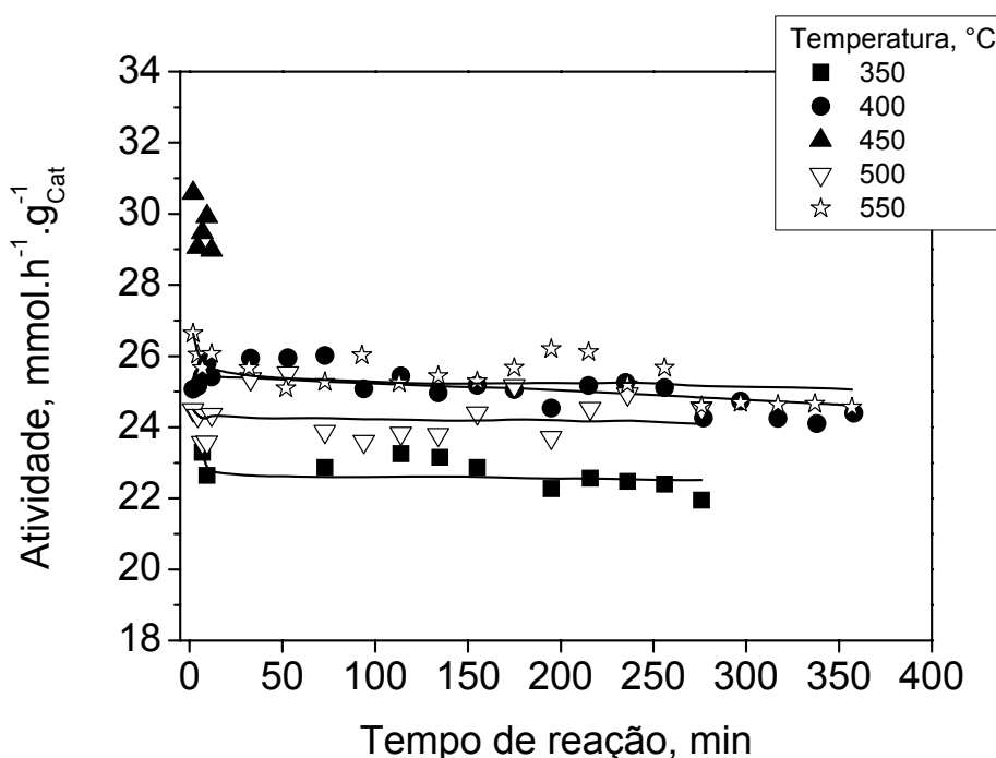
Figura 4.2. Atividade dos catalisadores bimetálicos 50Pt50Ni contendo 130 \mu\text{mol} \text{M}/\text{g}_{\text{cat}} e 1min de tempo de permanência na temperatura de redução.
