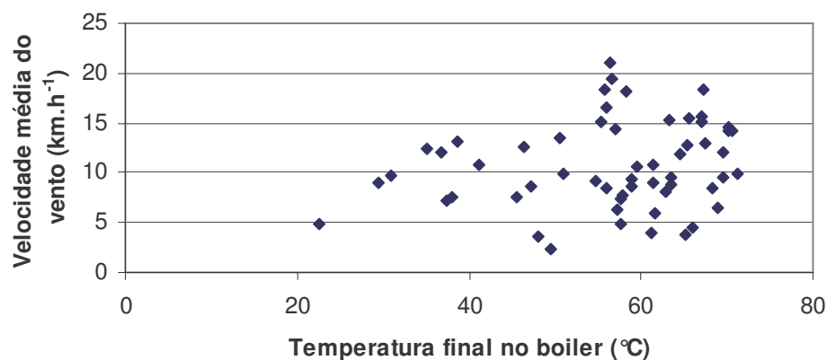
Figura 18 - Temperatura final da água no boiler em relação à velocidade do vento.
