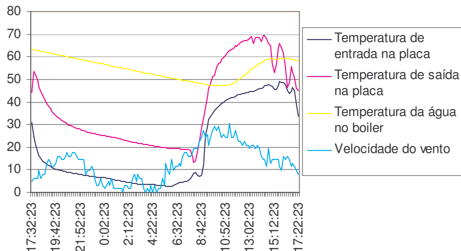
Figura 19 - Relação entre as temperaturas da água na entrada e saída da placa, da água do boiler e da velocidade do vento, no período de 24 horas.
