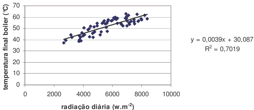
Figura 28 - Relação entre a radiação diária e a temperatura final da água no boiler .
