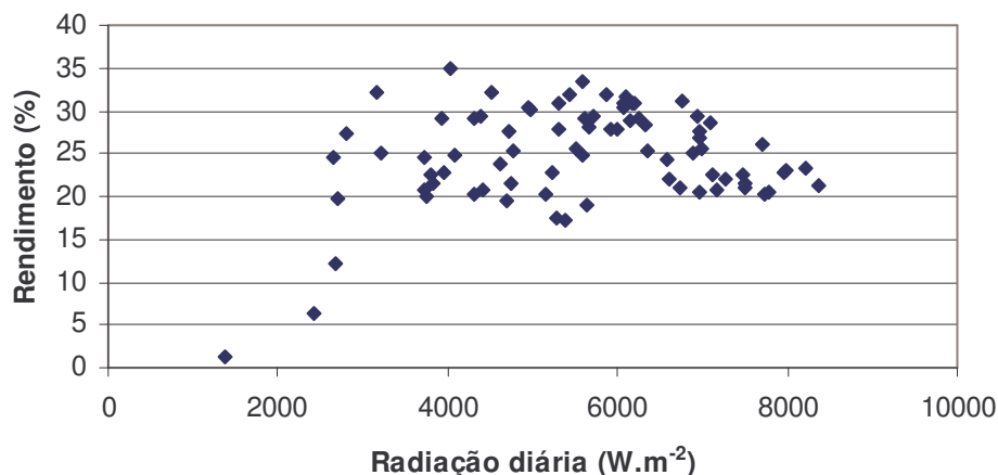
Figura 30 - Rendimento do sistema relativamente à PEE.
