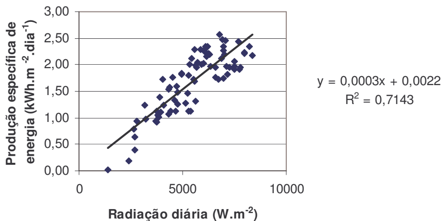
Figura 29 - Relação entre a radiação diária e a produção específica de energia.
