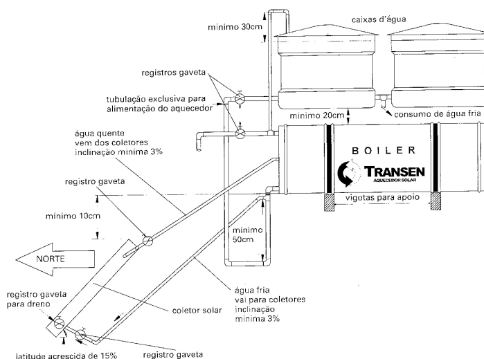
Figura 2 - Esquema de ligação de um sistema de aquecimento de água, por energia solar, para funcionar por termostifão.
