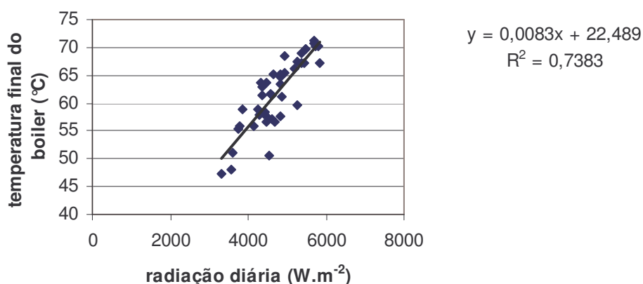
Figura 21 - Temperatura final da água no boiler em relação à radiação total diária no inverno.
