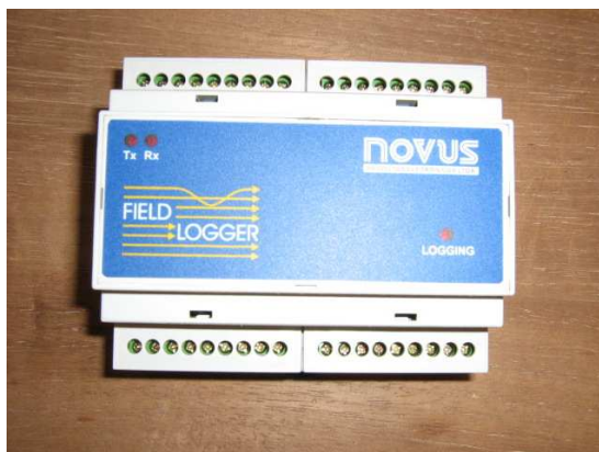
Figura 17 - Registrador eletrônico.
