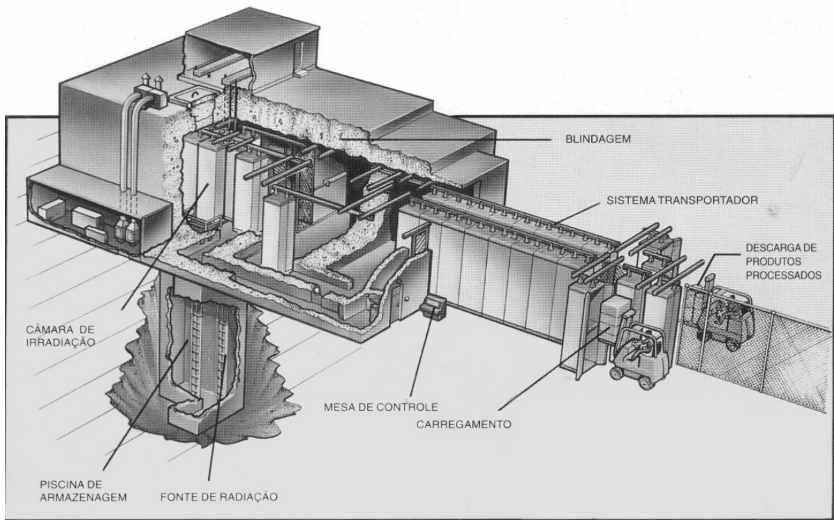
Figura 2. Irradiador comercial (DURANTE, 2002).
