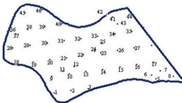
Figura 4 - Área experimental de 71 ha e grade de amostragem para o ano agrícola de 2006/2007.
