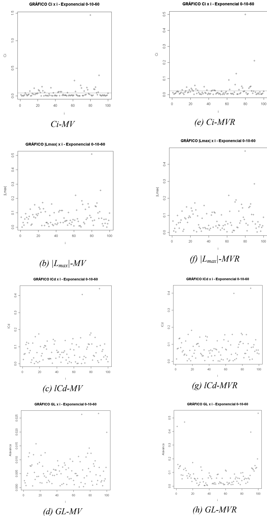
Figura 8 - Gráficos de diagnóstico C_i \times i , |L_{max}| \times i , ICd \times i e GL \times i , para a variável simulada Exponencial 0-10-60, com os estimadores MV e MVR.
