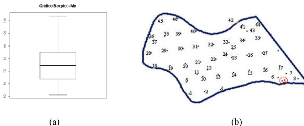
Figura 30 - Gráfico Box-plot da variável teor de manganês com os dados totais (a); Croqui da disposição amostral dos dados na área em estudo de 71 ha (b).
