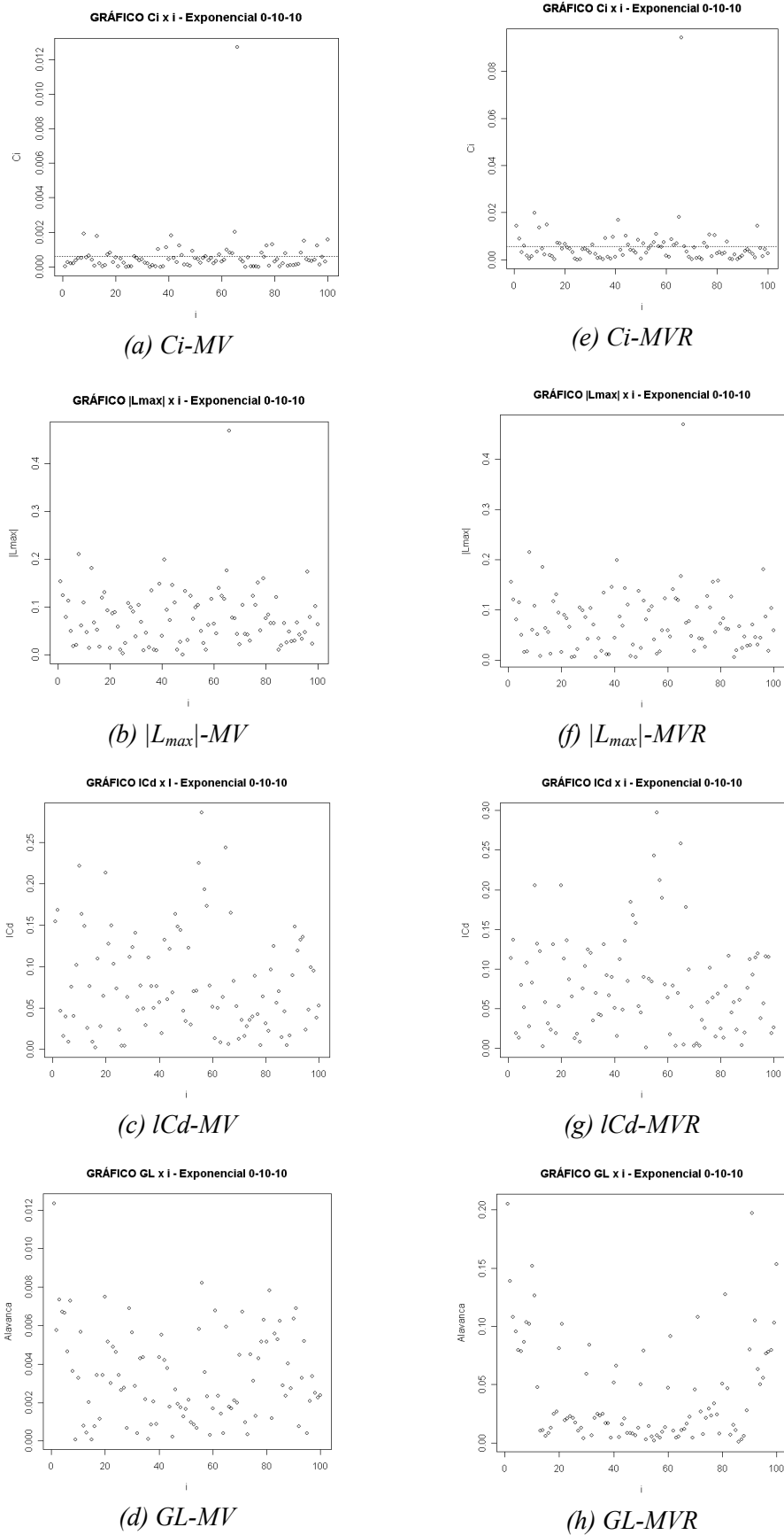
Figura 5 - Gráficos de diagnóstico C_i \times i , |L_{max}| \times i , ICd \times i e GL \times i , para a variável simulada Exponencial 0-10-10, com os estimadores MV e MVR.
