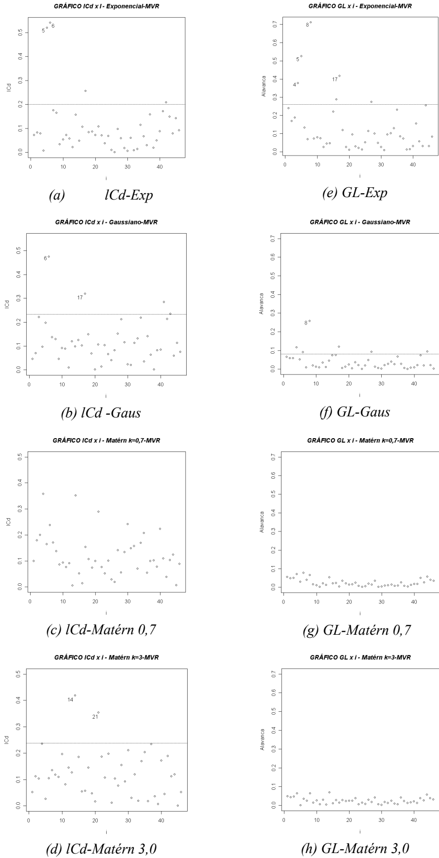
Figura 34 - Gráficos de diagnóstico ICd \times i e GL \times i , para a variável manganês, com o estimador MVR.
