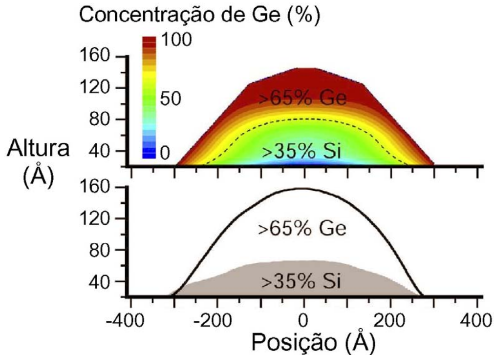
Fig. 6.14 – (a) Mapa de composição em espaço real para os domos de Ge; (b) perfis de AFM para domos de tamanho típico antes e depois do etching seletivo em solução de 31% H_2O_2 , evidenciando o núcleo rico em Si.
