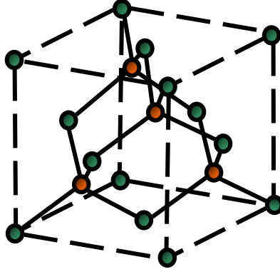
Fig. 6.3 – Célula unitária de uma estrutura zinblend de SiGe. Os átomos de Ge aparecem na cor laranja.
