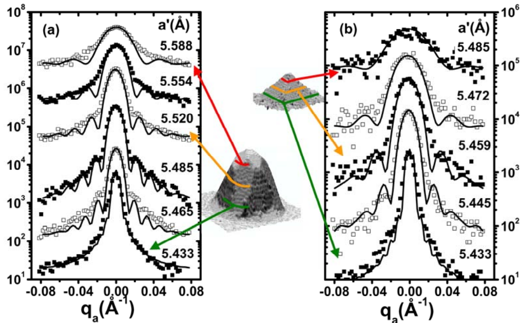
Fig. 6.5 – Varreduras angulares ao longo da direção [1-10] em diferentes parâmetros de rede locais para as amostras de domos (a) e pirâmides (b). As linhas contínuas são ajustes utilizando a eq. 6.8. As figuras que indicam esquematicamente a localização de cada região com parâmetro de rede fixo foram obtidas por microscopia de varredura por tunelamento [Rastelli02].
