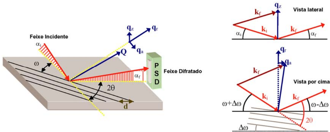
Fig. 6.1 – Geometria de difração por incidência rasante (GID). As componentes radial ( q_r ), angular ( q_a ) e vertical ( q_z ) do vetor transferência de momento são vistas em detalhe à direita.
