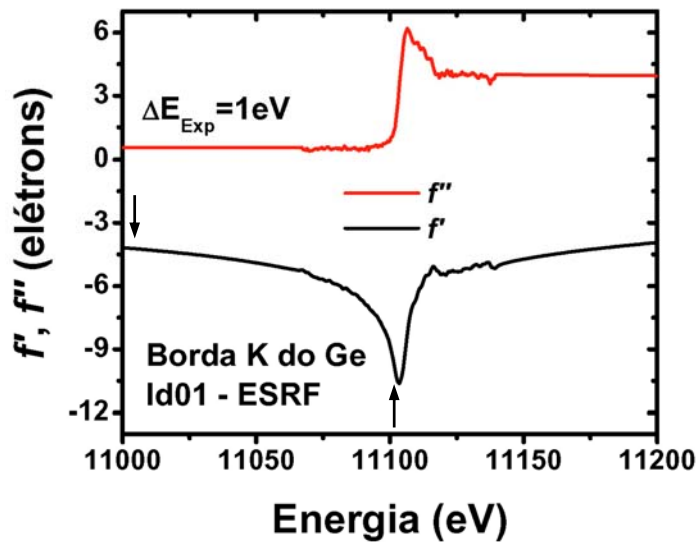
Fig. 6.2 – Correções f' e f'' do fator de espalhamento atômico do Ge próximo à borda de absorção K. Comparando-se medidas feitas nas energias assinaladas por setas é possível obter, através do contraste de intensidades espalhadas, a concentração de Ge no material estudado.
