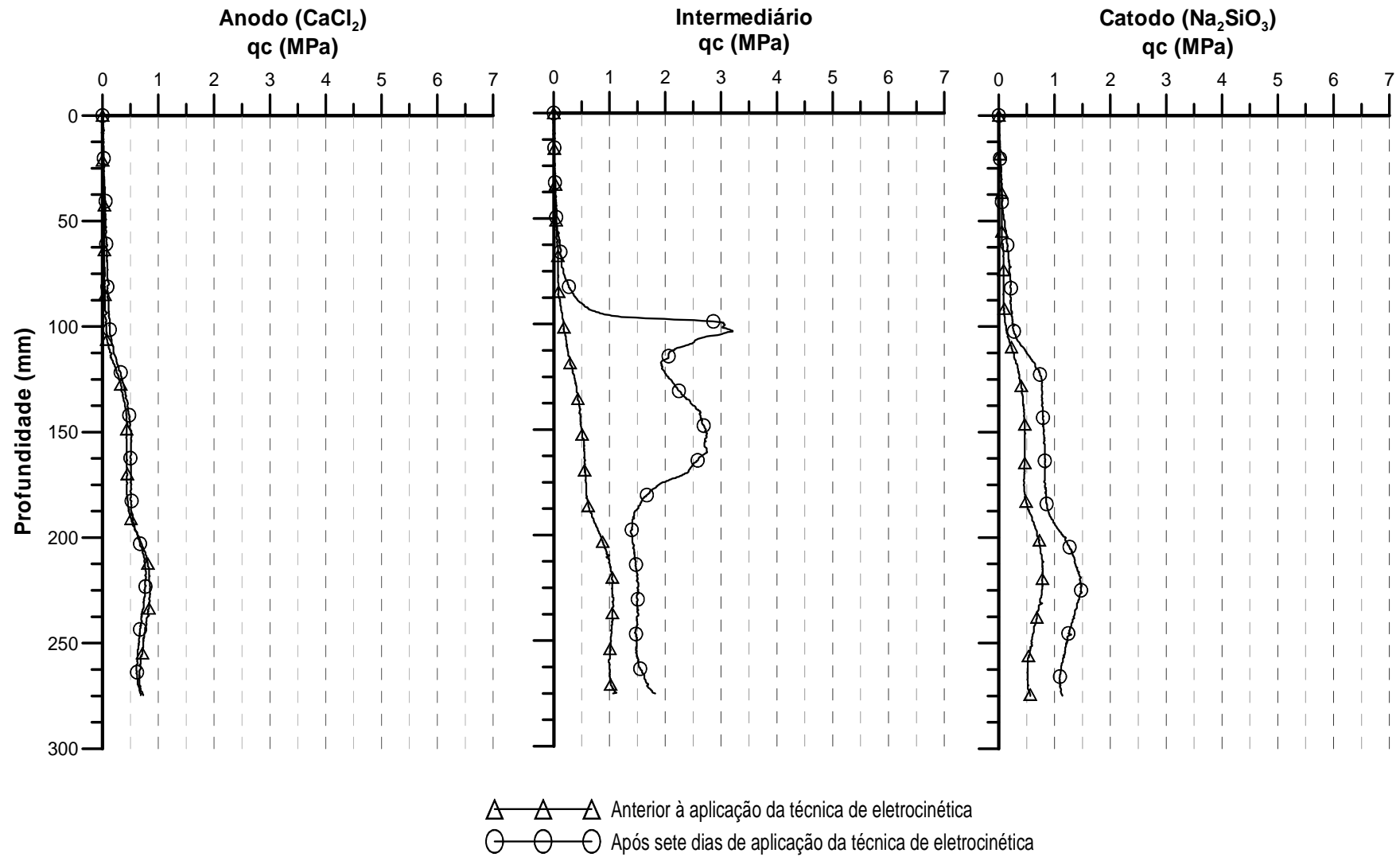
Figura 4.26: Ensaio de prospecção na célula eletrocinética 07 (C_E_07).
