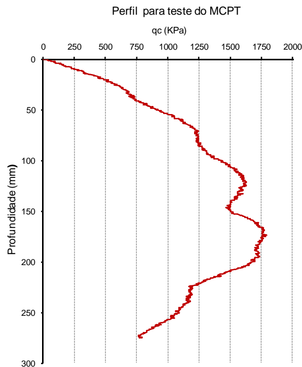
Figura 4.7: Perfil para teste do MCPT.
