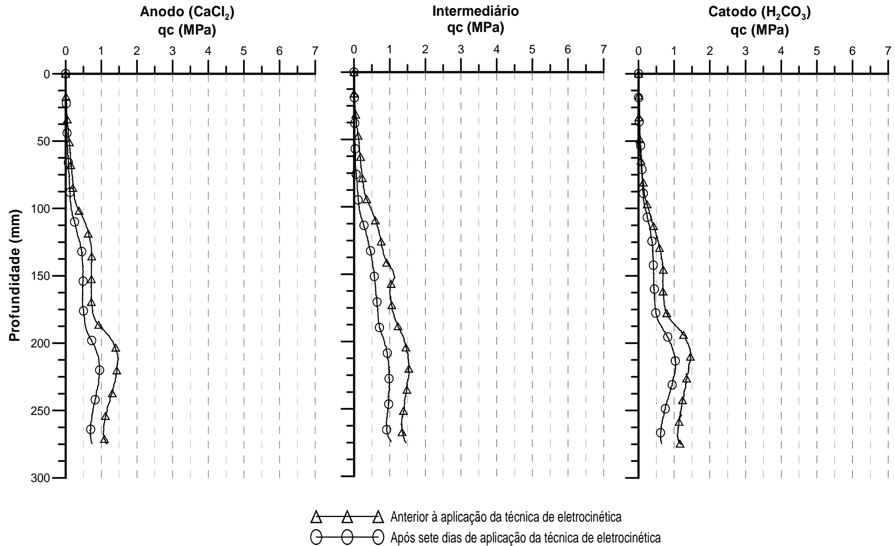
Figura 4.16: Ensaio de prospecção na célula eletrocinética 04 (C_E_04).
