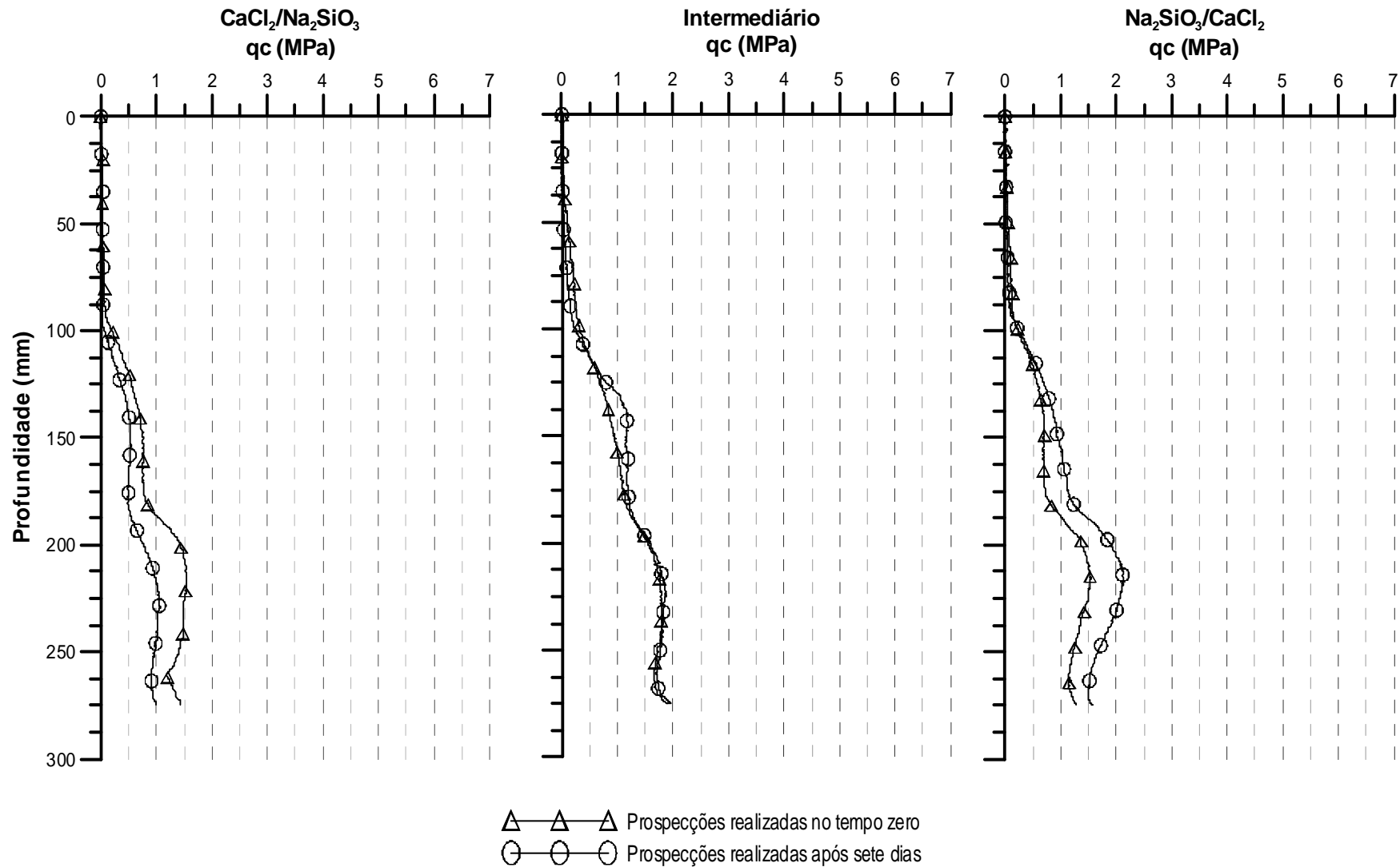
Figura 4.32: Ensaio de prospecção na célula eletrocinética 11 (C_E_11).
