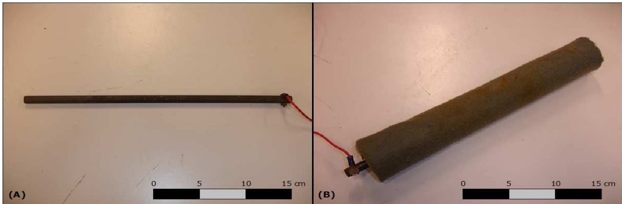
Figura 3.6: Eletrodos de aço carbono - (A) eletrodo e (B) eletrodo posicionado no interior dos drenos.
