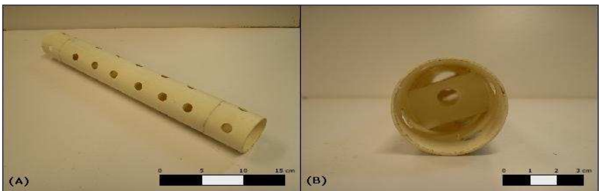
Figura 3.3: TUDO de PVC - (A) vista dos furos na parede do tubo e (B) vista do encaixe do eletrodo.
