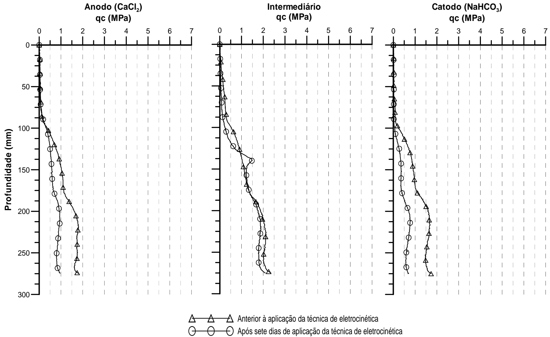
Figura 4.36: Ensaio de prospecção na célula eletrocinética 13 (C_E_13).
