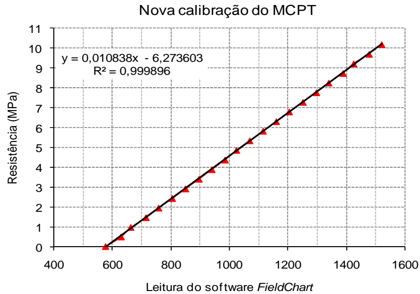
Figura 4.6: Nova curva de calibração do MCPT.
