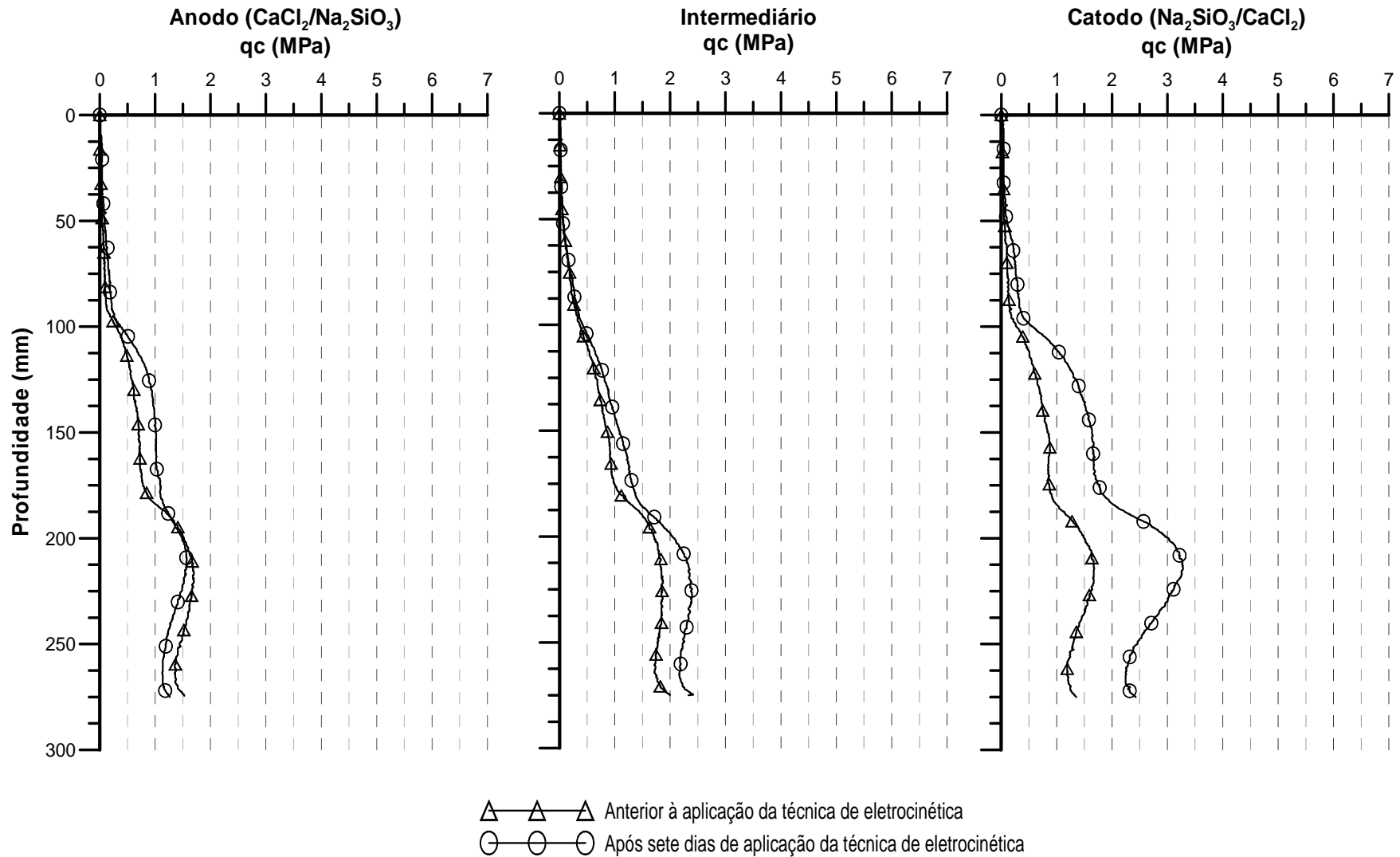
Figura 4.30: Ensaio de prospecção na célula eletrocinética 10 (C_E_10).
