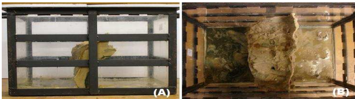
Figura 4.24: Cimentação ocorrida na C_E_07 - (A) Vista lateral e (B) Vista superior.
