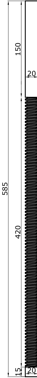
Rosca esquerda M 20 - passo 1 mm (1 peça)
