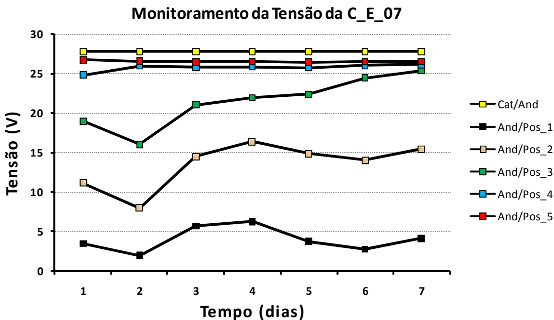
Figura 4.9: Monitoramento da tensão durante a C_E_07.
