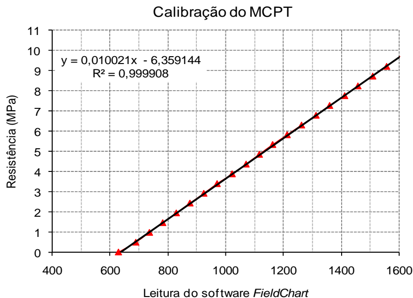
Figura 4.5: Curva de calibração do MCPT.
