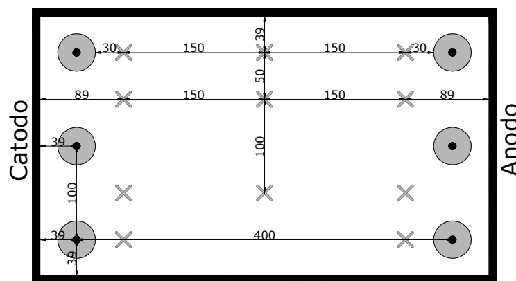
Figura 3.16: Locais dos ensaios de prospecção da C_E_02.
