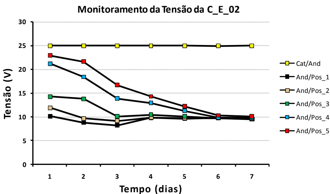
Figura 4.8: Monitoramento da tensão durante a C_E_02.
