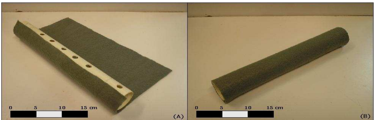
Figura 3.4: Drenos - (A) cobertura do tubo pelo geotêxtil e (B) dreno pronto.
