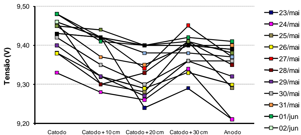
Figura 4.4: Variação de tensão durante o segundo ensaio.
