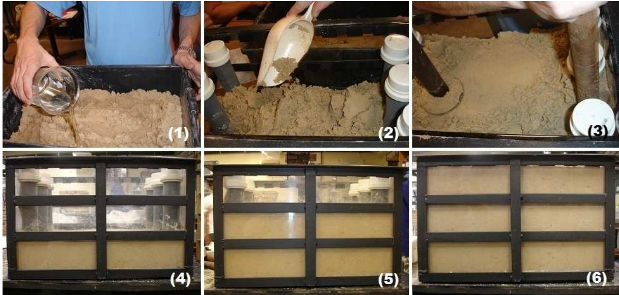
Figura 3.13: Preparação do corpo de prova de uma célula eletrocinética.
