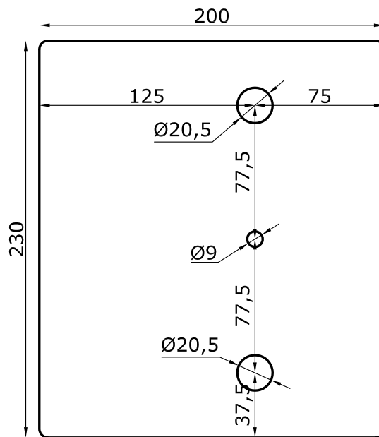
Placa metálica de ¼" de espessura (1 peça)
