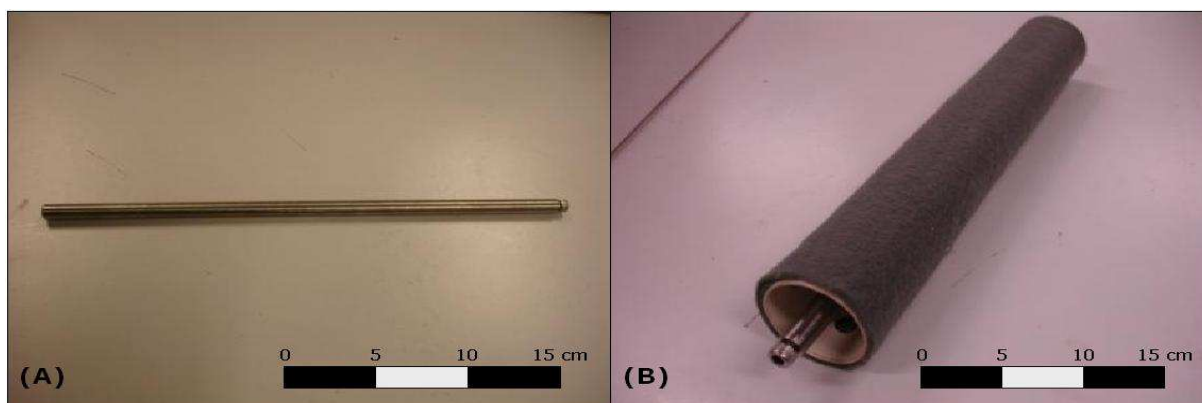
Figura 3.5: Eletrodos de titânio - (A) eletrodo e (B) eletrodo posicionado no interior dos drenos.
