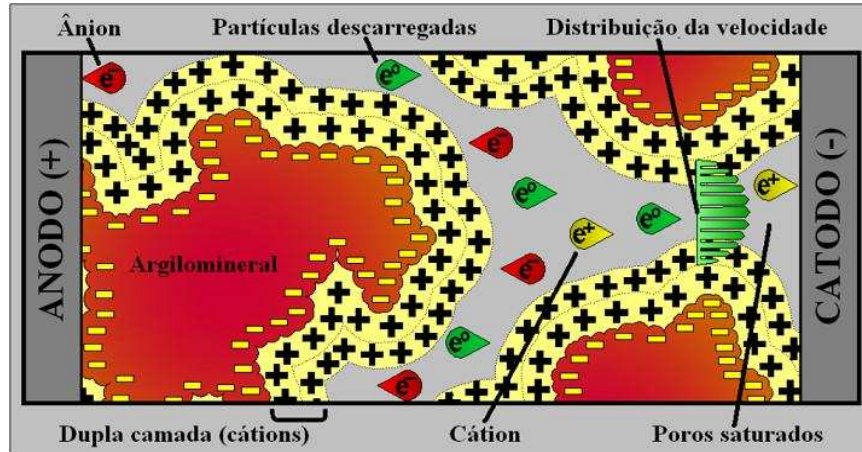
Figura 2.2: Eletrosmose e eletromigração.
