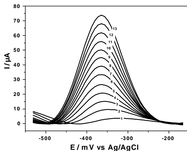
Figura 3.12: Voltamogramas de onda quadrada para diferentes concentrações de \text{N}_2\text{H}_4 sobre GP/FeTPyPz em \text{NaOH} 0,1 \text{ mol L}^{-1} com a = 40 \text{ mV} , \Delta E_s = 8 \text{ mV} e f = 30 \text{ s}^{-1} , onde: 1) 5; 2) 15; 3) 24; 4) 34; 5) 43; 6) 52; 7) 61; 8) 70; 9) 78; 10) 87; 11) 95; 12) 104; 13) 111 \mu\text{mol L}^{-1} .
