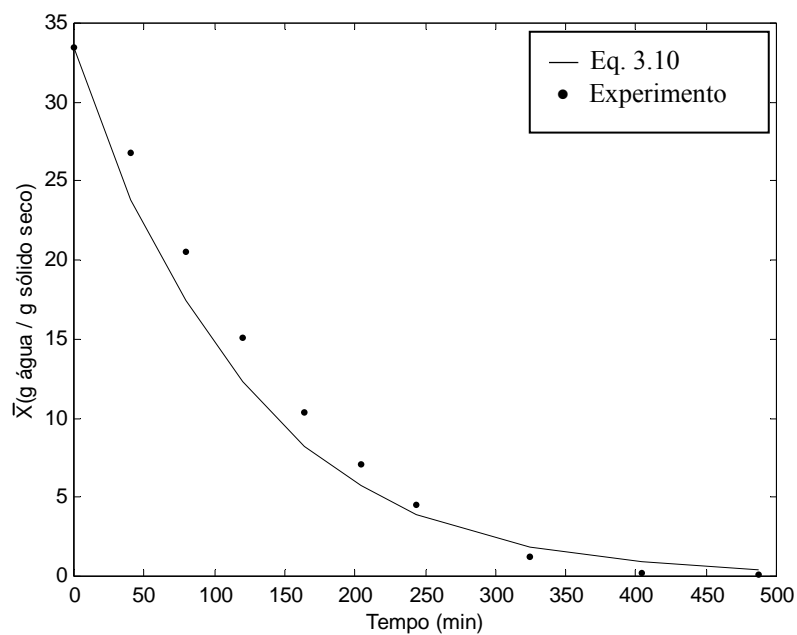
Figura 7.13: umidade média em função do tempo, com V_a=2,0 m/s, D_0=2,66 cm e T_a=50^\circ\text{C} . Modelo bidimensional com número de Biot de massa local.
