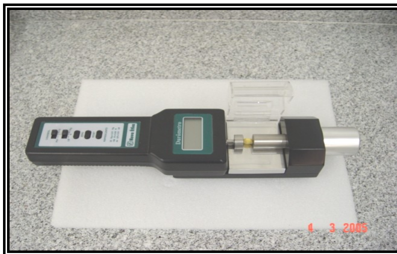
Figura 13- Durômetro digital
