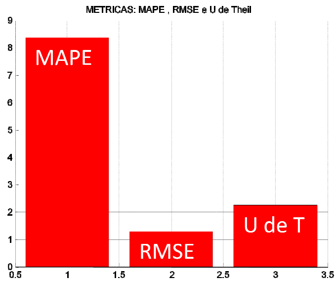
Figura 4-5 Utilização de séries sem tratamento estatísticos - métricas
