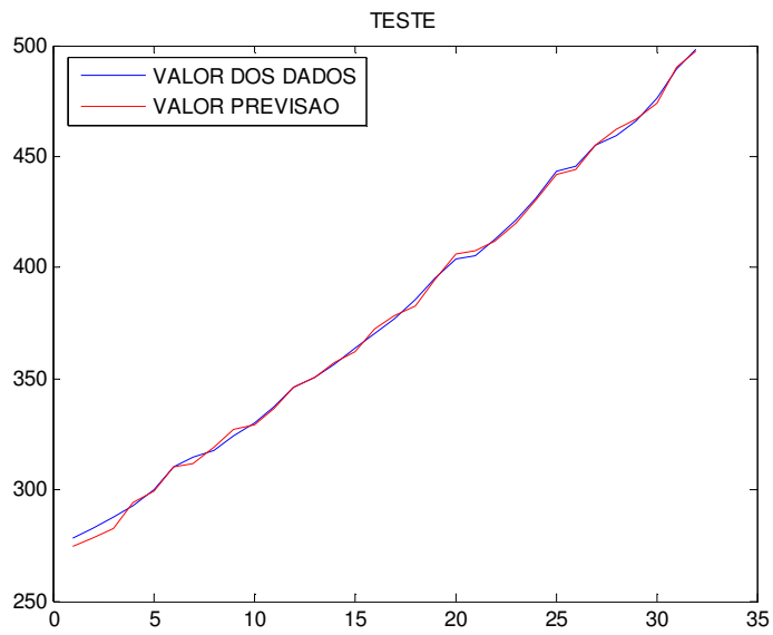
Figura 4-7 Utilização de séries com tratamento estatísticos - teste
