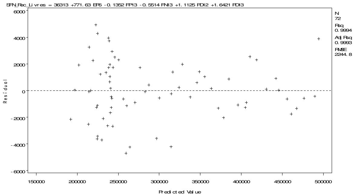
Figura 4-2 Análise resíduos
