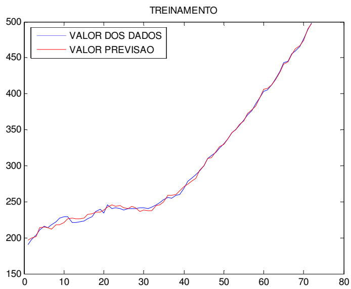
Figura 4-5 Utilização de séries sem tratamento estatísticos - métricas
