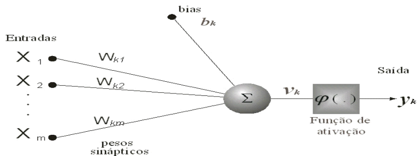
Figura 3-1 Modelo não-linear de um neurônio – Haykin 2001
