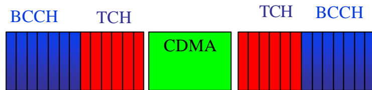
Figura 26 – Sugestão para Disposições dos BCCHs
