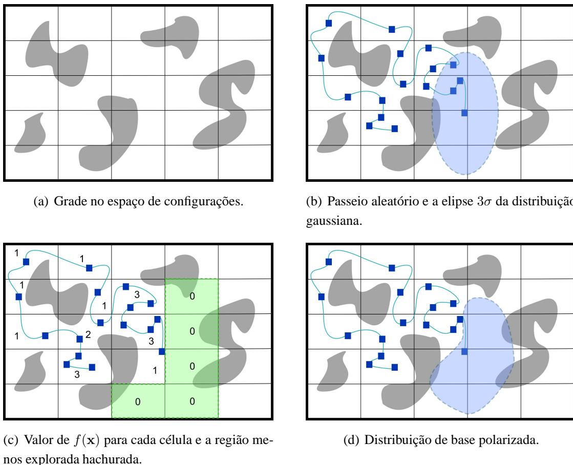
Figura 5.6: Utilização de grades como métrica de explorabilidade para polarização da distribuição de base do ARW.
