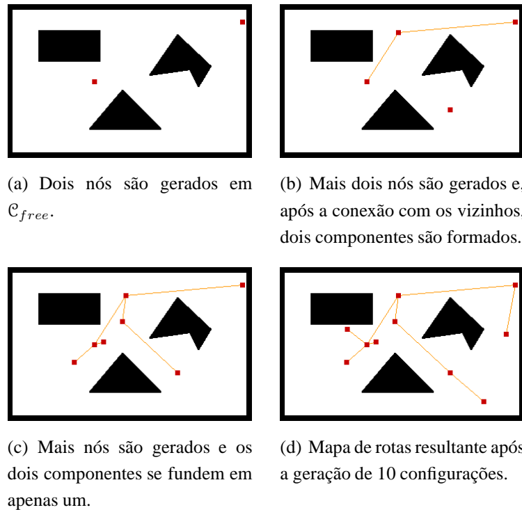
Figura 3.4: Evolução da construção do mapa de rotas no algoritmo PRM.
