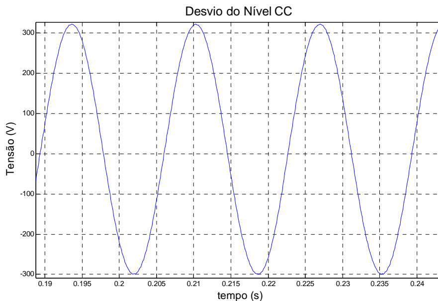
Figura 3. 20 - Forma de onda da tensão com desvio do nível CC no valor de +10V.
