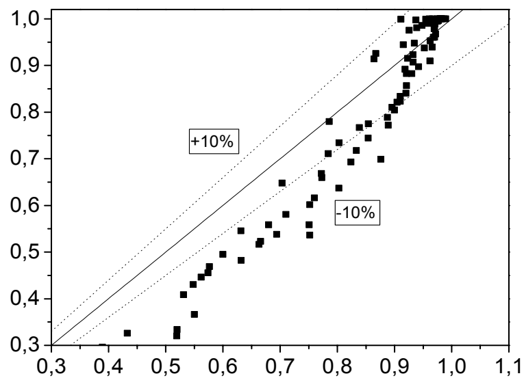
Figura 4. 14 - Eficiências de coleta experimental e teórica em relação a d_p (Equação de PAYET et al. (1992)) para o filtro de poliéster.
