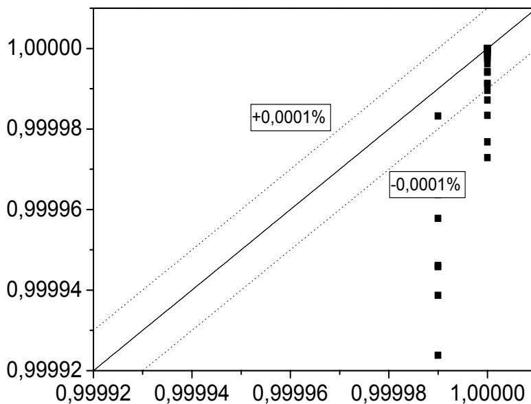
Figura 4. 38 - Eficiências de coleta experimental e teórica em relação a d_p (Equação de PAYET et al. (1992)) para o filtro HEPA.
