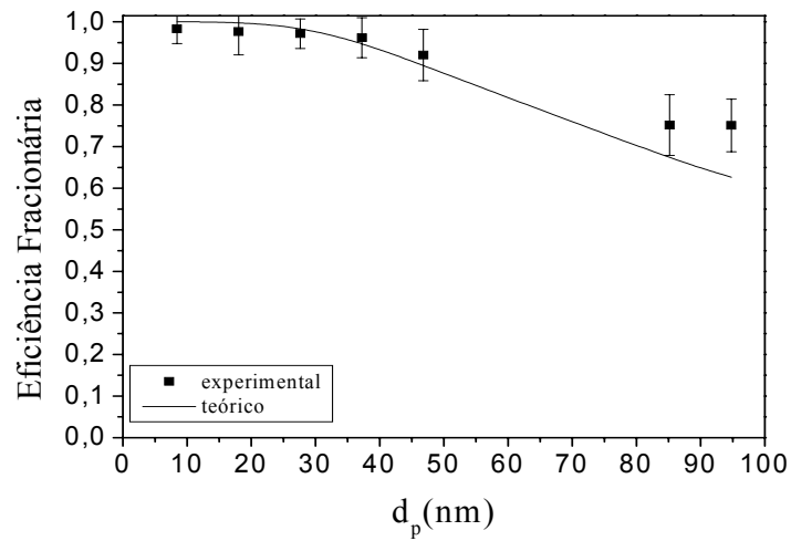
Figura J. 3 – Eficiência experimental e teórica do poliéster em relação ao diâmetro das partículas para U_0=5,0 cm/s.
