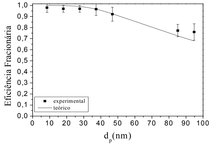
Figura J. 2 – Eficiência experimental e teórica do poliéster em relação ao diâmetro das partículas para U_0=4,0 cm/s.
