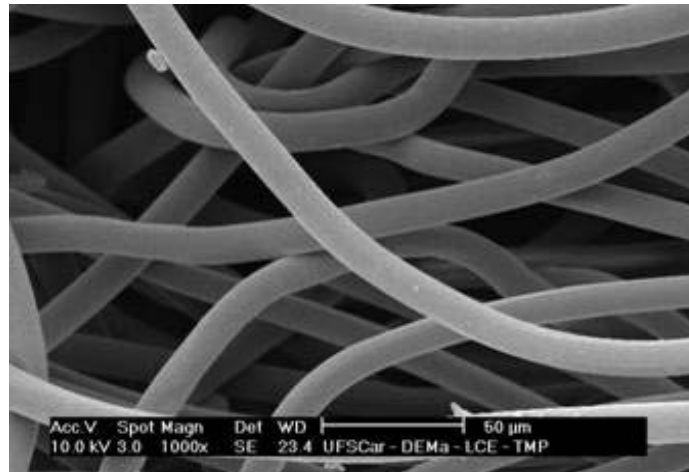
Figura 3. 14 - Vista do filtro de Poliéster
