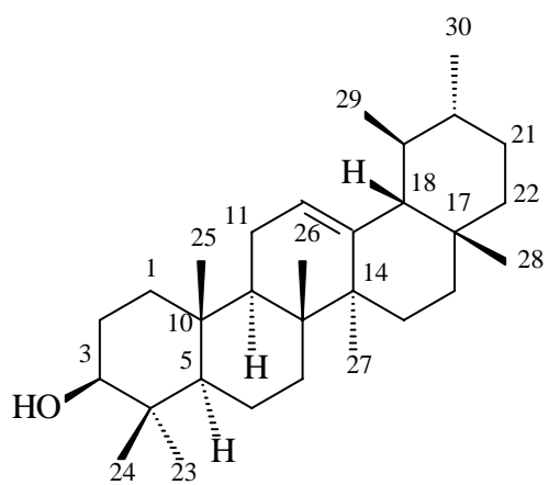
\alpha - amirina
