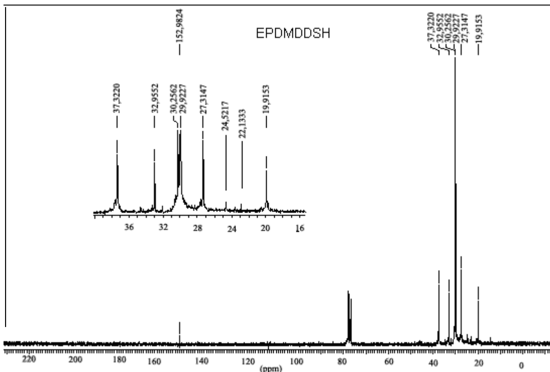
Figura 19. Espectroscopia de ressonância magnética nuclear C^{13} do EPDMDDSH
