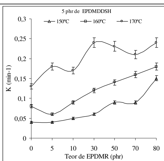
Figura 40. Efeito da temperatura na constante de velocidade em função do teor de EPDMR, misturas compatibilizadas
