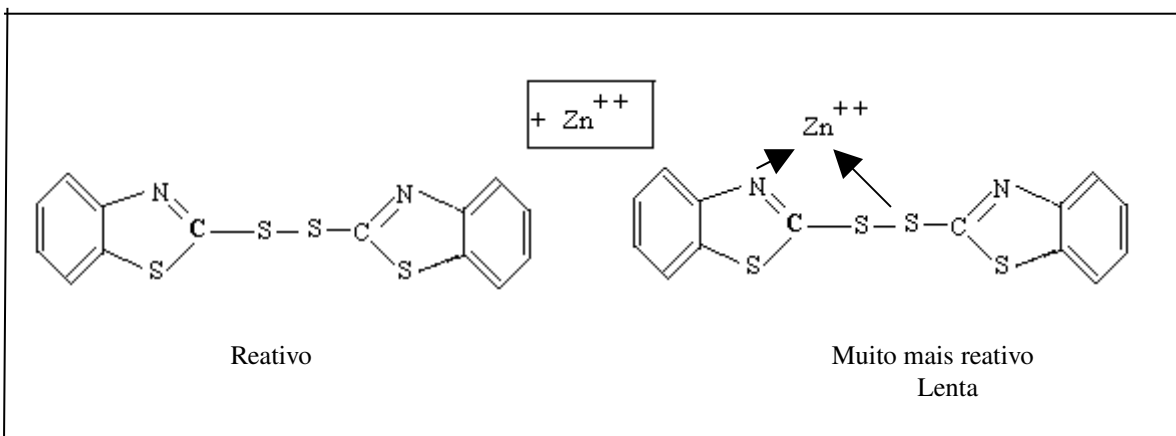
Figura 7. Esquema representativo da participação do ZnO na ativação do sistema de vulcanização (MARK et al , 1994)
