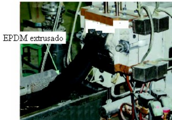
Figura 3. Processo de extrusão: EPDM saindo do orifício da extrusora (FUKUMORI & MASUSHITA, 2002).
