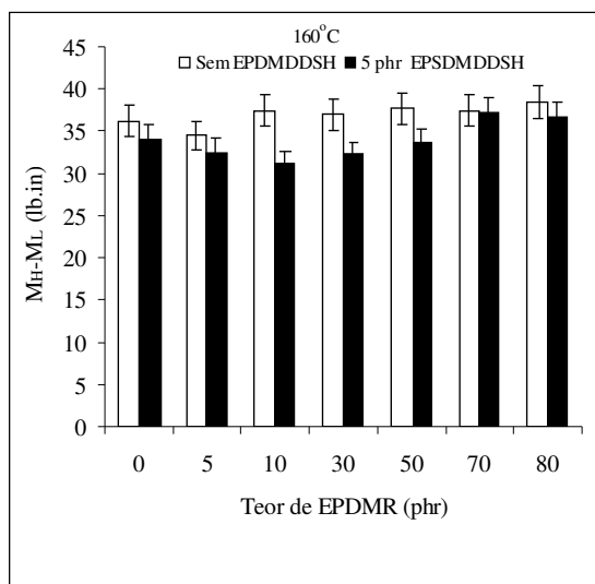
Figura 20 b. Efeito da adição de EPDMDDSH na variação da diferença do torque a 160°C
