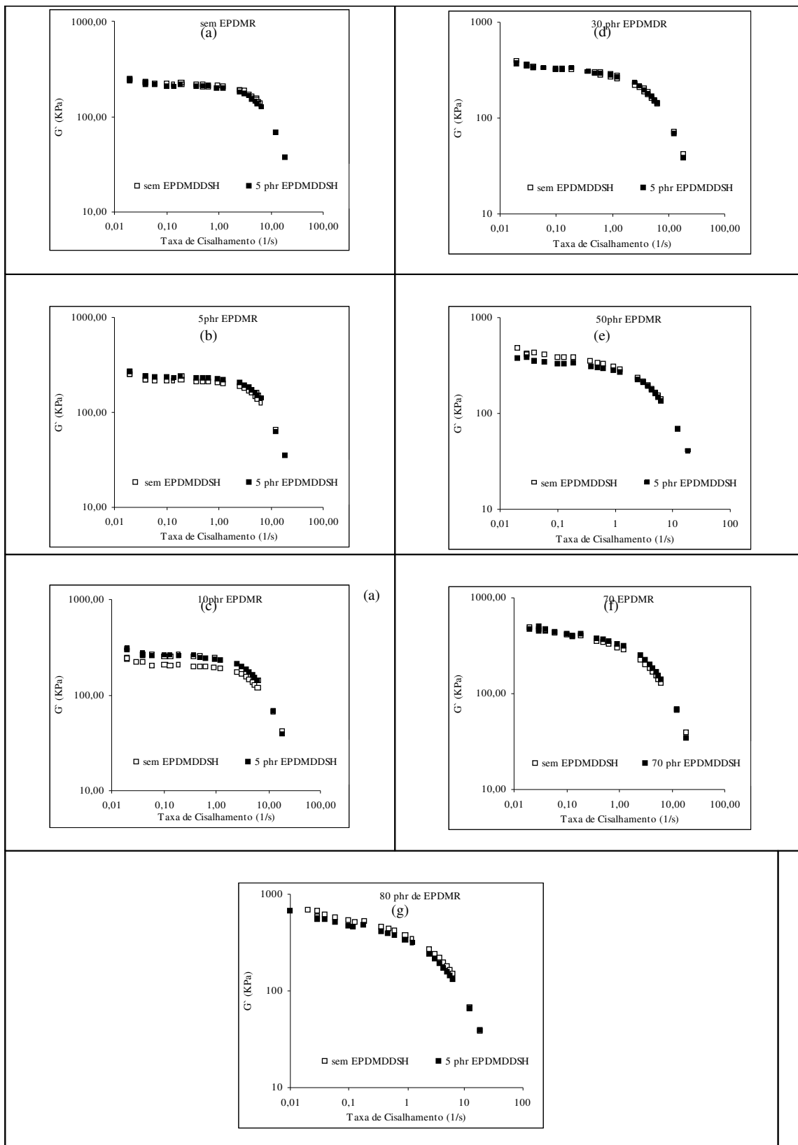
Figuras 32 a, b, c, d, e, f e g, variação do módulo elástico com taxa de cisalhamento das misturas 0, 5, 10, 30, 50, 70 e 80 phr de EPDMDR não vulcanizadas, respectivamente.
