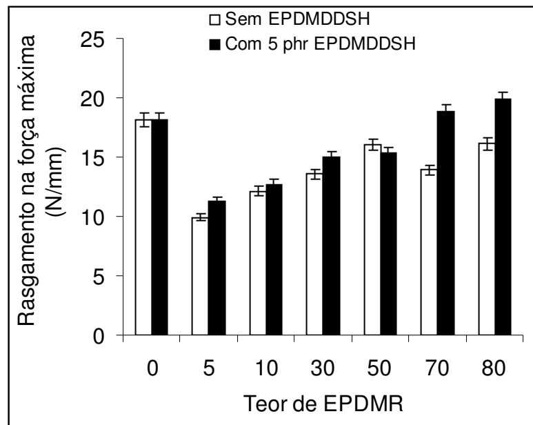
Figura 27. Efeito do EPDMDDSH e do teor de EPDMR na resistência ao rasgamento das composições de EPDM
