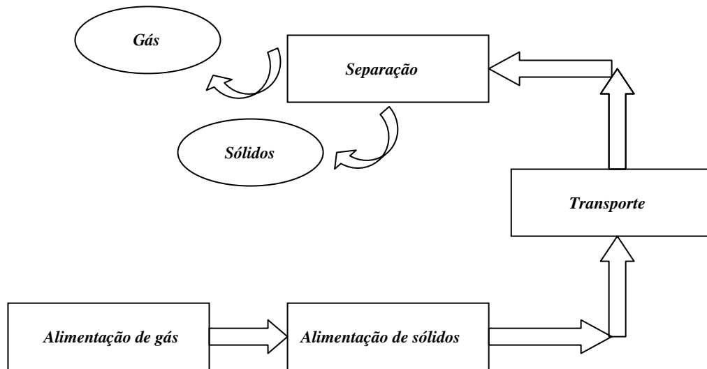
Figura 2.2 – O sistema de transporte pneumático (Marcus et al. , 1990).
