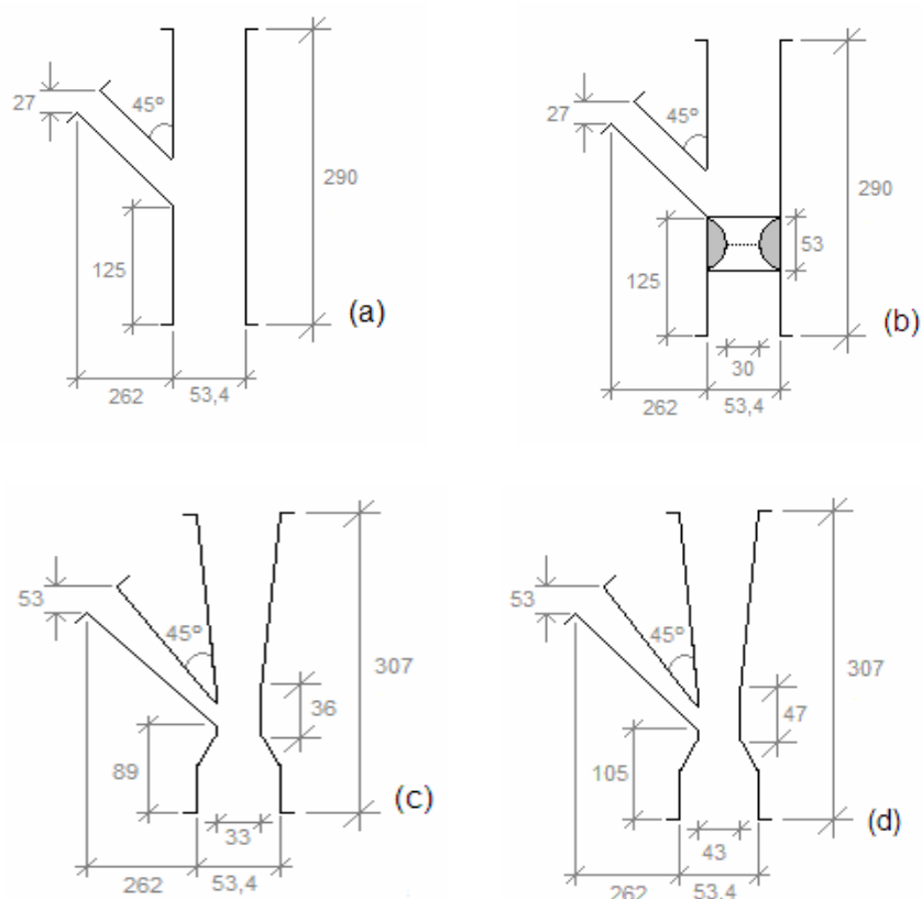
Figura 3.2: Configurações de alimentação. (a) Sem restrição; (b) bocal redutor; (c) Venturi 33 mm; (d) Venturi 43 mm. Desenhos fora de escala; dimensões em mm.
