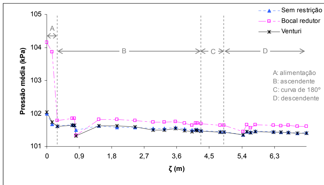
Figura 4.3 – Pressão estática média ao longo do leito para Q_f = 0,03 \text{ m}^3/\text{s} nas três configurações de alimentação.
