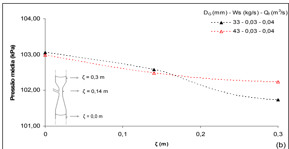
Figura 4.14: Pressão média ao longo do alimentador Venturi. (a) 0,85 mm; (b) 2,0 mm.
