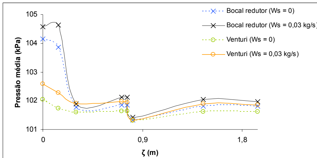
Figura 4.8 – Pressão média ao longo da região de aceleração do leito para Q_f = 0,03 \text{ m}^3/\text{s} ; W_s = 0 e 0,03 \text{ kg/s} , para as configurações de alimentação bocal redutor e venturi.
