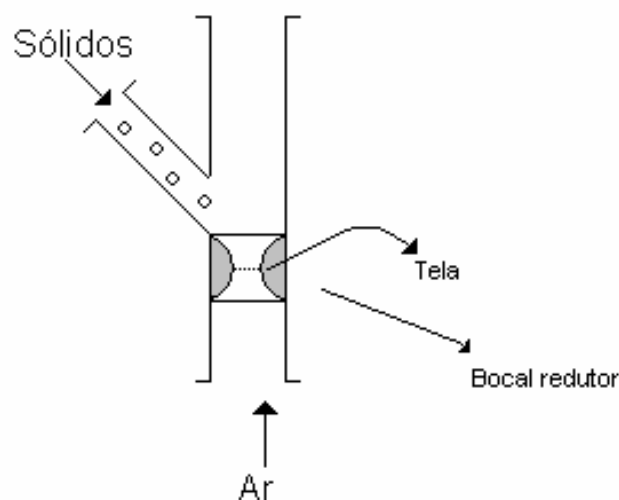
Figura 2.5 – Bocal redutor.
