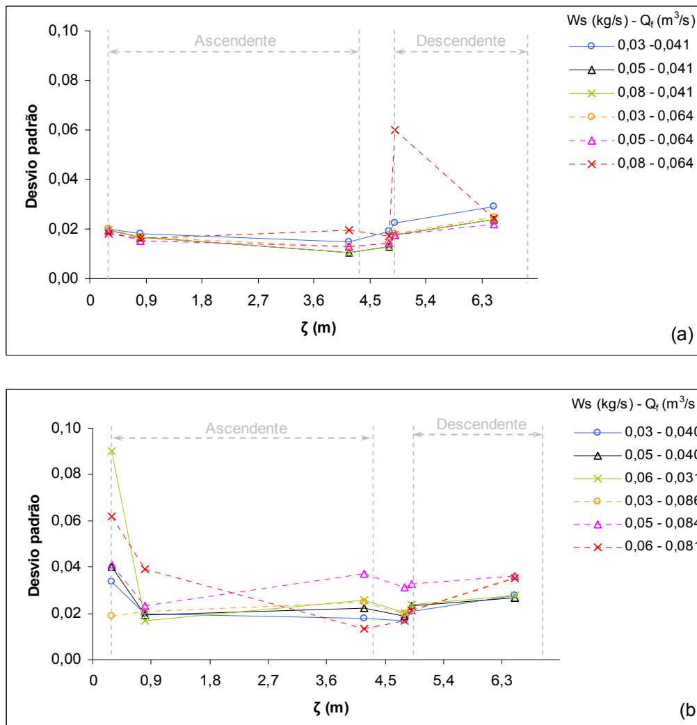
Figura 4.11 – Desvio padrão ao longo do leito para diferentes condições operacionais e d_p = 2,0 mm. (a) Alimentador gravitacional com bocal redutor; (b) alimentador gravitacional combinado com Venturi.
