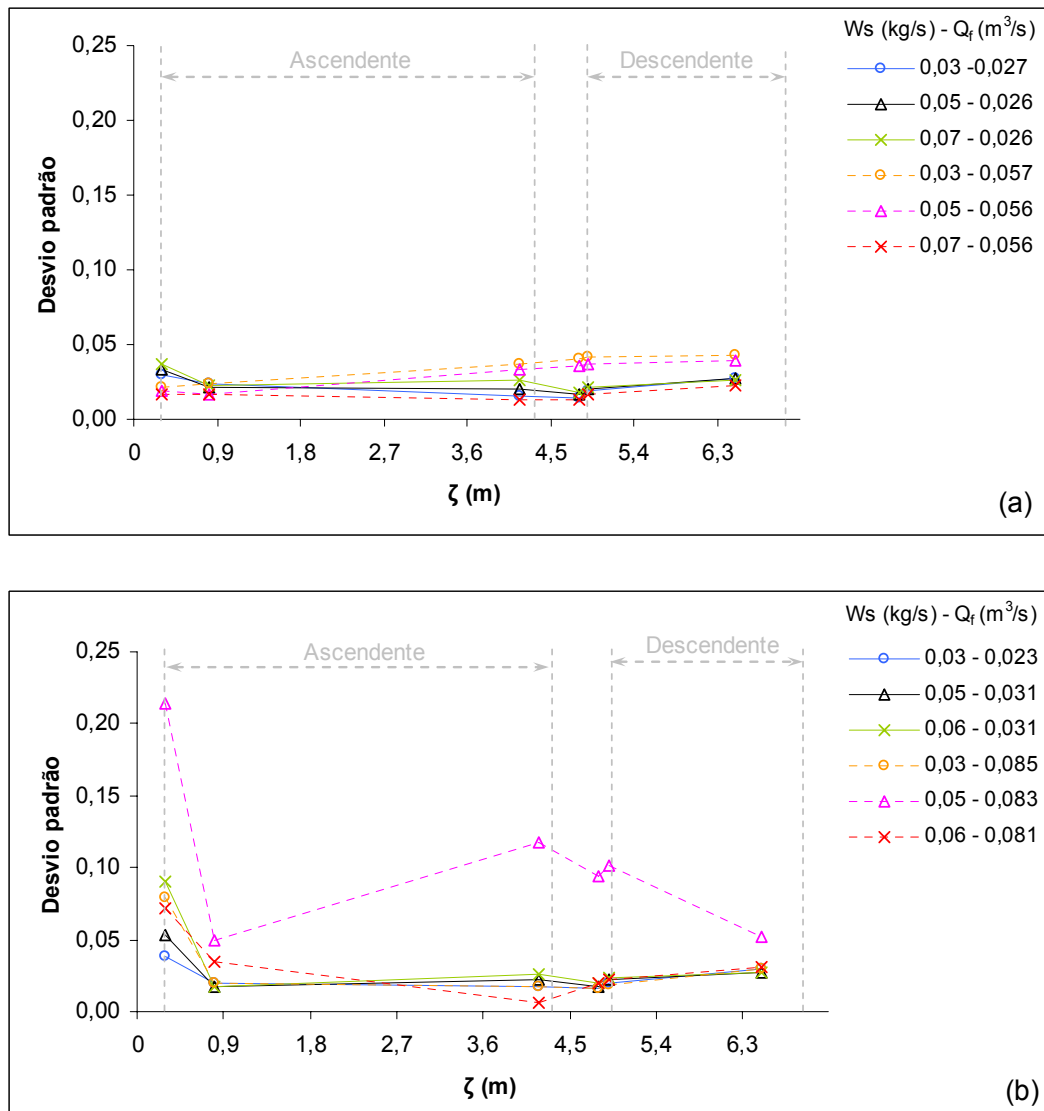
Figura 4.7 – Desvio padrão ao longo do leito para diferentes condições operacionais e dp = 0,85 mm. (a) Alimentador gravitacional com bocal redutor; (b) alimentador gravitacional combinado com Venturi.
