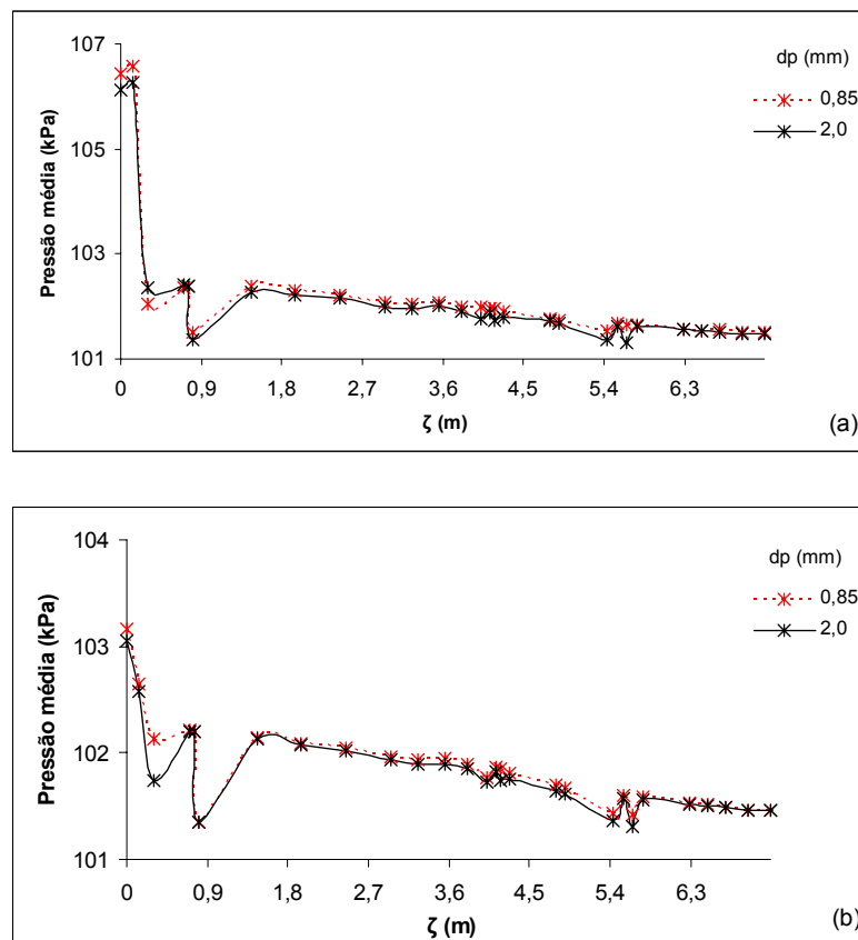
Figura 4.12: Pressão média ao longo do leito para Q_f = 0,04 \text{ m}^3/\text{s} e W_s = 0,03 \text{ kg/s} . (a) Alimentador gravitacional combinado com bocal redutor; (b) alimentador gravitacional combinado com Venturi.
