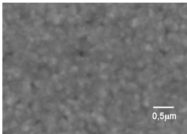
FIG. 6.14 Micrografias obtidas por MEV (30000x) de filmes de ZnTe depositados sobre vidro/SnO 2 :F com temperatura de fonte de 680°C.
