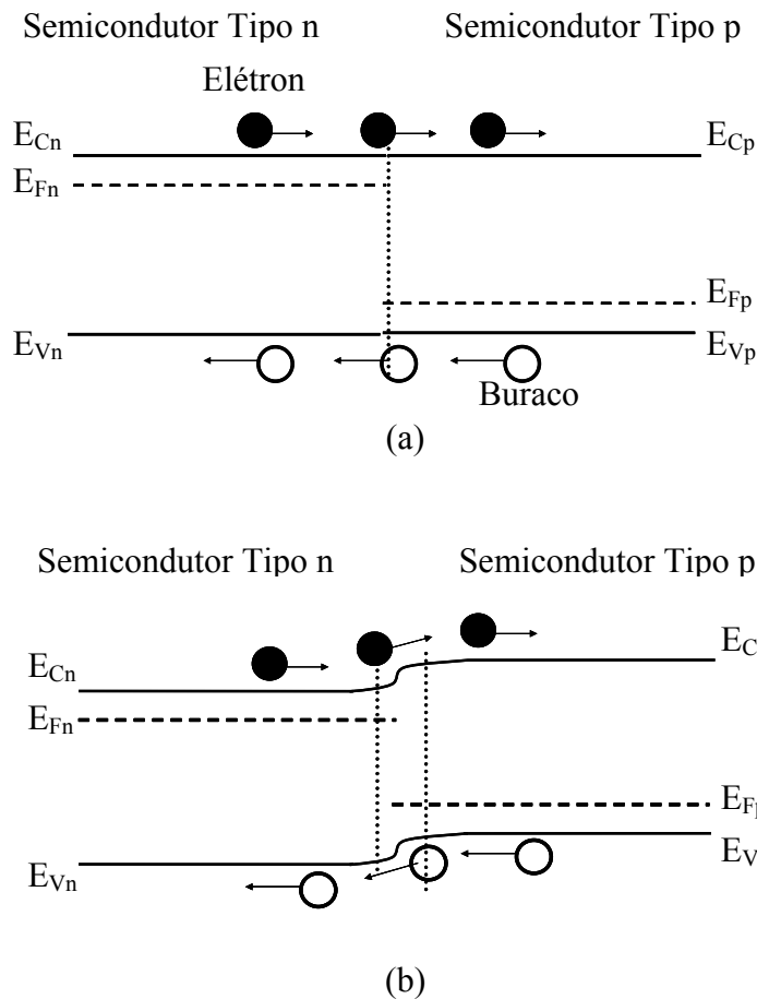
FIG. 2.5 Processo de formação da região de depleção de uma junção pn
