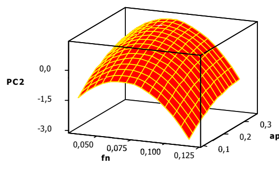
Figura 4.11 – Experimentos de confirmação: Superfície de Resposta para PC_2
