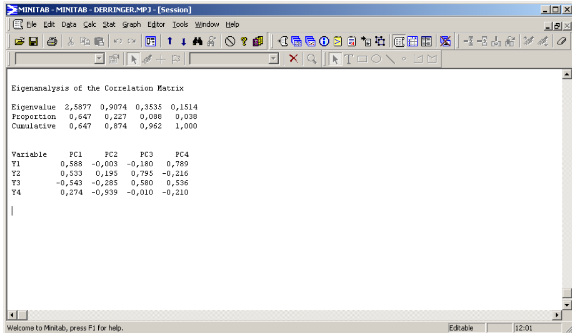
Figura 6.4 – Análise de componentes principais
