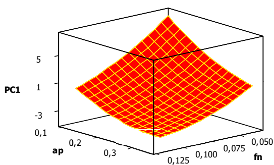
Figura 4.10 – Experimentos de confirmação: Superfície de Resposta para PC_1
