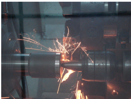
Figura 4.12 – Experimentos de confirmação: Início do processo de torneamento
