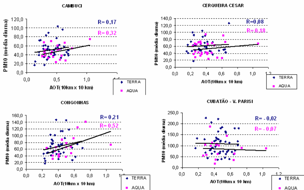
Figura 4.3: Diagramas de Dispersão e correlações entre a média diurna da concentração de material particulado MP_{10}(\mu\text{g}/\text{m}^3) nas estações da CETESB e a AOD média (10 km x 10 km), para os meses de junho, julho e agosto.
