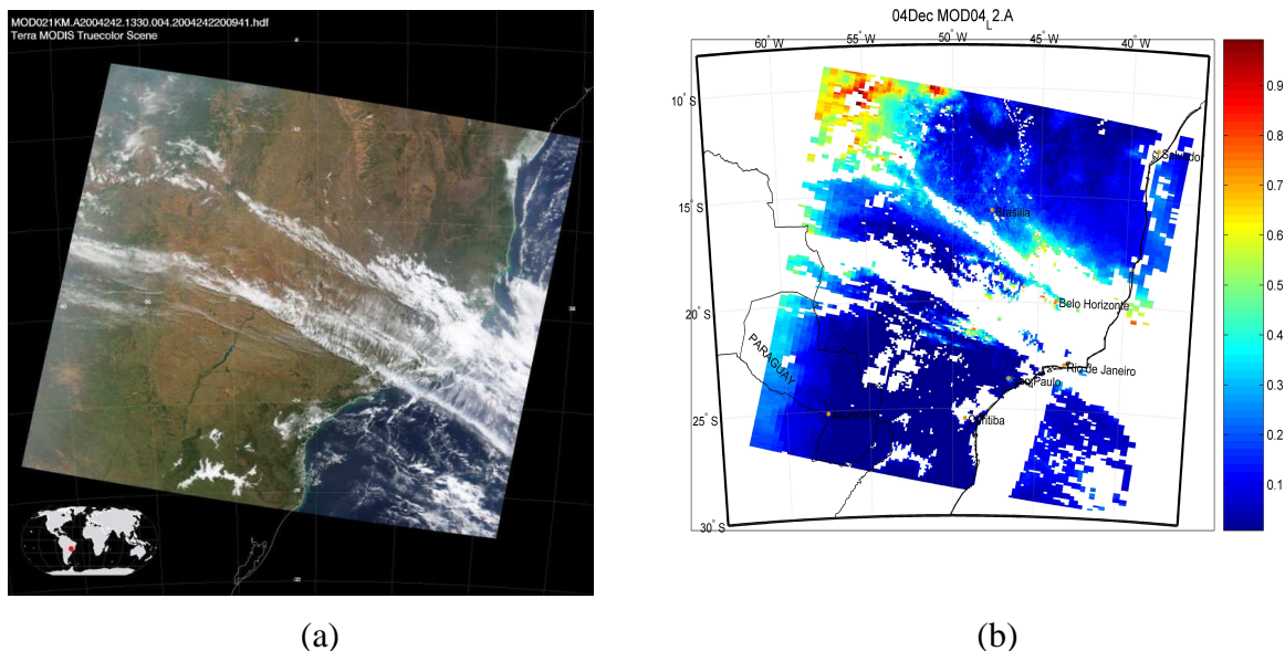
Figura 1.12: a) Imagem do sensor MODIS, no visível, a bordo do satélite TERRA para o dia 04 de dezembro de 2004 sobre a RMSP, b) Imagem da mesma área, mostrando o produto de AOD utilizado pela NASA.
