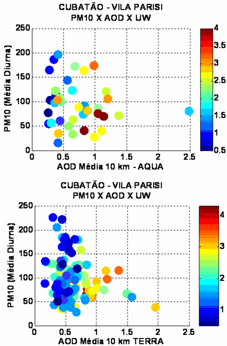
Figura 4.13 (a): Diagrama de dispersão entre o Material Particulado Fino e a AOD Média de 10 km x o Vapor d'água (cm)- barra de cores. No topo para o satélite AQUA e na base para o satélite TERRA. Estação de Cubatão V. Parisi.
