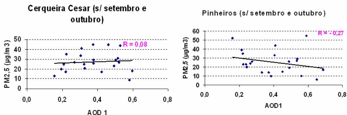
Figura 4.19: Diagramas de dispersão e correlações entre a concentração de material particulado fino MP_{2,5} ( \mu\text{g}/\text{m}^3 ) e a AOD1 sem os meses de setembro e outubro.
