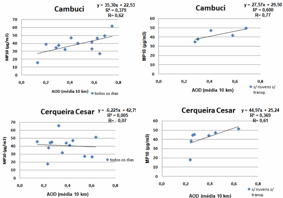
Figura 4.24: Diagramas de dispersão e correlações entre a concentração de MP_{10} ( \mu\text{g}/\text{m}^3 ) – média diurna e AOD média 10 km x 10 km. À esquerda todos os dias disponíveis para cada estação e à direita somente dias sem a presença de nuvens e sem a observação de aerossol acima da CM.
