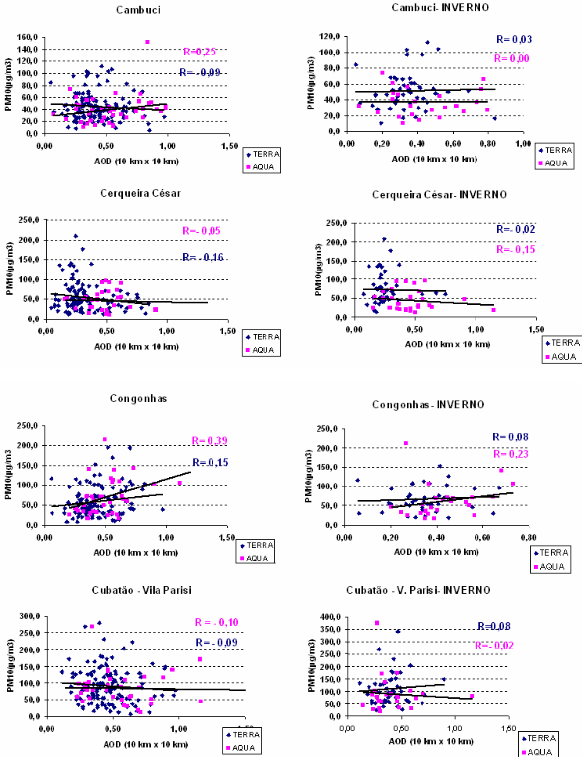
Figura 4.1: Diagramas de Dispersão e correlações entre a concentração de material particulado MP_{10}(\mu\text{g}/\text{m}^3) nas estações da CETESB e a AOD média (10 km x 10 km). À esquerda é mostrada a dispersão para todo o período e a direita somente médias no período de inverno. Curva do TERRA média horária das 11 h e do AQUA das 13 h, para o MP_{10} .
