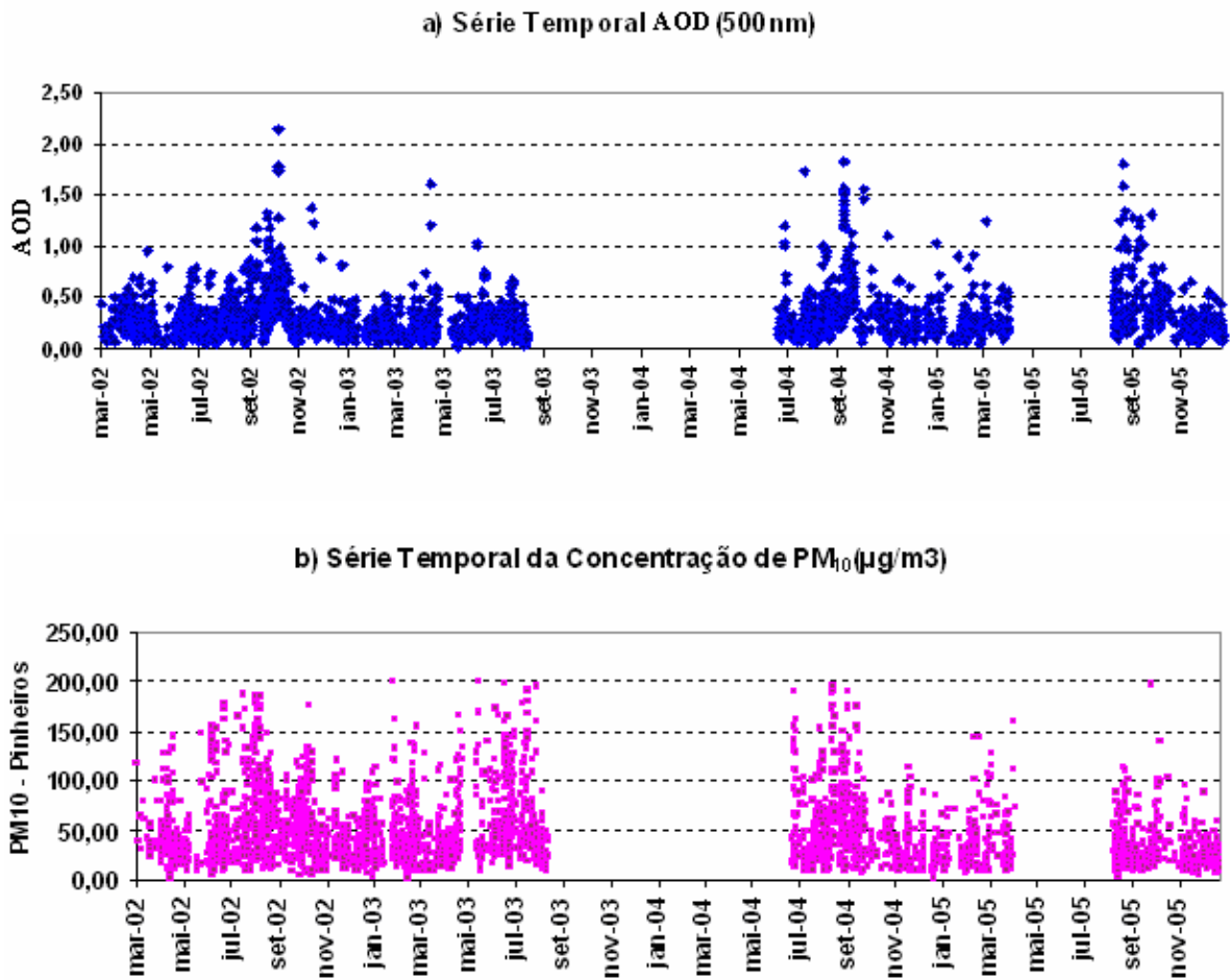
Figura 4.6: a) Séries temporais de profundidade óptica de aerossol em 500 nm, b) Séries temporais da concentração de material particulado, em \mu\text{g}/\text{m}^3 .
