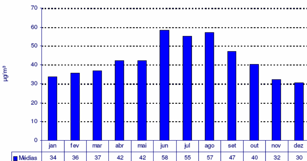
Figura 1.5: Concentrações Médias Mensais de MP_{10} de 2002 a 2006 na RMSP (CETESB, 2007).
