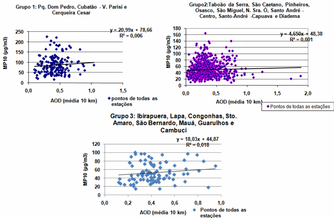
Figura 4.11: Correlações entre MP_{10} e a AOD (média 10 km) para os 3 grupos de estações.
