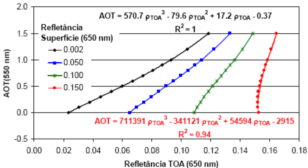
Figura A- 4: Equações de inversão da refletância no TOA em profundidade óptica (AOD), definidas para uma condição específica de posições angulares do Sol e do sensor, para o modelo de aerossol 3 e algumas refletâncias de superfície ( \rho_{sup}(650) = 0,002; 0,05; 0,1; 0,15 ). Os cálculos das refletâncias no topo da atmosfera (650 nm) para diferentes \tau_a (550 nm) foram realizados com o código de transferência radiativa SBDART. Fonte: Castanho (2005).
