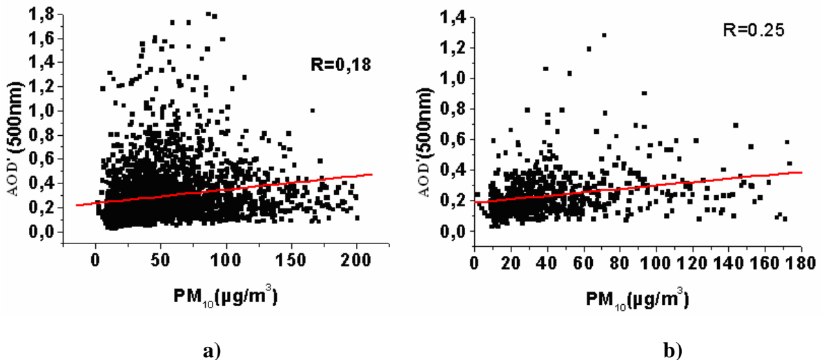
Figura 4.7: Diagrama de dispersão entre AOD (500nm) e PM_{10} ( \mu\text{g}/\text{m}^3 ). a) série temporal completa, b) série temporal sem os meses de setembro e outubro e só com os horários entre 11 e 14 h.
