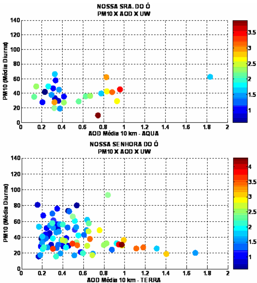
Figura 4.13 (c): Mesmo que na Figura 4.13 (a) para a Estação Nossa Senhora do Ó.
