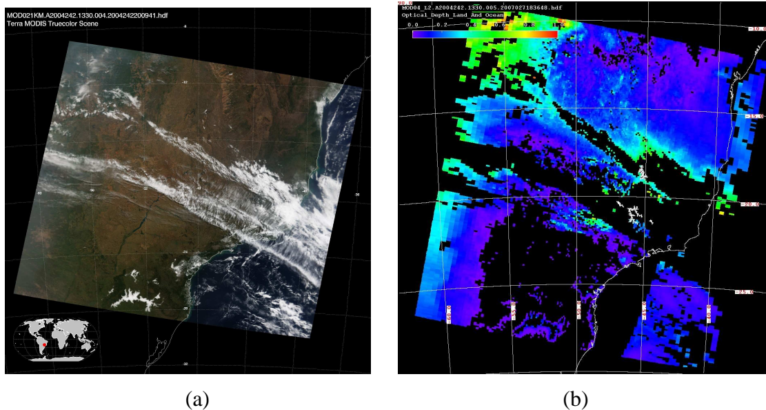
Figura 3.1: Imagem para o dia 242 do ano de 2004 do TERRA: a) Imagem do MODIS no visível, b) Produto de AOD 10 km do MODIS, c) Produto de AOD 10 km do MODIS na RMSP, d) Produto do Modelo Dinâmico na RMSP com resolução de 1,5 km x 1,5 km – Refletância Crítica, e) Produto do Modelo Dinâmico na RMSP com resolução de 1,5 km x 1,5 km – Modelo 3 de aerossol
