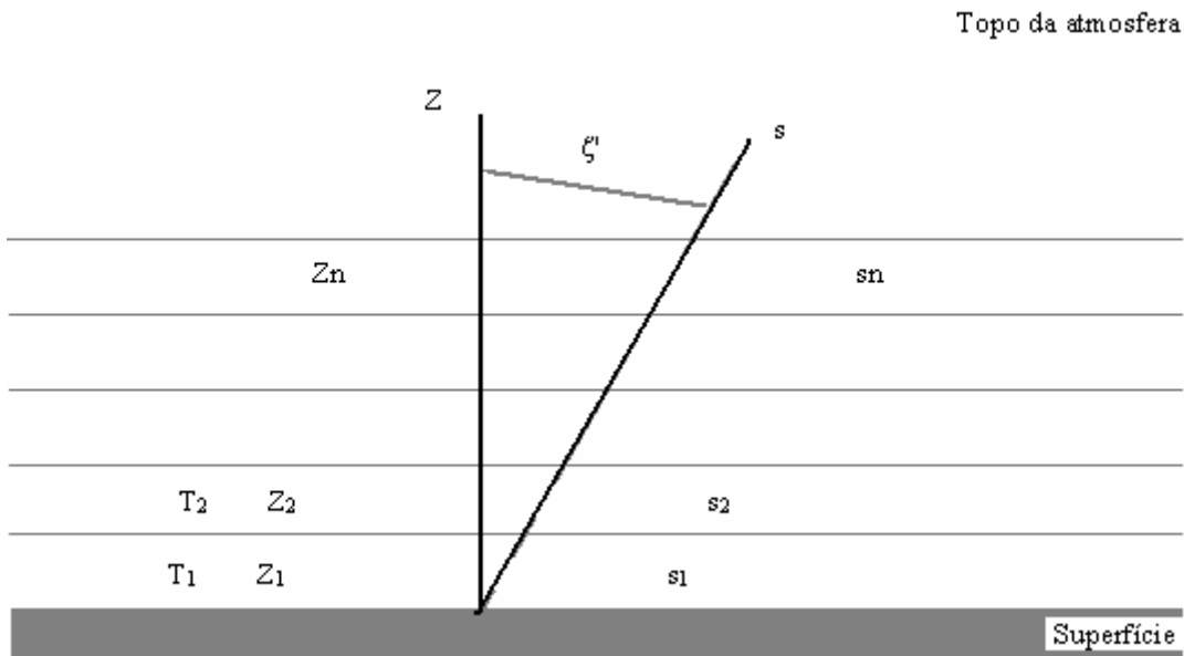
Figura 2.6: Atmosfera plano-paralela com camadas verticais e homogêneas horizontalmente.
