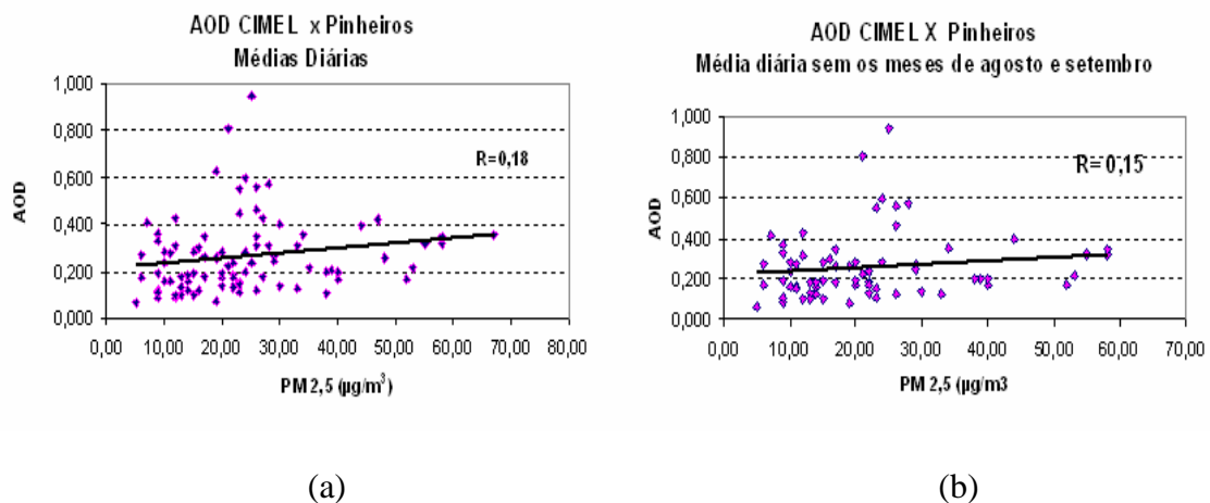
Figura 4.9: Diagrama de dispersão para as medidas de AOD-CIMEL e MP_{2,5} . Em (a) série temporal completa e em (b) excluindo-se os meses de agosto e setembro.
