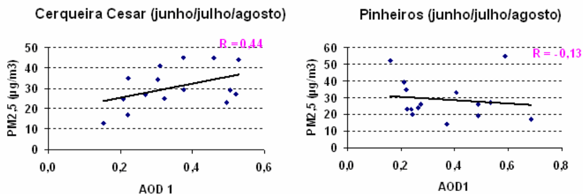
Figura 4.18: Diagramas de dispersão e correlações entre a concentração de material particulado fino MP_{2,5} ( \mu\text{g}/\text{m}^3 ) e a AOD1 para os meses de junho, julho e agosto.
