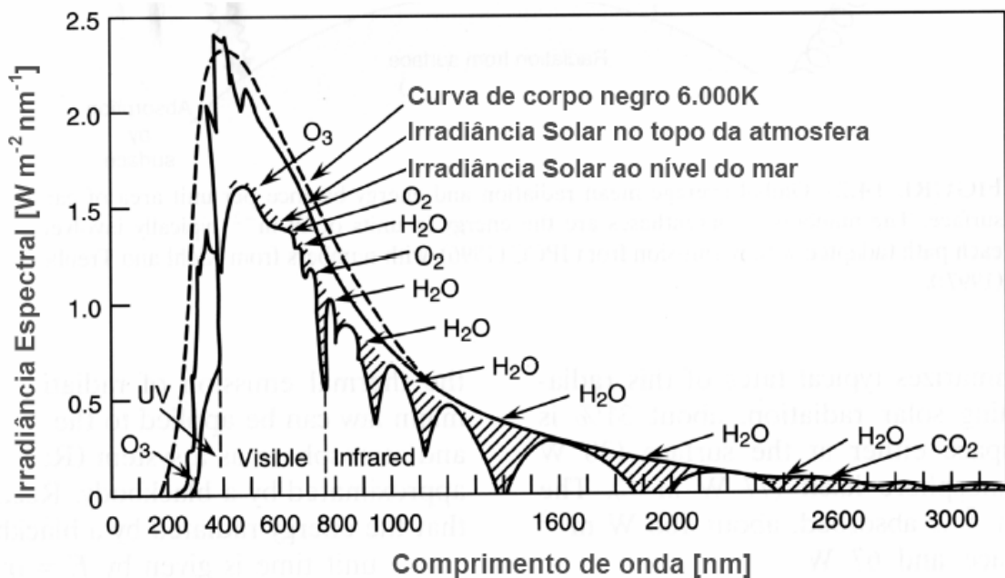
Figura 2.5: Espectro da Irradiância solar no topo da atmosfera e ao nível do mar. A linha tracejada representa a curva de um corpo negro a 6000 K e as regiões hachuradas indicam as regiões de absorção da radiação pelos constituintes da atmosfera (Figura adaptada de SEINFELD & PANDIS, 1998).
