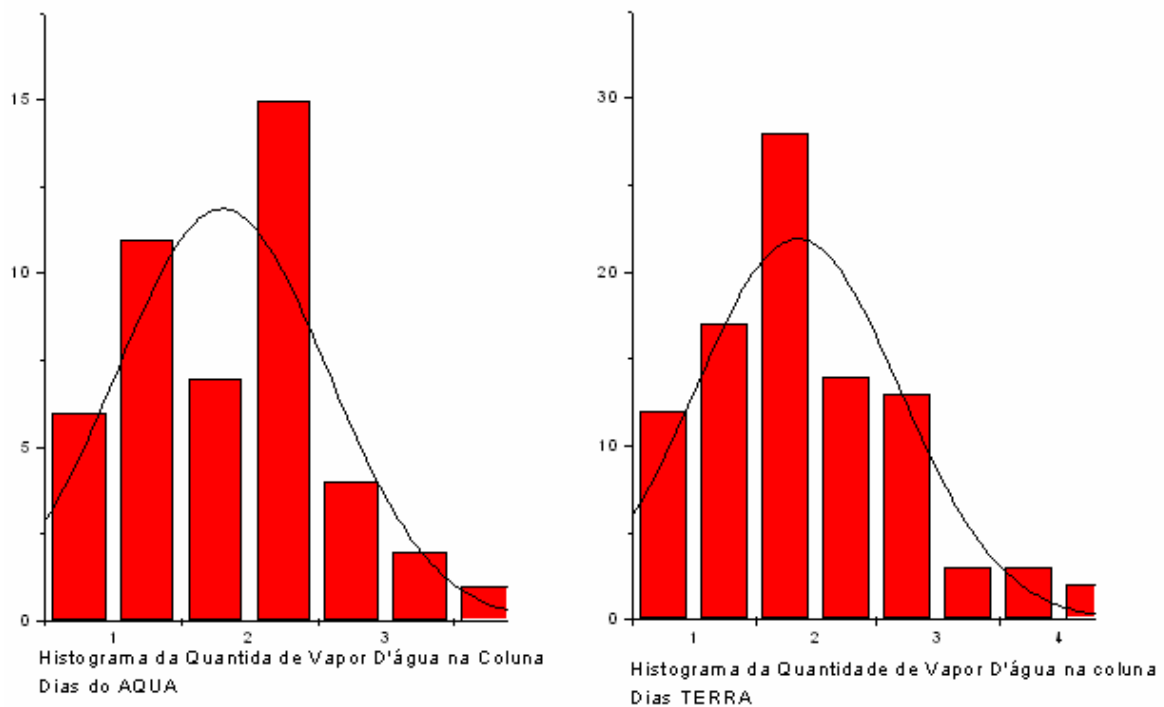
Figura 4.14: Histograma da distribuição de pontos em função das medidas de quantidade de vapor d'água na coluna, à esquerda a distribuição do pontos do AQUA e a direita do TERRA.
