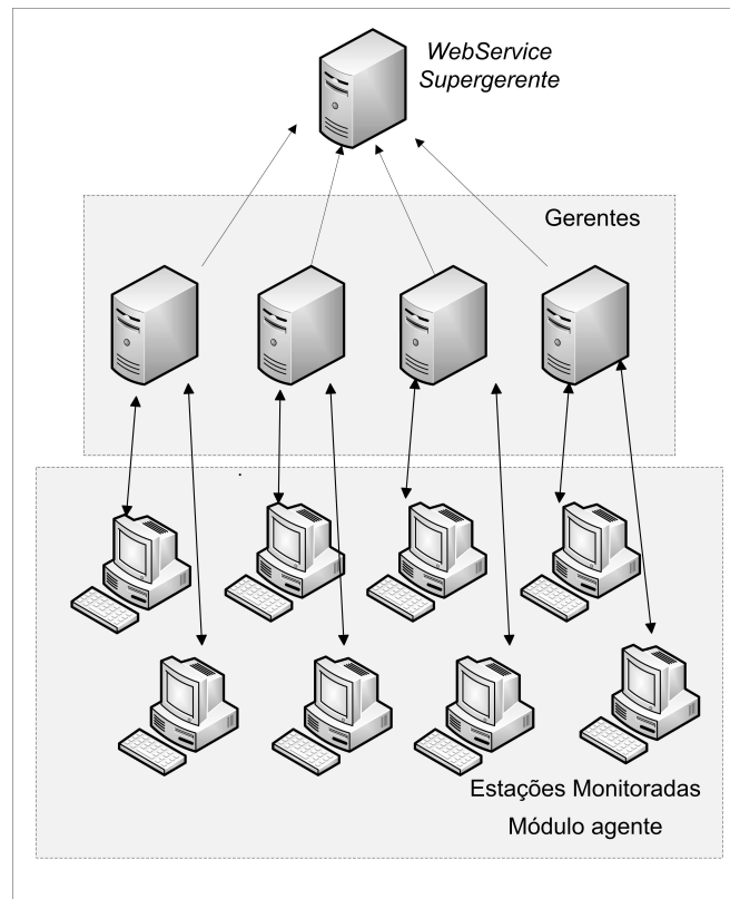
Figura 4.5: Diagrama de infra-estrutura do CACIC
