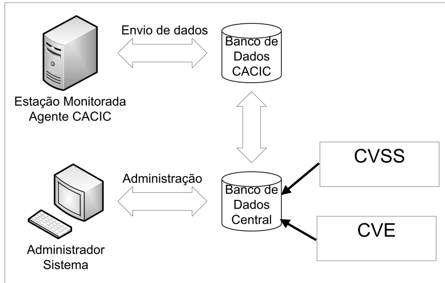
Figura 7.4: Visão conexão e envio de dados
