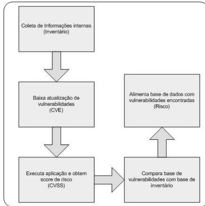
Figura 9.12: Procedimentos de coleta de informações
