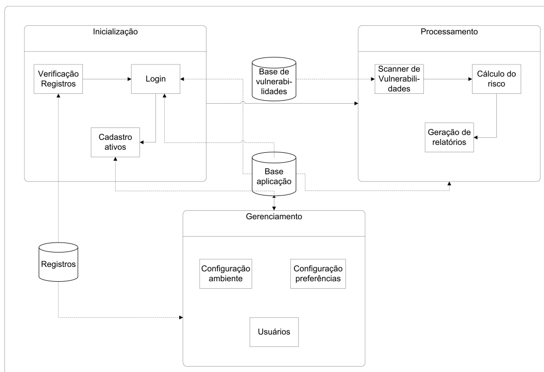
Figura 6.3: Estrutura do AGRIS
