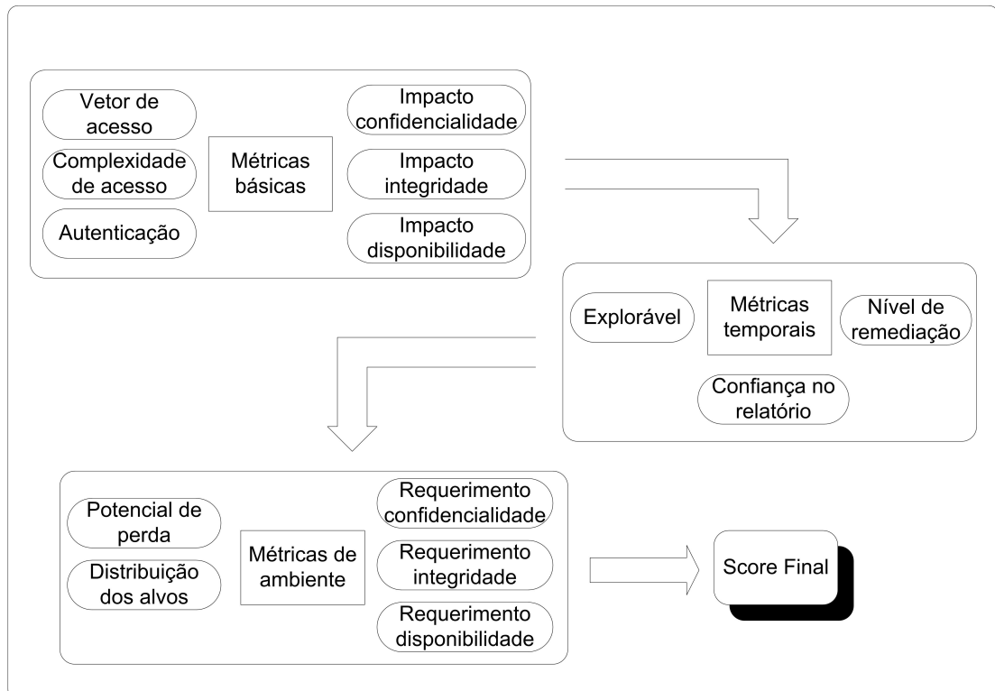
Figura 5.4: Organização do CVSS
