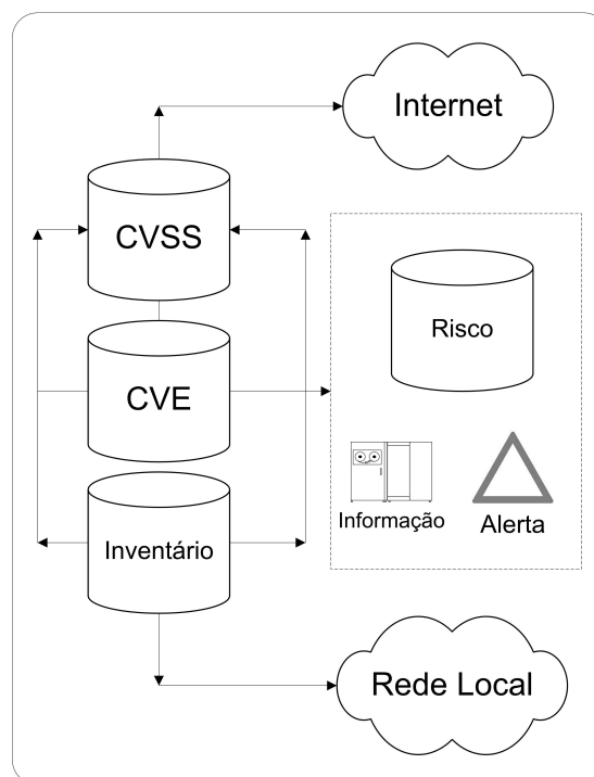
Figura 7.3: Modelagem de infra-estrutura de risco
