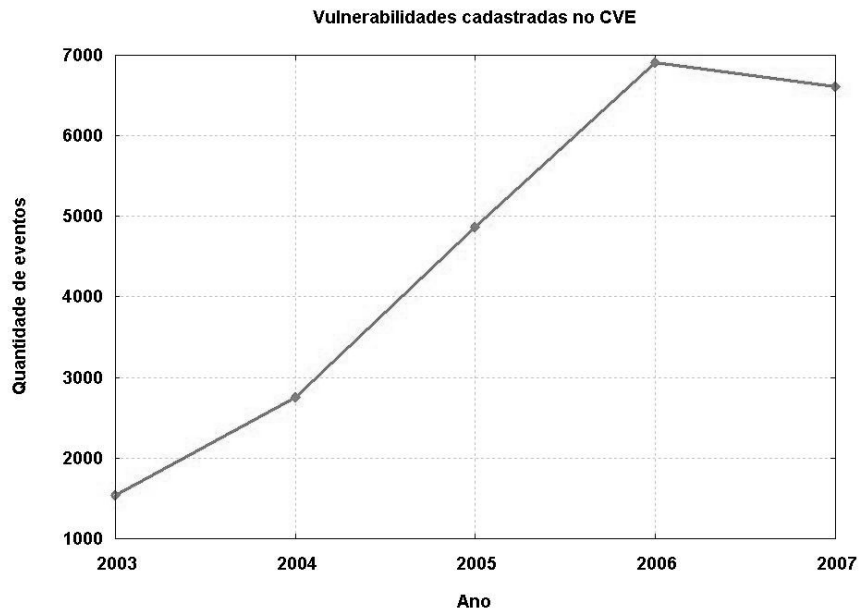
Figura 5.3: Vulnerabilidades cadastradas pelo CVE
