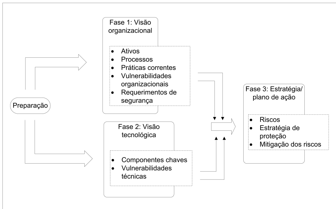
Figura 6.1: Processos do OCTAVE
