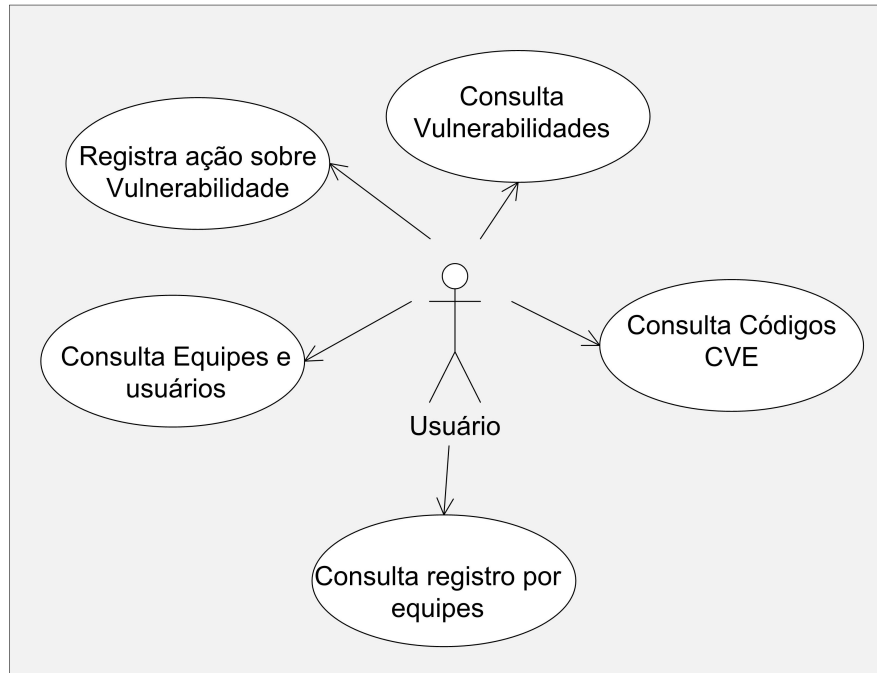
Figura 7.2: Diagrama de caso de uso - Usuário
