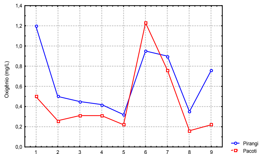
Figura 07 - Teor de oxigênio dissolvido (mg/L) da água de percolação nos bancos areno-lamoso dos estuários dos rios Pacoti e Pirangi - CE observados durante o período de estudo.
