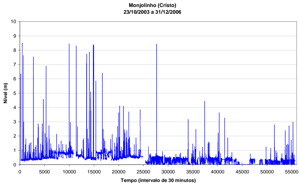
Figura A9 – Níveis hidrométricos ocorridos entre 23/10/2003 e 31/12/2006, registrados na bacia do córrego Monjolinho (Av. Tancredo Neves, próximo à rotatória do shopping Iguatemi).
