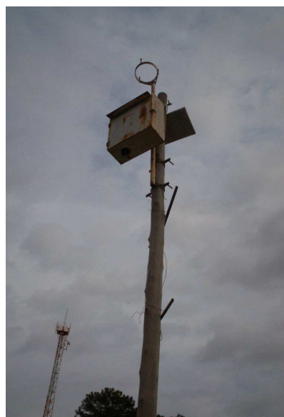
Figura 22: Detalhe do posto (Monjolinho – Casa Branca), hoje desativado. (Foto: TFS, 01/11/2007)
