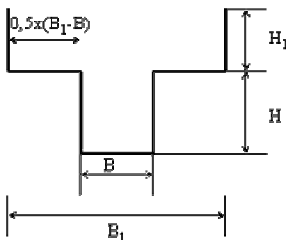
Figura 11: Seção transversal composta (Miller e Cunge, 1975). Fonte: IPH-UFRGS, ALM/FEA/IMF-UFPel, DFIS-FURG (2004).
