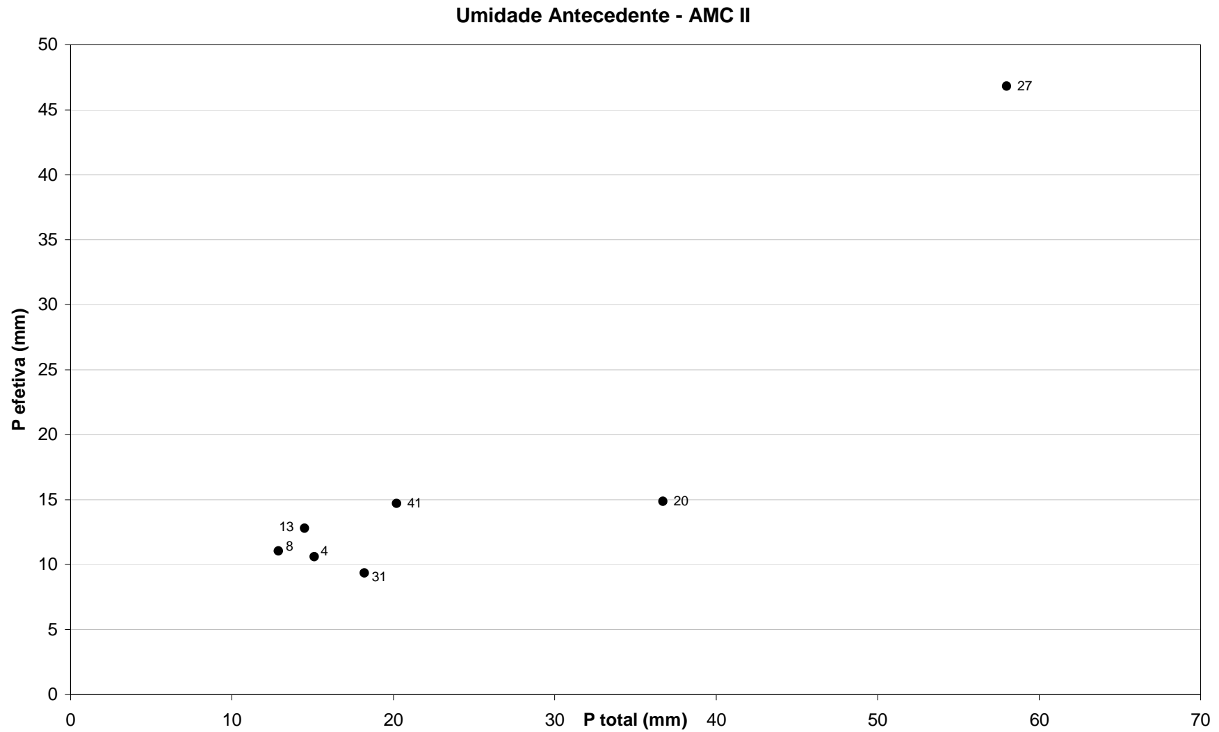
Figura C3 – Precipitação total versus precipitação efetiva para os eventos com condições de umidade antecedente II (os números ao lado de cada ponto correspondem ao número do evento).
