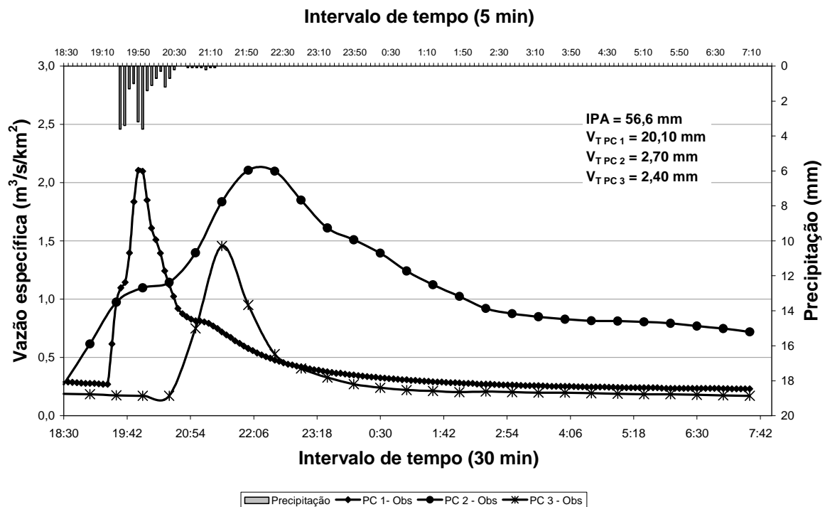
Figura 30: Precipitação observada (22,5 mm) e hidrogramas observados em função das vazões específicas e utilizados na fase de calibração. Dia: 09/01/2004, evento (b).
