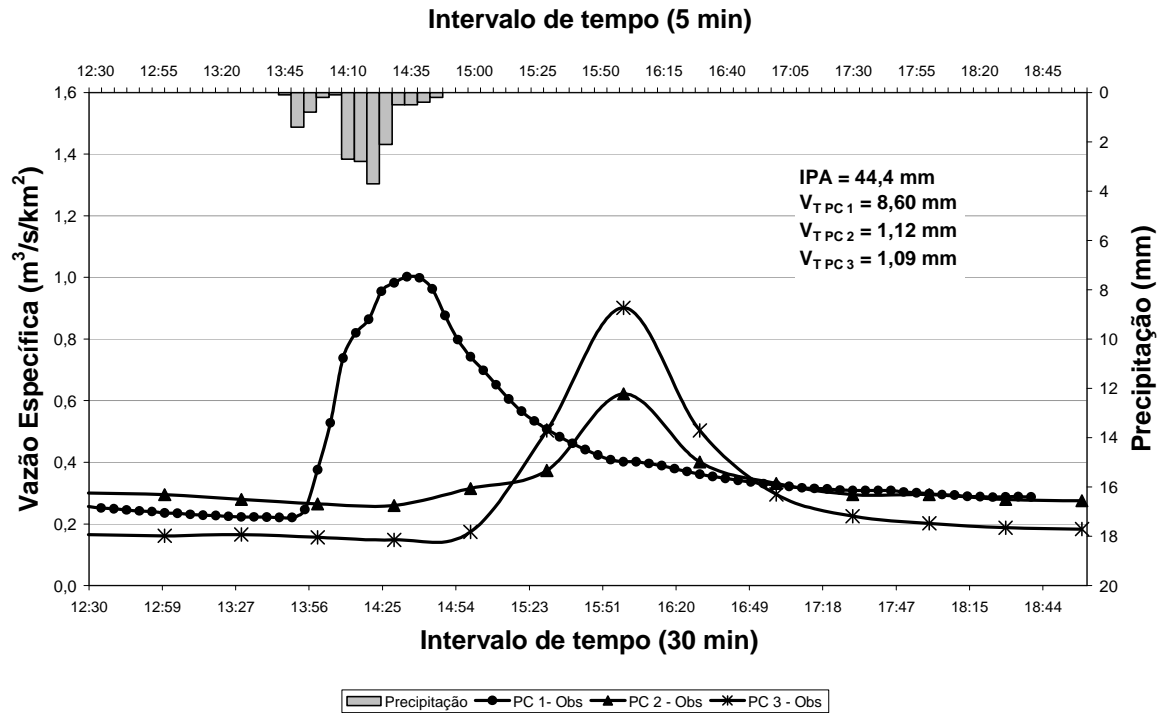
Figura 29: Precipitação observada (15,5 mm) e hidrogramas observados em função das vazões específicas e utilizados na fase de calibração. Dia: 09/01/2004, evento (a).
