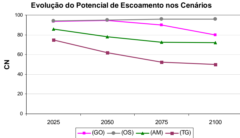
Figura 80: Evolução do parâmetro CN para os lotes urbanos.
