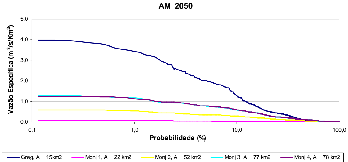
Figura 71: Curvas de permanência de cheias do cenário AM 2050.
