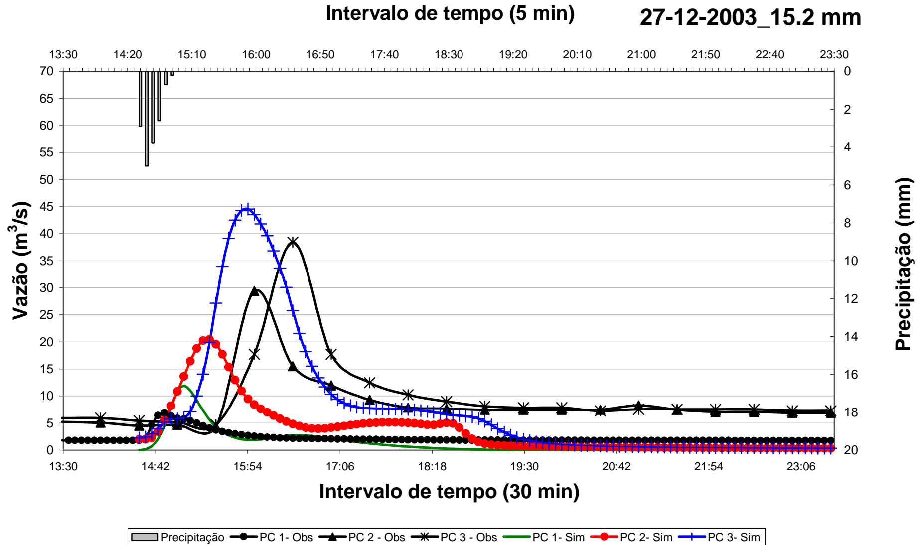
Figura 51: Gráfico das vazões simuladas e observadas nos três pontos de controle para efeitos de validação do modelo de simulação, relativo ao evento “e”.
