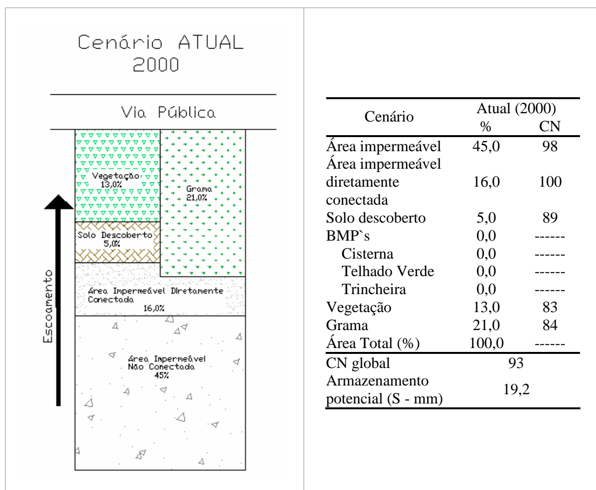
Figura 60: Características do lote de referência.
