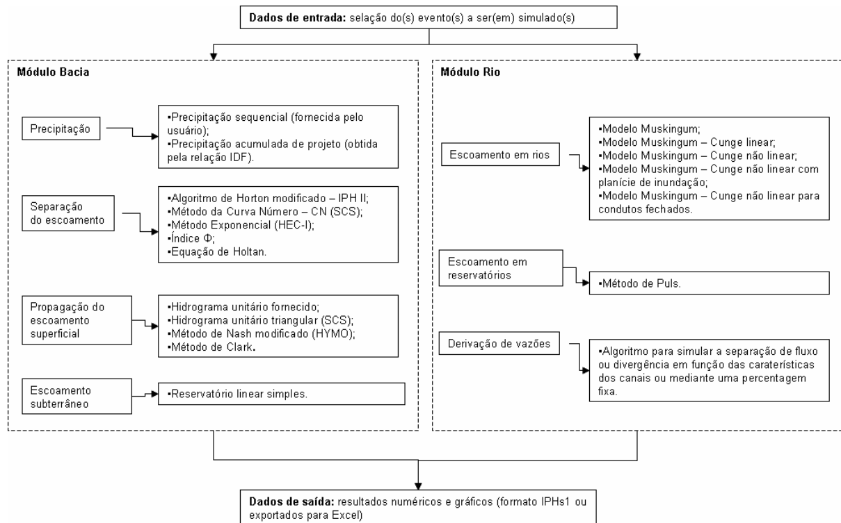
Figura 9: Configuração detalhada dos módulos bacia e rio com os métodos adotados.
