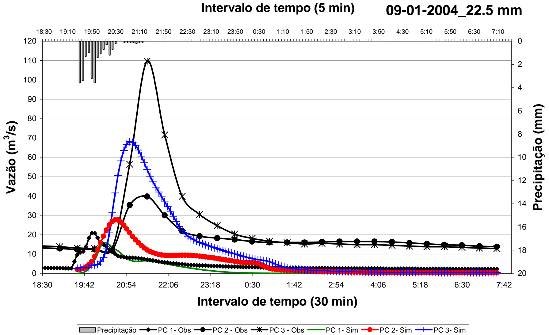
Figura 48: Gráfico das vazões simuladas e observadas nos três pontos de controle para efeitos de calibração do modelo de simulação, relativo ao evento “b”.
