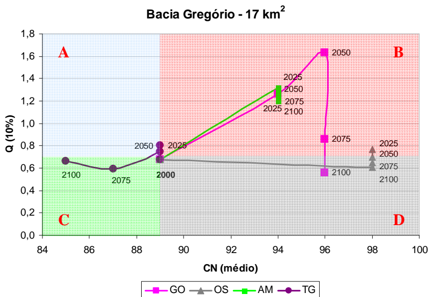
Figura 79: Avaliação dos benefícios e dos passivos de cada cenário para a bacia do Gregório.
