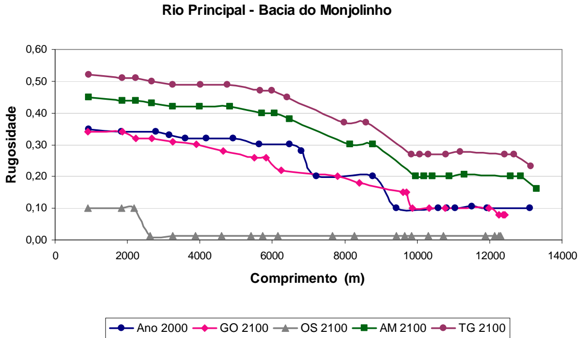
Figura 59: Rugosidade ao longo do principal rio da bacia do Monjolinho.
