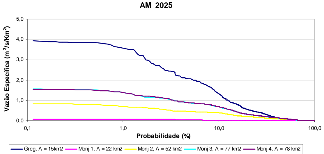
Figura 70: Curvas de permanência de cheias do cenário AM 2025.
