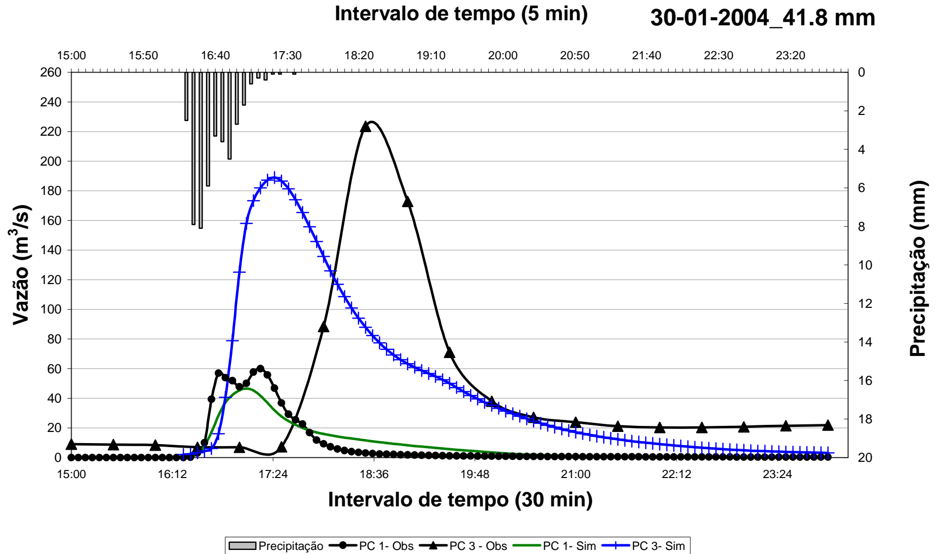
Figura 49 Gráfico das vazões simuladas e observadas nos três pontos de controle para efeitos de calibração do modelo de simulação, relativo ao evento “c”.
