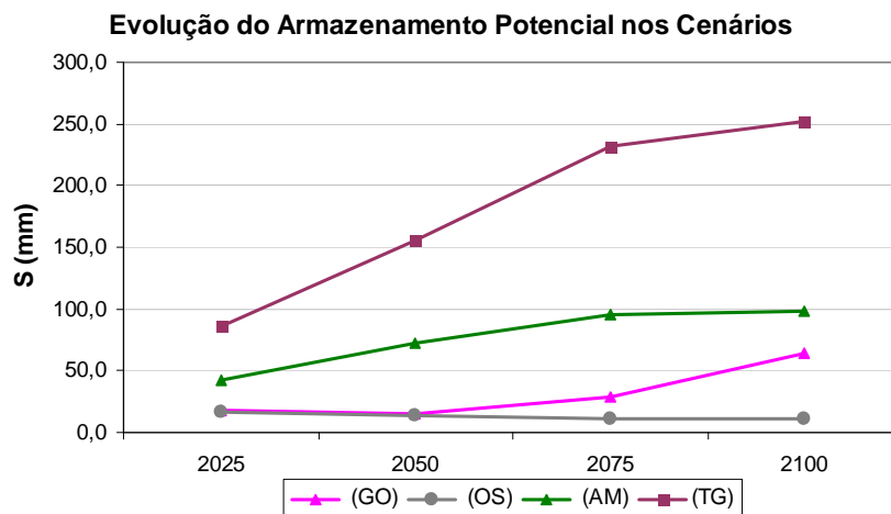
Figura 81: Evolução do armazenamento potencial de água no lote para os cenários.
