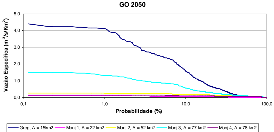
Figura 63: Curvas de permanência de cheias do cenário GO 2050.
