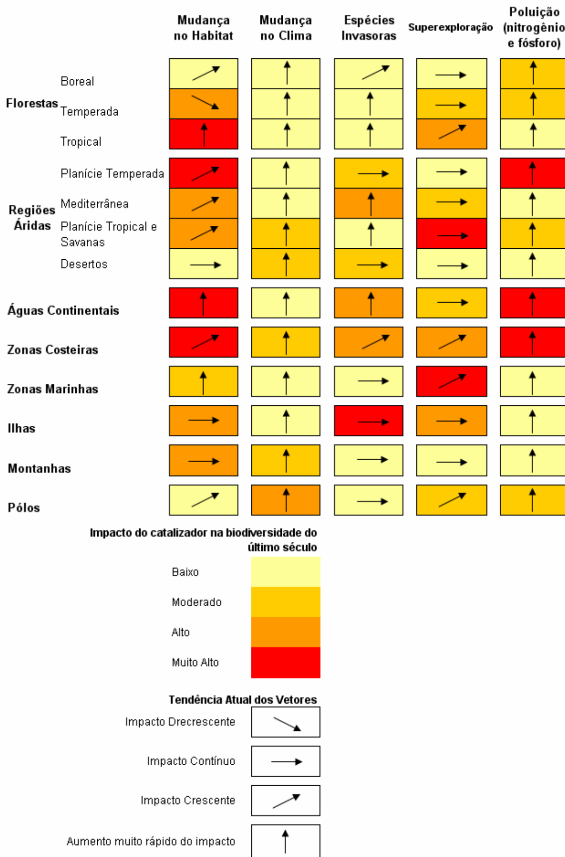
Figura 6: Avaliação dos principais vetores de mudança na biodiversidade e nos ecossistemas, e suas tendências.
