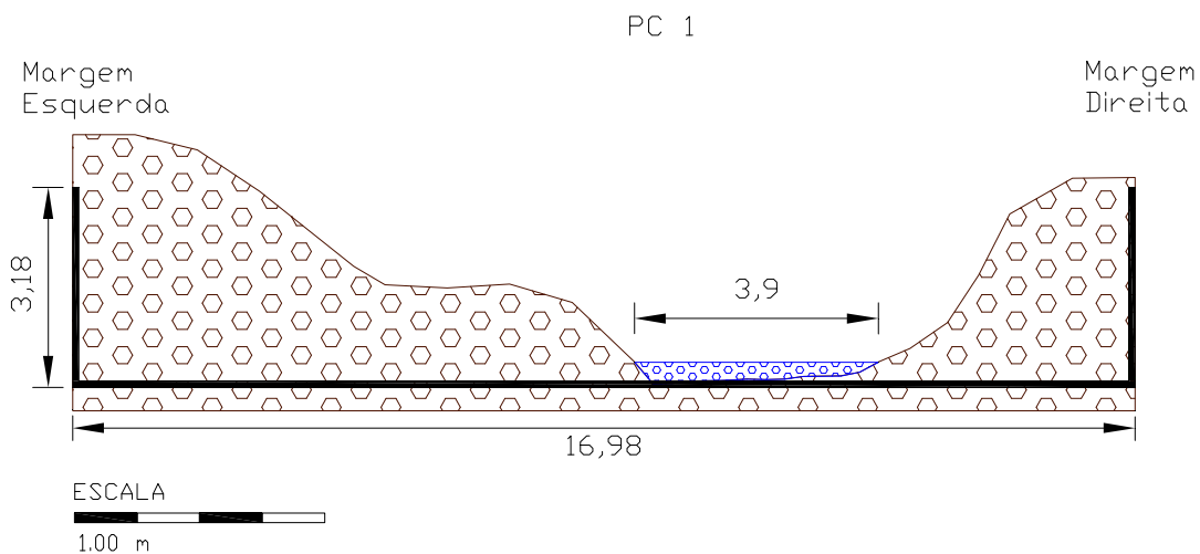
Figura 35: Seção transversal do ponto de controle 1 (PC 1), bacia do Córrego Gregório.
