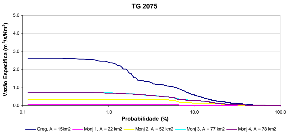
Figura 76: Curvas de permanência de cheias do cenário TG 2075.
