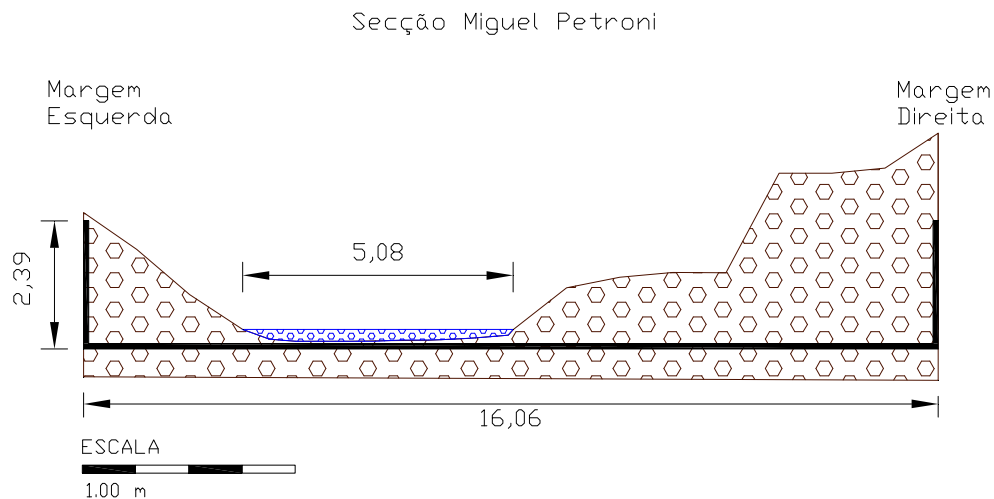
Figura 34: Seção transversal, rotatória na Rua Miguel Petroni.
