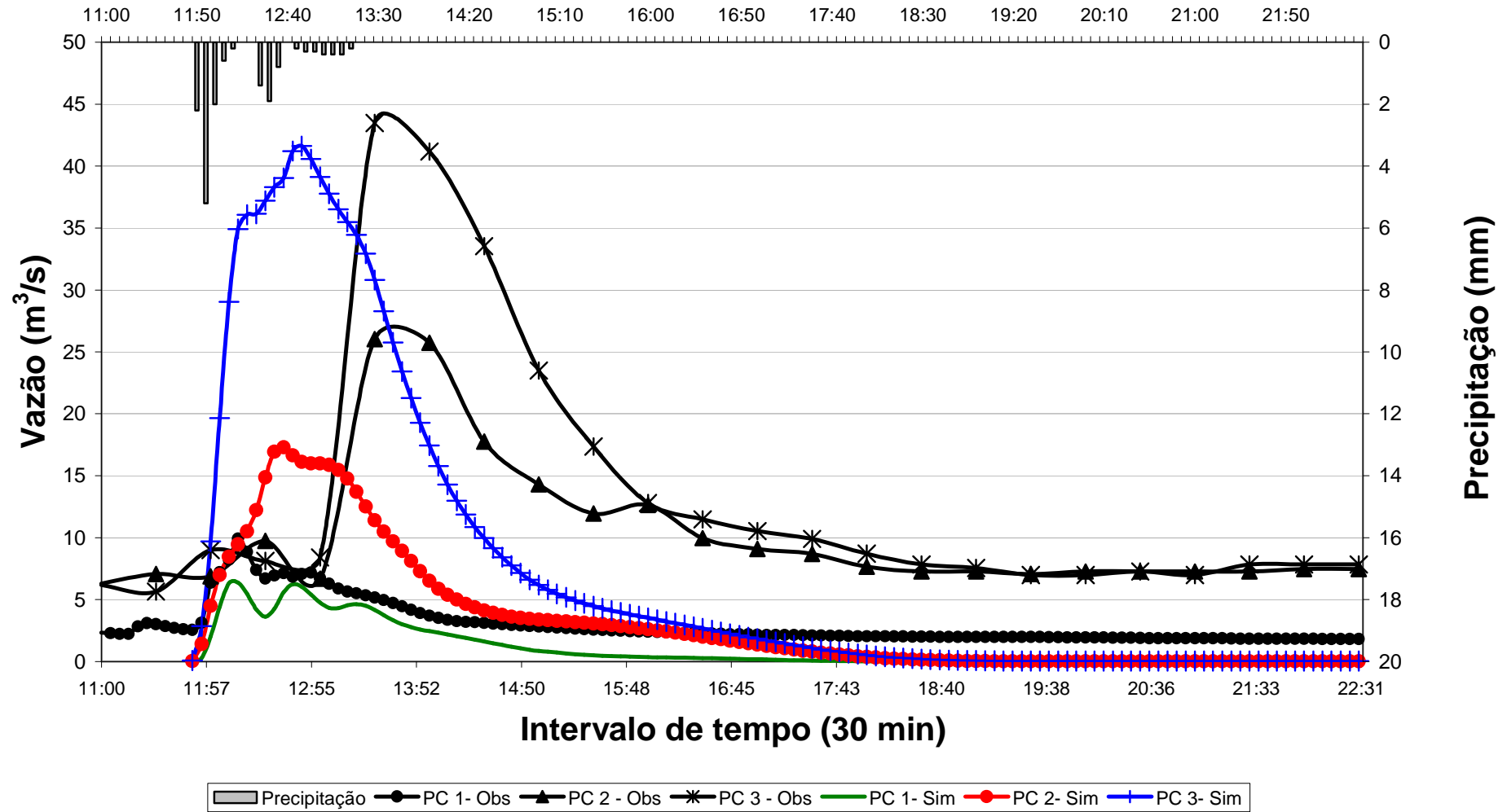
Figura 52: Gráfico das vazões simuladas e observadas nos três pontos de controle para efeitos de validação do modelo de simulação, relativo ao evento "F".
