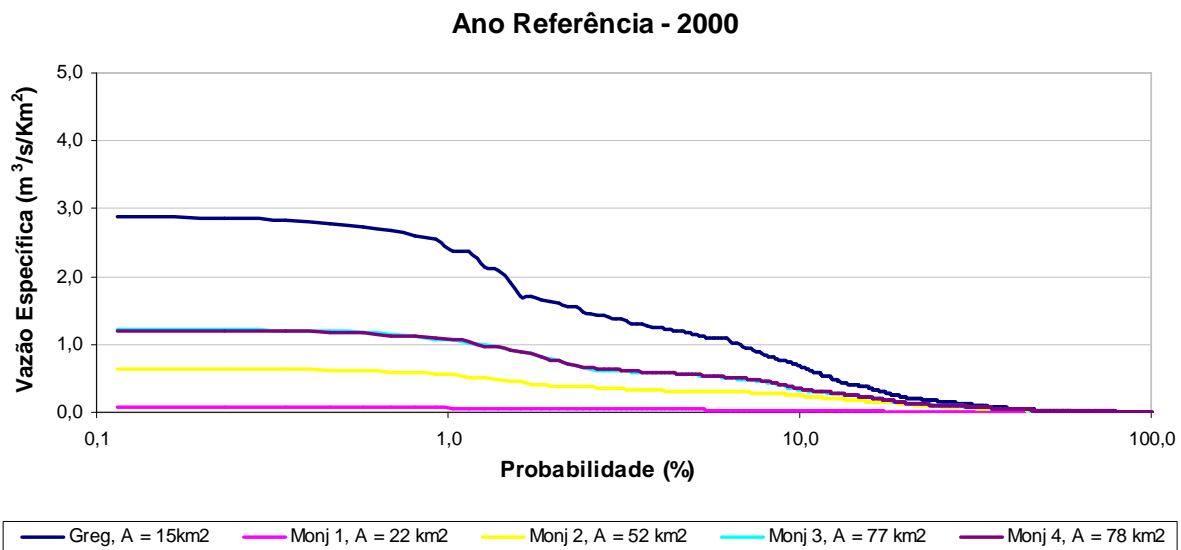
Figura 61: Curva de permanência de cheias para o ano de referência (2000).
