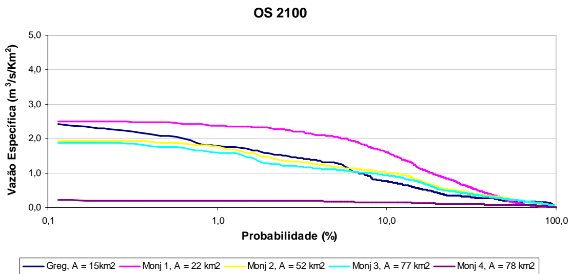
Figura 69: Curvas de permanência de cheias do cenário OS 2100.
