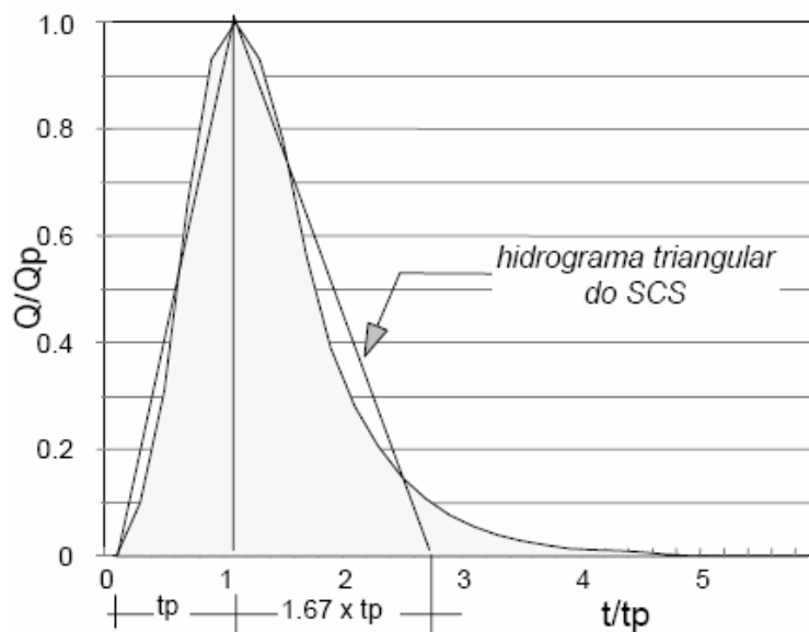
Figura 10: Hidrograma Unitário Triangular do SCS. Fonte: IPH-UFRGS, ALM/FEA/IMF-UFPel, DFIS-FURG (2004).
