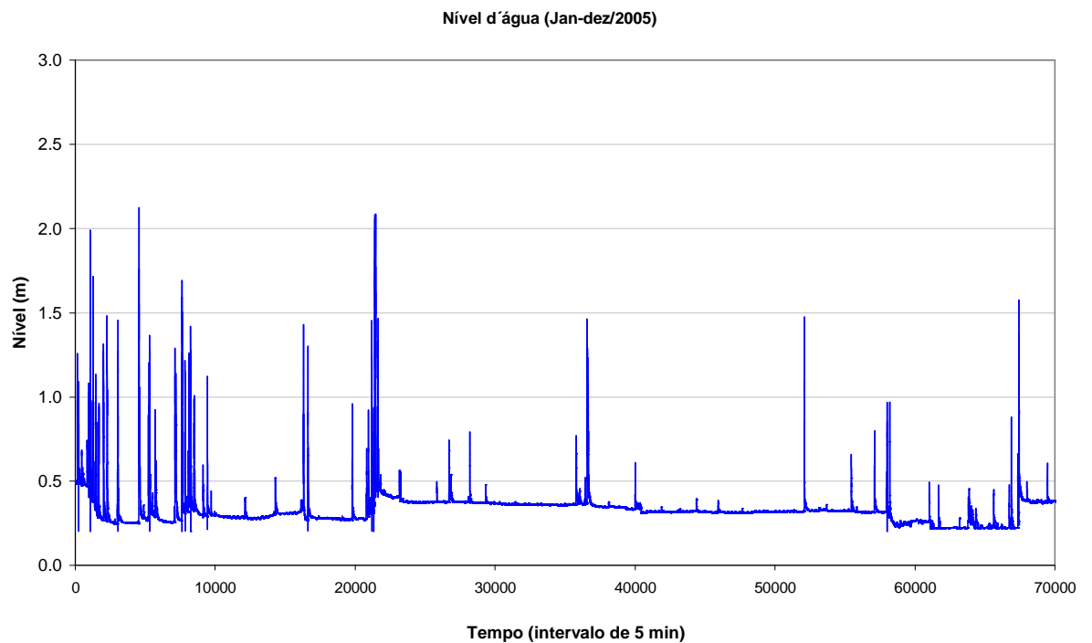
Figura A4 – Níveis hidrométricos ocorridos entre 01/01/2005 e 31/12/2005, registrados na bacia do córrego Gregório.
