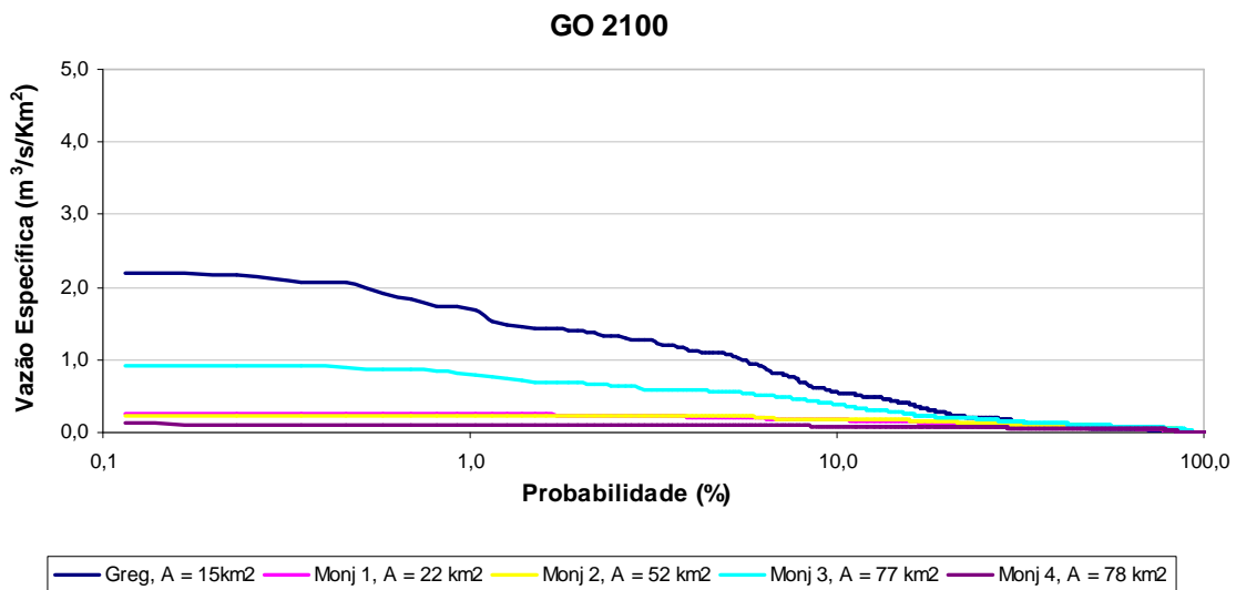
Figura 65: Curvas de permanência de cheias do cenário GO 2100.
