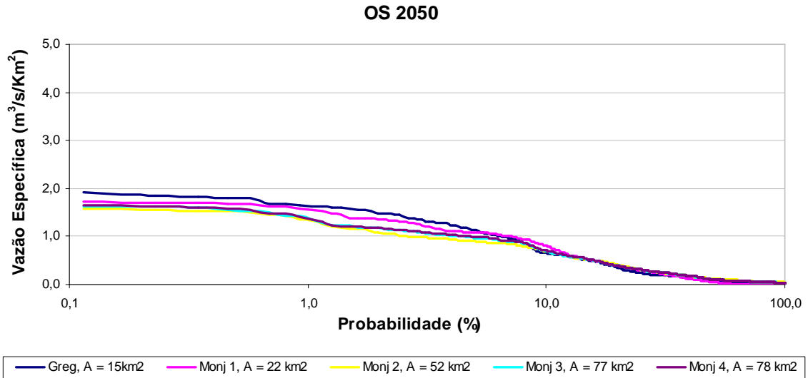
Figura 67: Curvas de permanência de cheias do cenário OS 2050.
