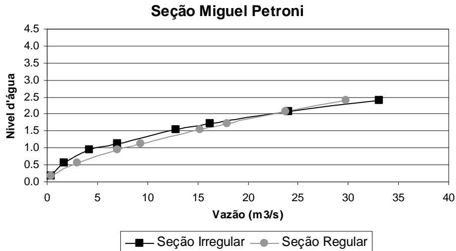
Figura 38: Estimativa da seção fictícia a partir da seção real da Rua Miguel Petroni, Bacia Monjolinho.
