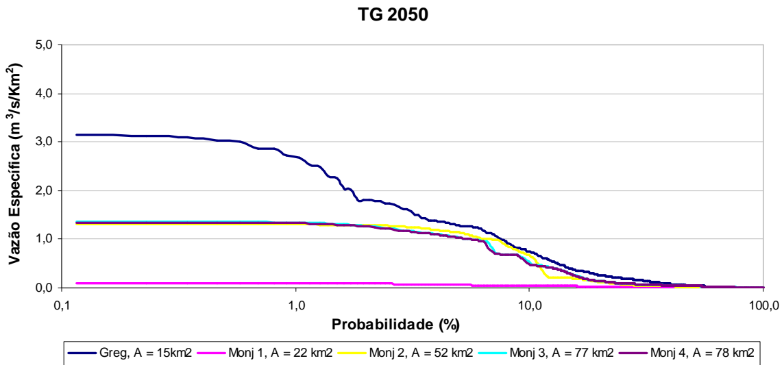
Figura 75: Curvas de permanência de cheias do cenário TG 2050.
