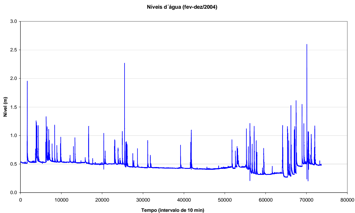
Figura A2 – Níveis hidrométricos ocorridos entre 01/02/2004 e 31/12/2004, registrados na bacia do córrego Gregório.
