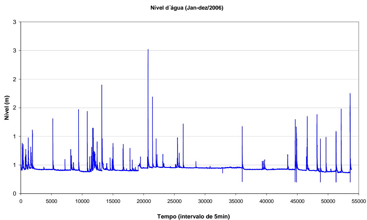
Figura A6 – Níveis hidrométricos ocorridos entre 01/01/2006 e 05/12/2006, registrados na bacia do córrego Gregório.
