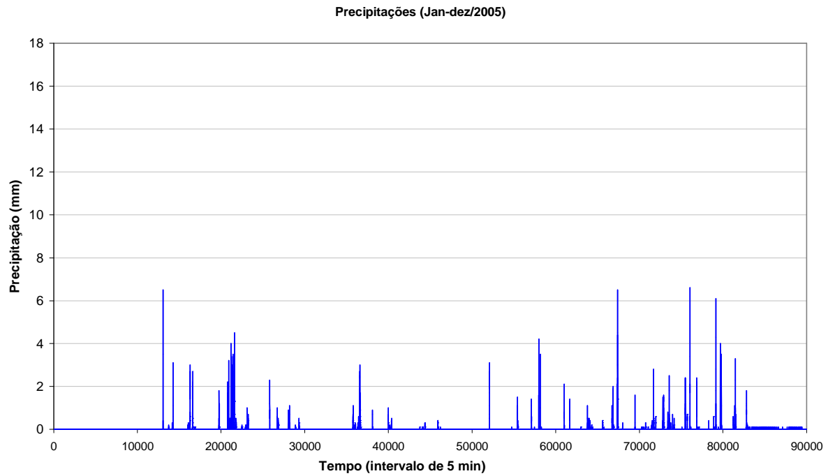
Figura A3 – Precipitações ocorridas entre 01/01/2005 e 31/12/2005, registradas na bacia do córrego Gregório.
