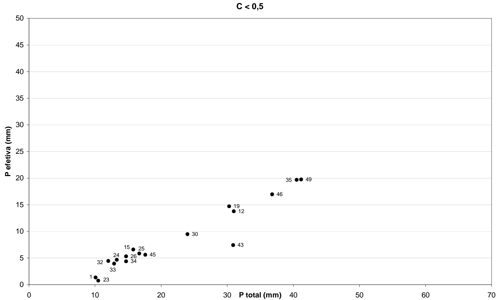
Figura C5 – Precipitação total versus precipitação efetiva para os eventos com coeficiente de escoamento superficial inferior a 0,50 (os números ao lado de cada ponto correspondem ao número do evento).
