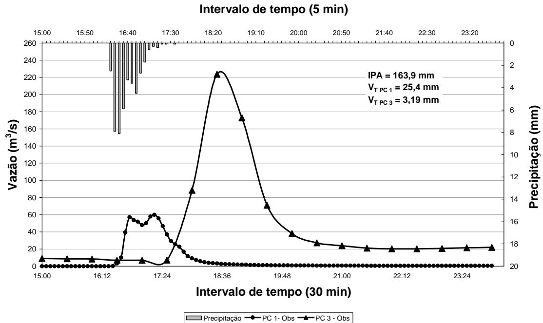
Figura 27: Precipitação observada (41,8 mm) e hidrogramas observados dados em função das vazões e utilizados na fase de calibração. Dia: 30/01/2004, evento (c).
