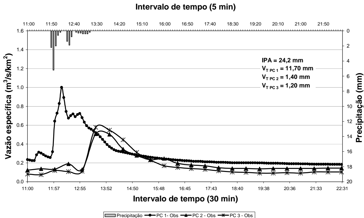
Figura 33: Precipitação observada (16,5 mm) e hidrogramas observados em função das vazões específicas e utilizados na fase de validação. Dia: 31/12/2003, evento (f).
