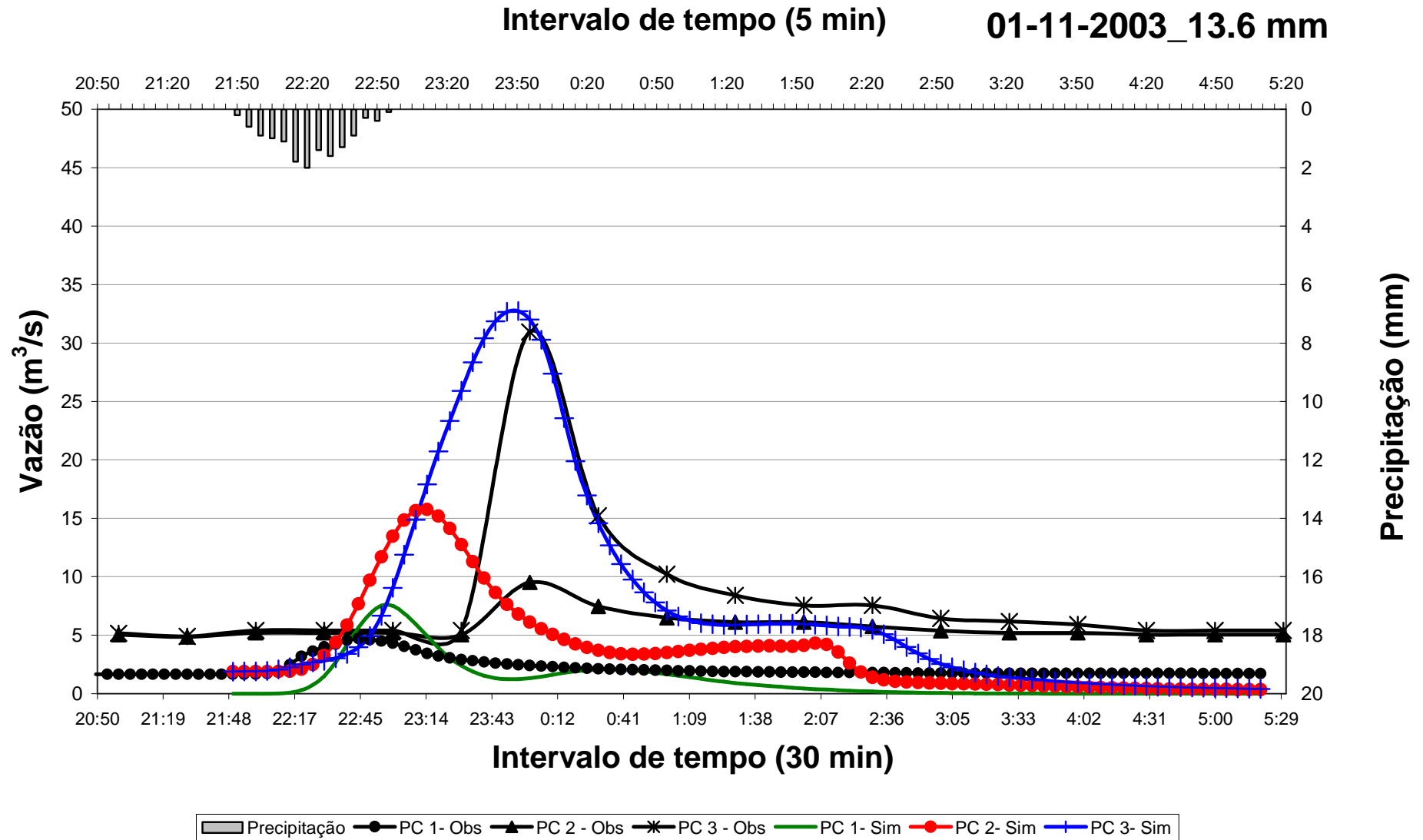
Figura 50: Gráfico das vazões simuladas e observadas nos três pontos de controle para efeitos de validação do modelo de simulação, relativo ao evento “d”.
