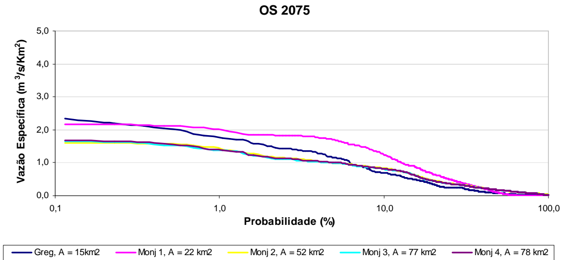
Figura 68: Curvas de permanência de cheias do cenário OS 2075.
