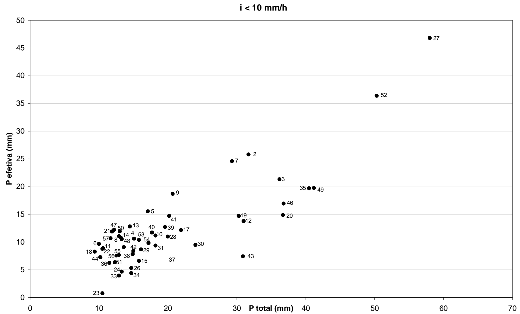
Figura C7 – Precipitação total versus precipitação efetiva para os eventos com intensidade média inferior à 10mm/h (os números ao lado de cada ponto correspondem ao número do evento).
