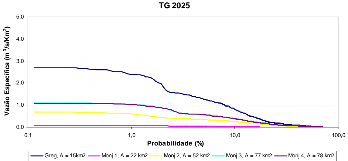
Figura 74: Curvas de permanência de cheias do cenário TG 2025.
