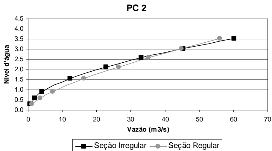
Figura 40: Estimativa da seção fictícia a partir da seção real do PC 2, Bacia Monjolinho (Casa Branca).
