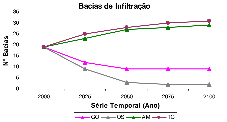
Figura 57: Utilização de bacias de infiltração nos cenários.
