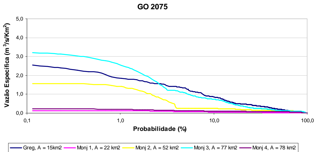
Figura 64: Curvas de permanência de cheias do cenário GO 2075.
