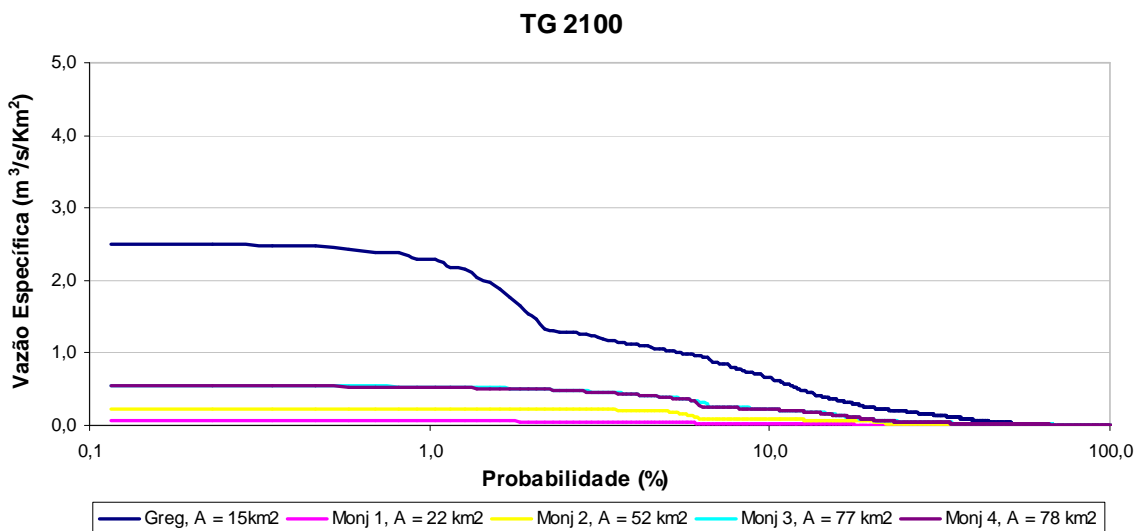
Figura 77: Curvas de permanência de cheias do cenário TG 2100.
