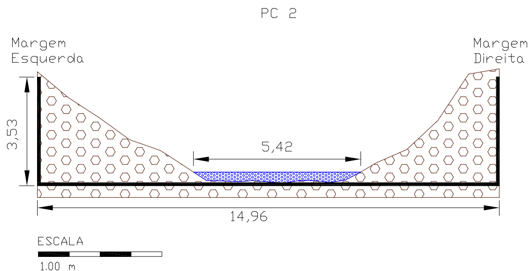
Figura 36: Seção transversal do ponto de controle 2 (PC 2), bacia do Córrego Monjolinho (Casa Branca).
