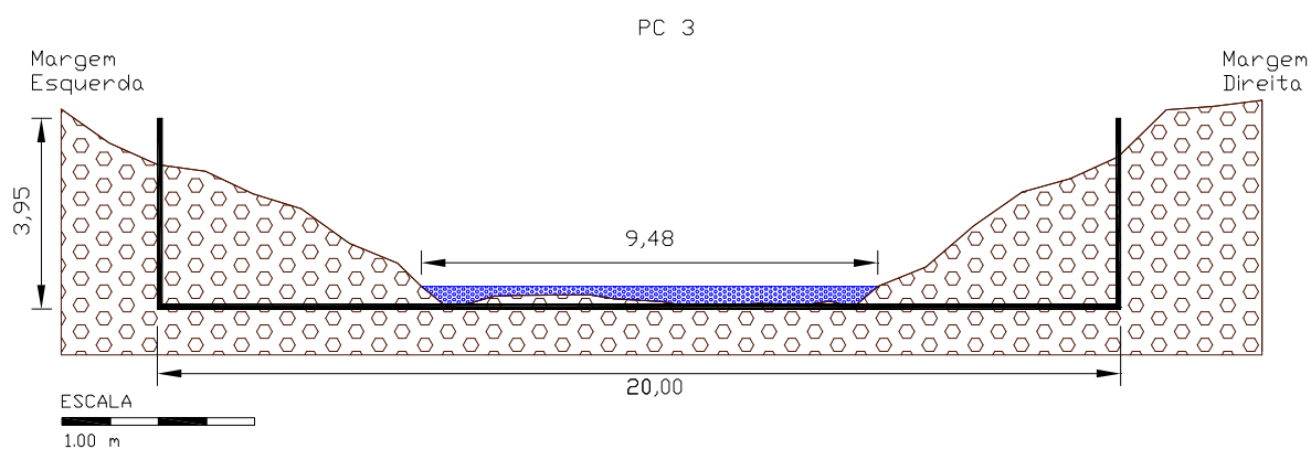
Figura 37: Seção transversal do ponto de controle 3 (PC 3), bacia do Córrego Monjolinho (Shopping Iguatemi).
