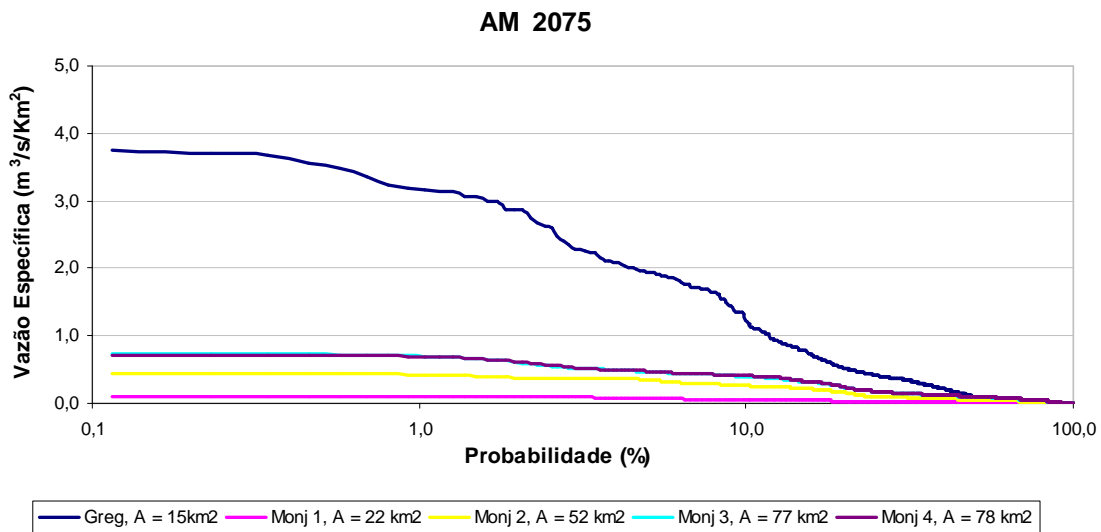
Figura 72: Curvas de permanência de cheias do cenário AM 2075.
