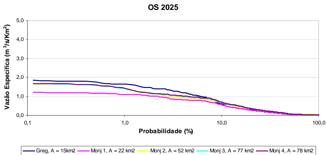
Figura 66: Curvas de permanência de cheias do cenário OS 2025.
