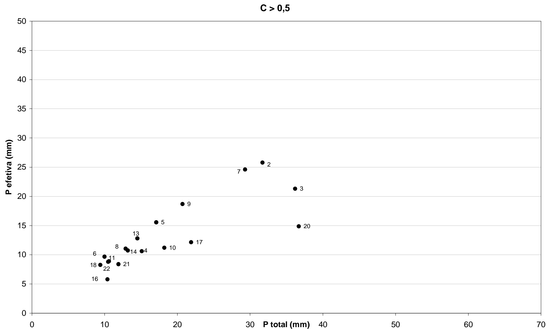
Figura C6 – Precipitação total versus precipitação efetiva para os eventos com coeficiente de escoamento superficial superior a 0,50 (os números ao lado de cada ponto correspondem ao número do evento).
