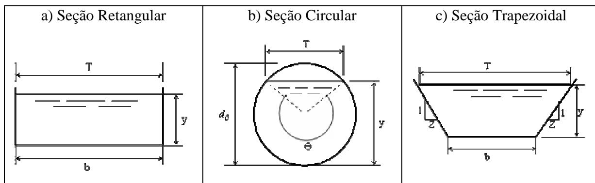
Figura 12: Tipos de seção.
