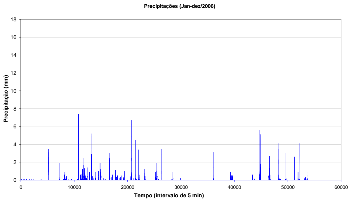
Figura A5 – Precipitações ocorridas entre 01/02/2006 e 05/12/2006, registradas na bacia do córrego Gregório.
