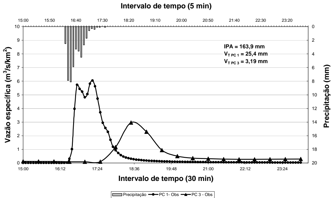
Figura 28: Precipitação observada (41,8 mm) e hidrogramas observados dados em função das vazões específicas e utilizados na fase de calibração. Dia: 30/01/2004, evento (c).
