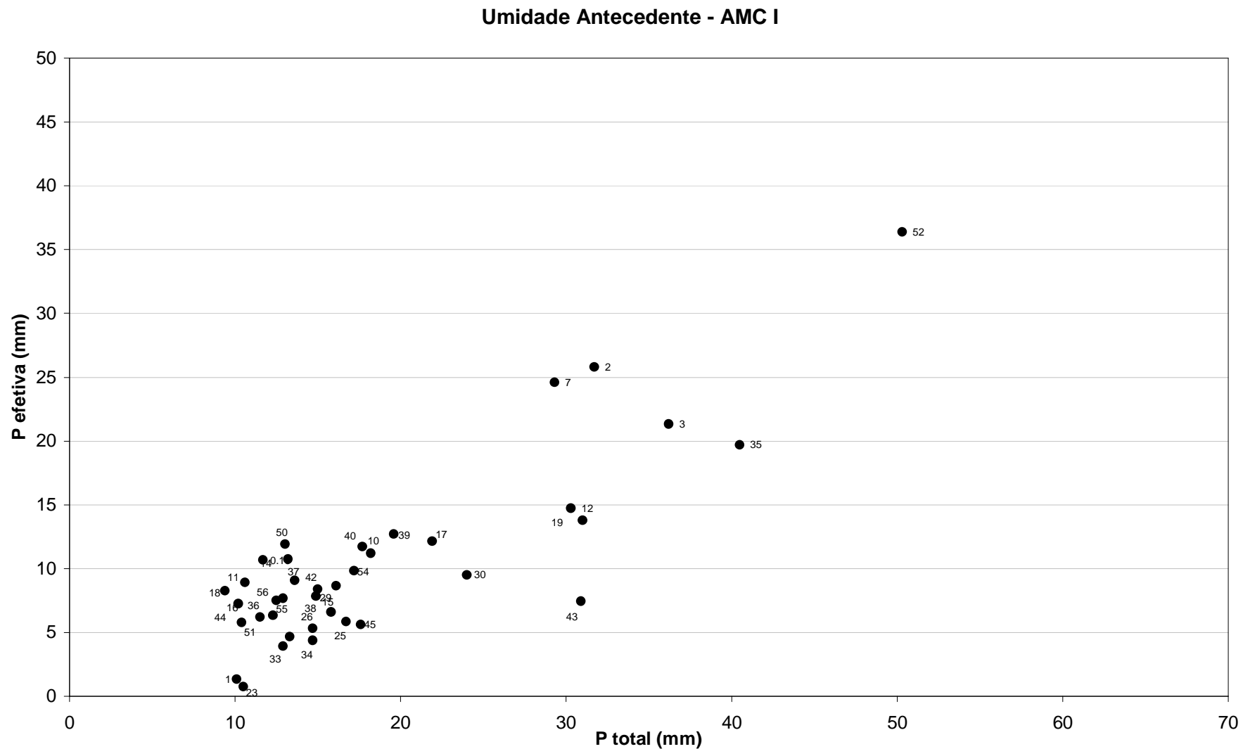
Figura C2 – Precipitação total versus precipitação efetiva para os eventos com condições de umidade antecedente I (os números ao lado de cada ponto correspondem ao número do evento).
