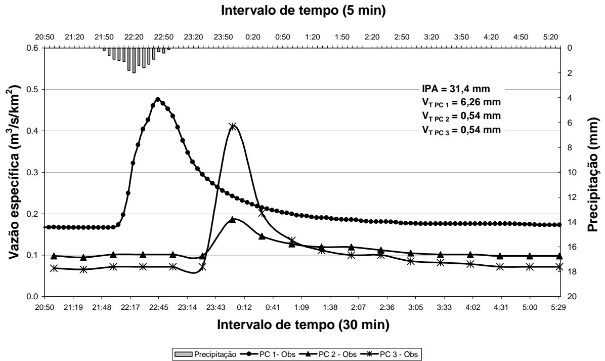
Figura 31: Precipitação observada (13,6 mm) e hidrogramas observados em função das vazões específicas e utilizados na fase de validação. Dia: 01/11/2003, evento (d).
