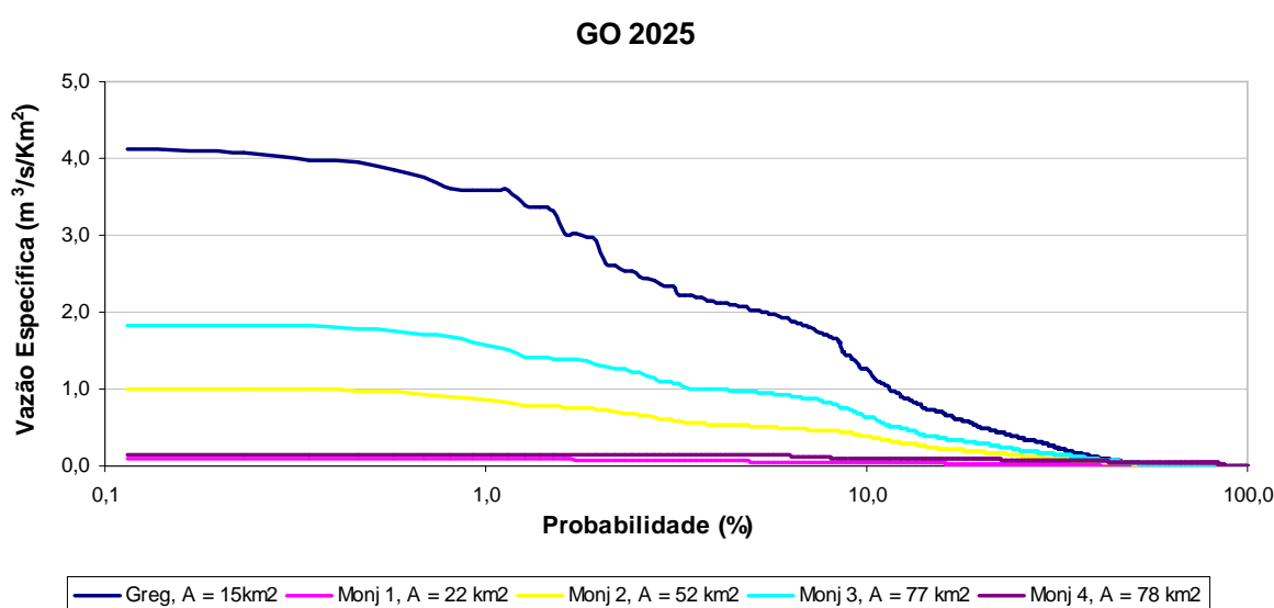
Figura 62: Curvas de permanência de cheias do cenário GO 2025.
