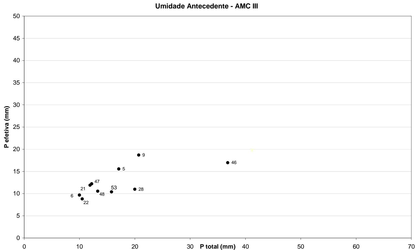
Figura C4 – Precipitação total versus precipitação efetiva para os eventos com condições de umidade antecedente III (os números ao lado de cada ponto correspondem ao número do evento).
