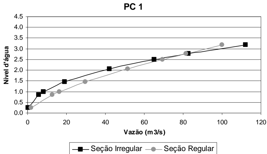
Figura 39: Estimativa da seção fictícia a partir da seção real do PC 1, Bacia do Gregório.
