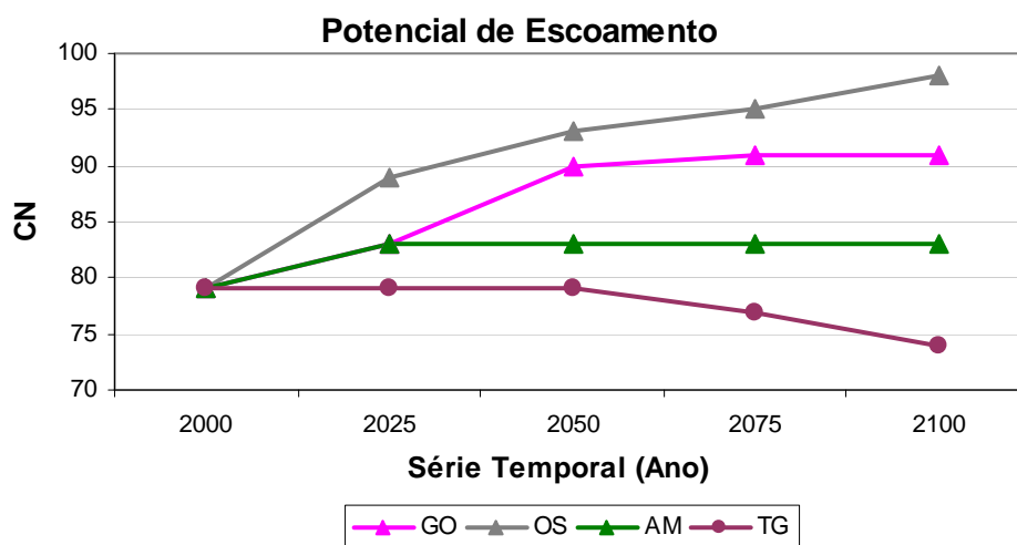
Figura 55: Evolução do potencial de escoamento nos cenários.
