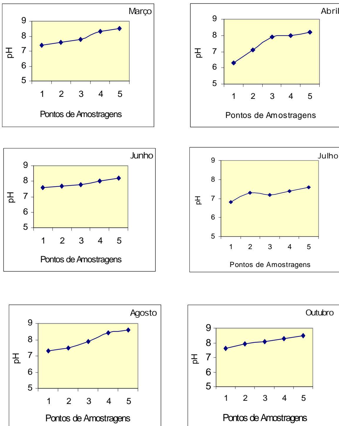
Figura 18. Distribuição do pH medido nas águas superficiais do estuário do rio Bacanga, Ilha de São Luís/MA.
