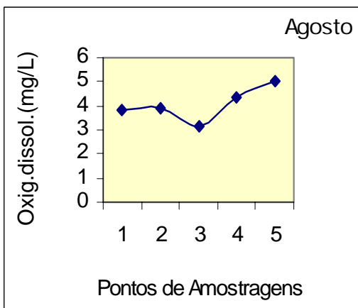
Figura 19. Distribuição espaço temporal do oxigênio dissolvido medido nas águas superficiais do estuário do rio Bacanga, Ilha de São Luís/MA.
