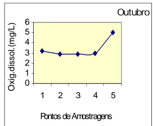
Figura 19. Distribuição espaço temporal do oxigênio dissolvido medido nas águas superficiais do estuário do rio Bacanga, Ilha de São Luís/MA.
