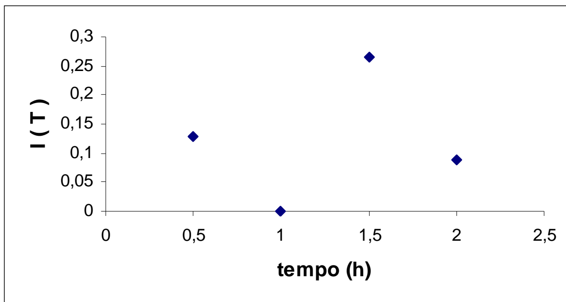
Figura 5. Coeficiente de correlação de informação em função do tempo de defasagem para a direção dos ventos no período chuvoso (Fev/02)
