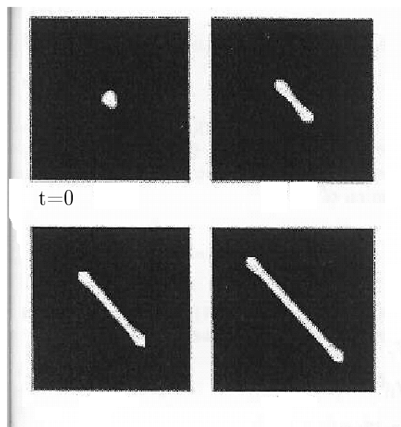
Figura 4.9: Evolução no tempo da solução u^\varepsilon(x, t) de (0.7) com \varepsilon = 0.05 , \alpha = 1.0 , \gamma = 1.0 , h(v) = a \exp(-bv) , a = 20\sqrt{2} e b = 6.41 .
