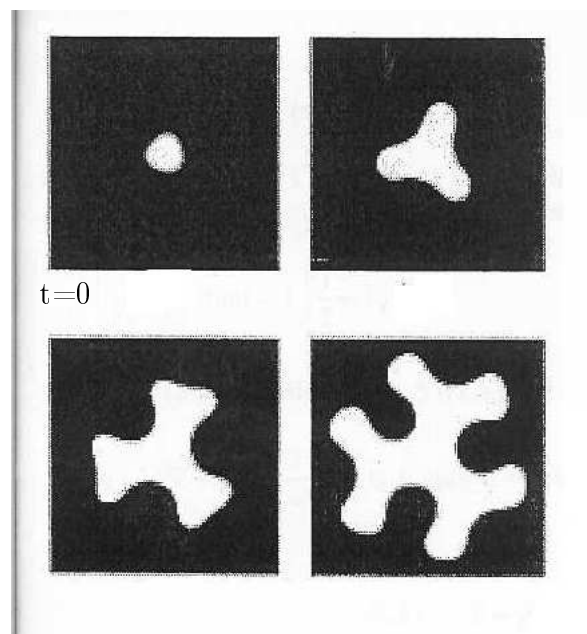
Figura 4.10: Evolução no tempo da solução u^\varepsilon(x, t) de (0.7) com \varepsilon = 0.05 , \alpha = 1.0 , \gamma = 0.5 , h(v) = a \exp(-bv) , a = 20\sqrt{2} e b = 17.55 .
