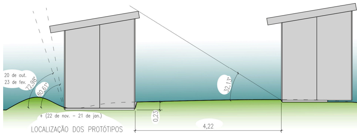
Figura 38 – Sugestão para localização, evitando sombreamento dos protótipos
