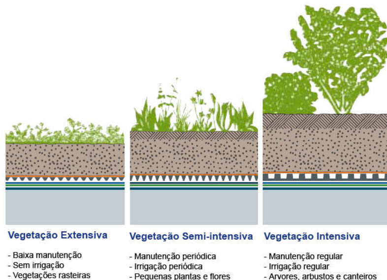
Figura 19 – Comparação entre as classificações de coberturas vegetais e considerações a respeito delas (Adaptação: ZinCo, 2007)
