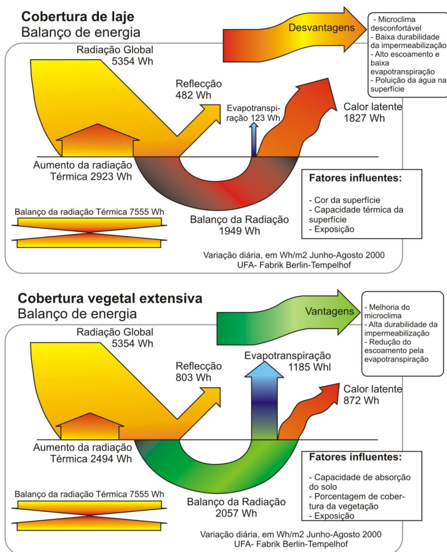
Figura 26 – Diferença de fluxo de calor entre uma laje e uma cobertura vegetal (SCHMIDT, 2002)
