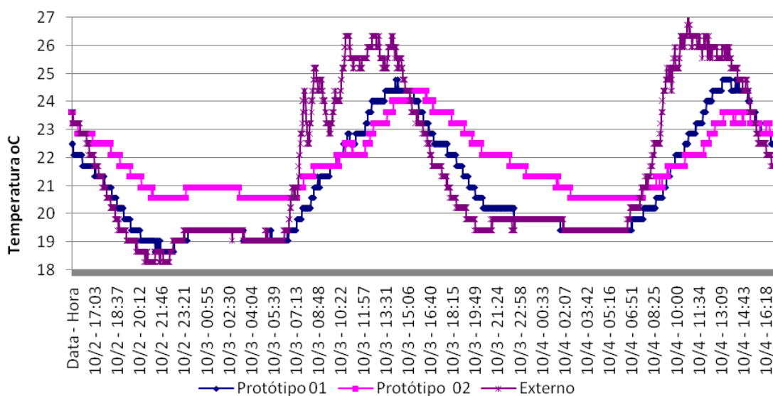
Gráfico 10 - Medições comparativas de temperaturas entre a laje e a cobertura vegetal
