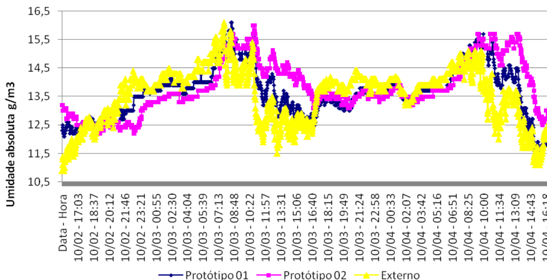
Gráfico 11 - Medições comparativas de umidade absoluta entre a laje e a cobertura vegetal
