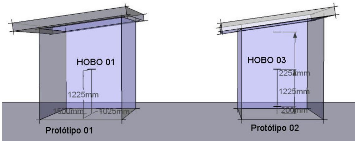
Figura 69 - Localização dos HOBOS® no interior do protótipo
