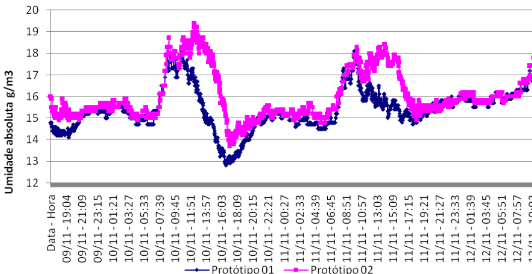
Gráfico 9 - Umidades absolutas obtidas pelos aparelhos nos dois protótipos
