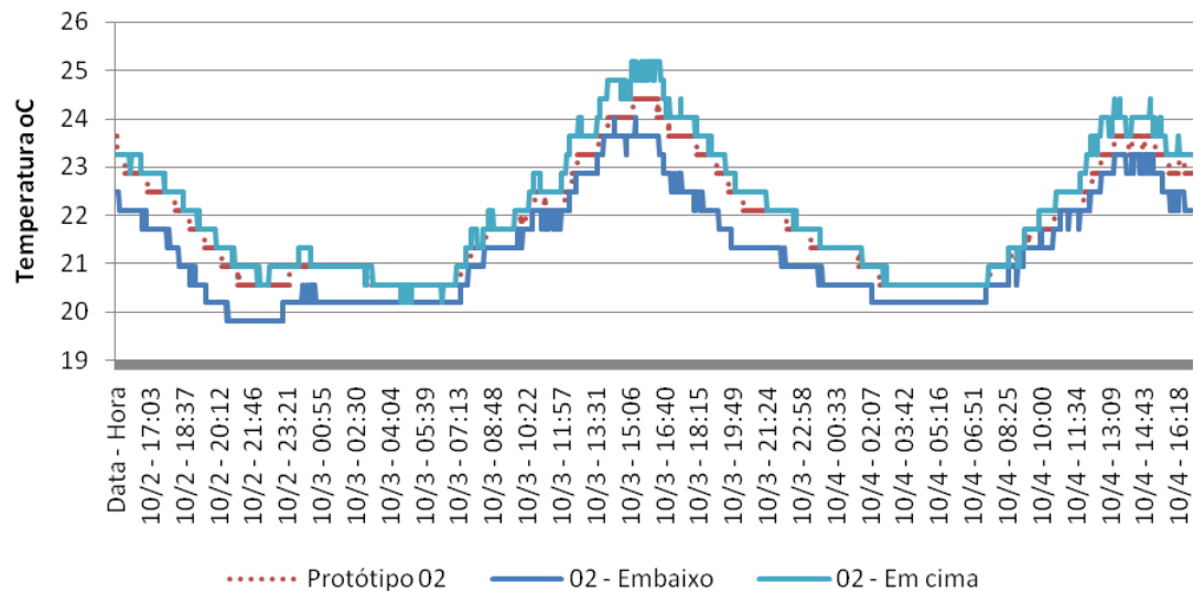
Gráfico 15 – Temperaturas no interior do protótipo 2, demonstrando o processo de estratificação do ar com cobertura vegetal
