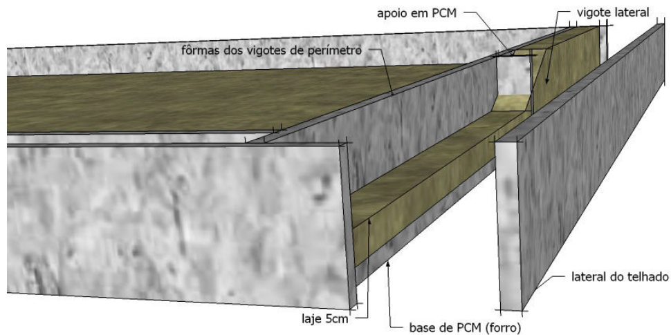
Figura 40 – Detalhe de montagem prévia da laje de cobertura
