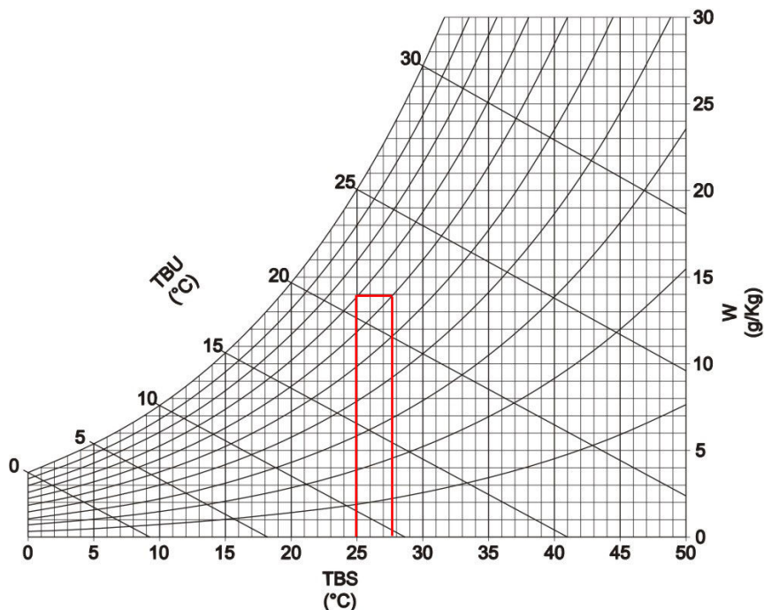
Gráfico 4 - Curva psicrométrica simplificada
