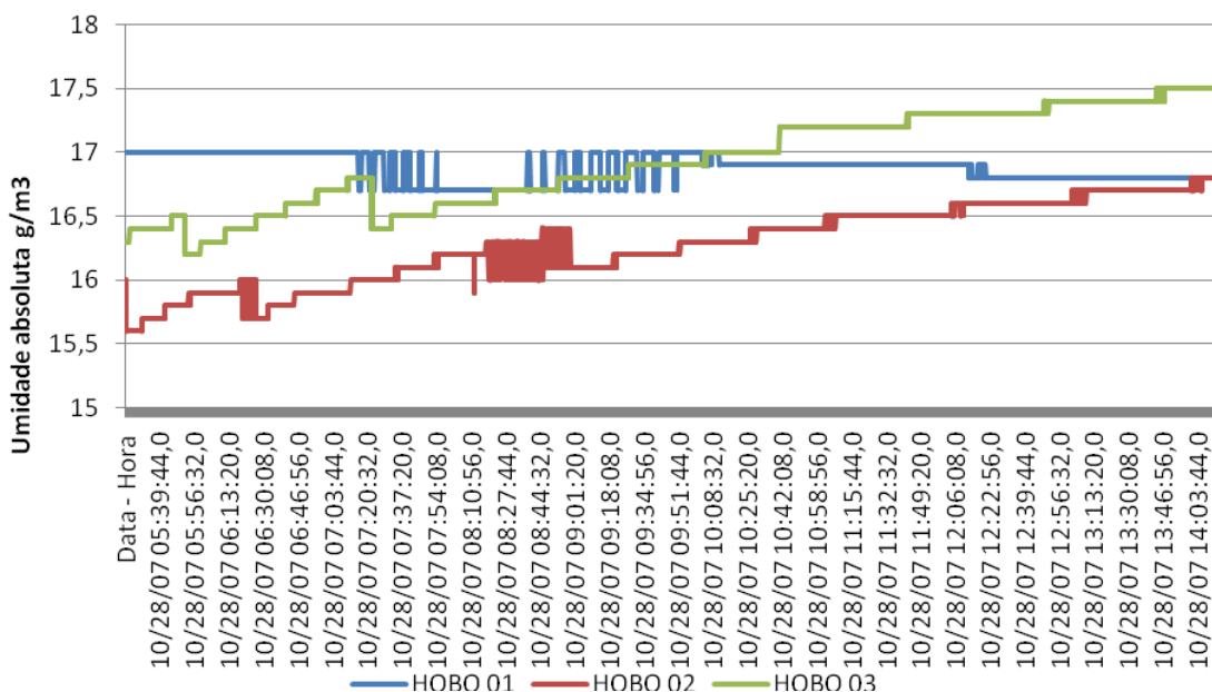
Gráfico 7 - Umidades absolutas obtidas pelos três aparelhos dentro da caixa térmica
