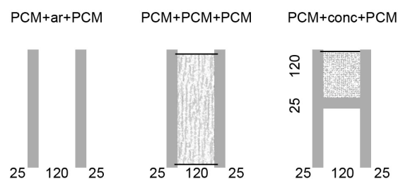
Figura 63 - Diferentes seções das paredes de PCM (unidades em mm)
