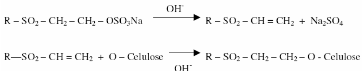
FIGURA 3 – Processo de tintura do algodão contendo o grupo sulfatoetilsulfonila como centro reativo da molécula.
