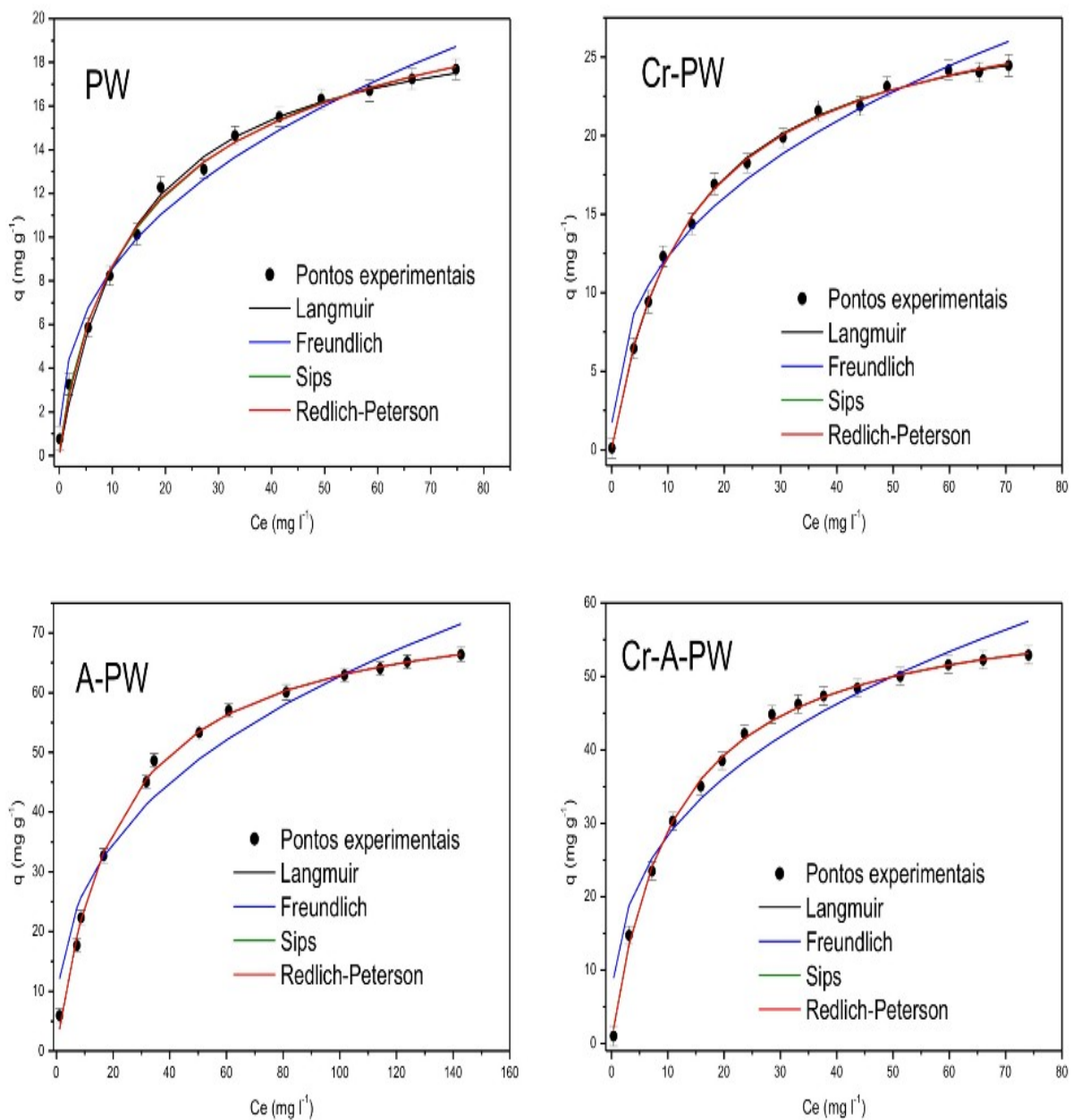
FIGURA 17 - Modelos de isothermas para remoção do HRR de soluções aquosas. Condições: concentração inicial dos corantes 25 \text{ mg L}^{-1} , temperatura de 25^\circ\text{C} , \text{pH}=2 e dosagem de biossorvente de 5,0 \text{ g L}^{-1} .
