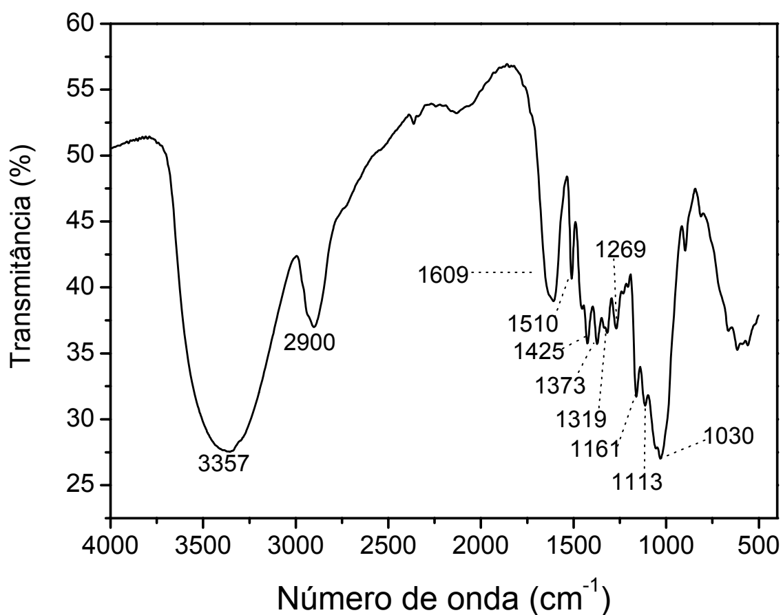
FIGURA 7 – Espectro de FTIR do resíduo de pinhão.
