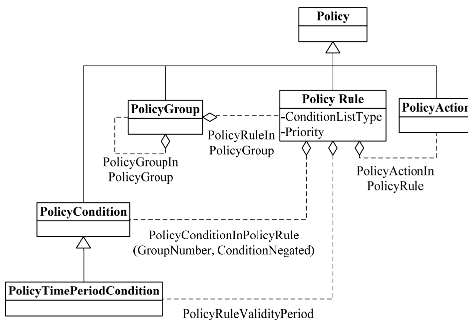
Figura 4.1: Principais classes do modelo PCIM
