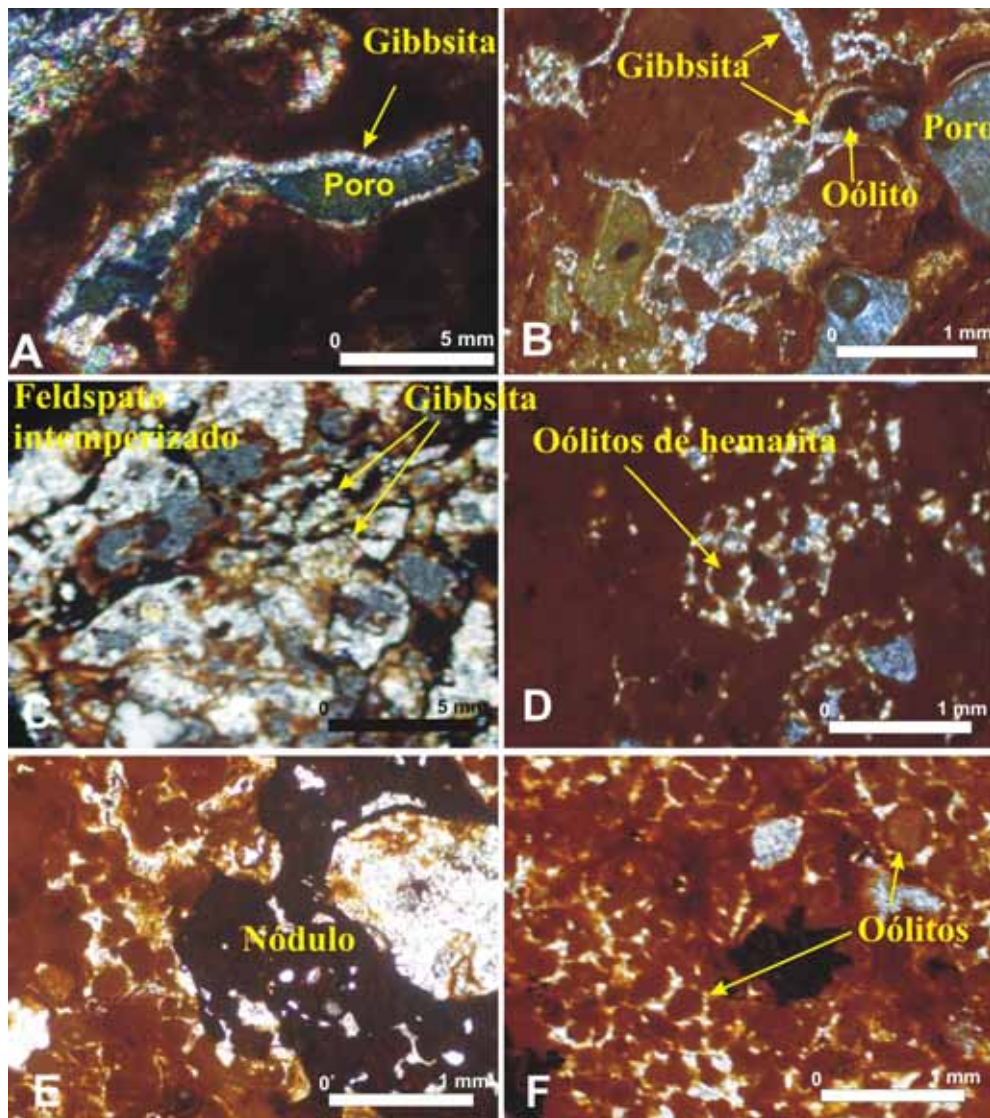
Figura 24 – Feições microscópicas da crosta do perfil 3. A – Gibbsita microcristalina perpendicular a parede do poro; B – camadas concêntricas de gibbsita ao redor dos nódulos; C – feldspato em estágio avançado de intemperismo; D – oólitos de hematita no interior de um alteromorfo de gibbsita; E e F – nódulo de hematita e individualização de vários oólitos na crosta ferro-aluminosa.
