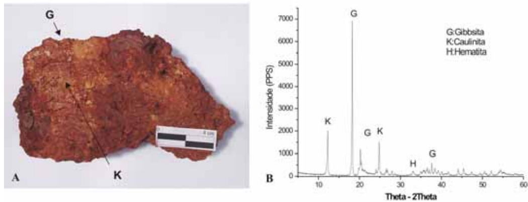
Figura 23 – Saprolito do perfil 3. A – fragmento do topo do saprolito; B – difratograma de raios-X com a identificação das reflexões dos principais minerais presentes no saprolito.
