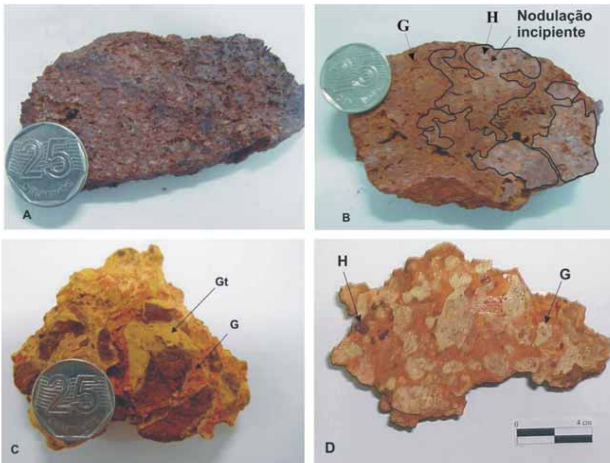
Figura 19 – Feições macroscópicas do perfil 2. A – saprolito poroso com foliação e lineamento preservados; B – crosta aluminosa protonodular; C – crosta aluminosa protopisolítica; D – crosta aluminosa pisolítica. (Gt = goethita, G = gibbsita, H = hematita).
