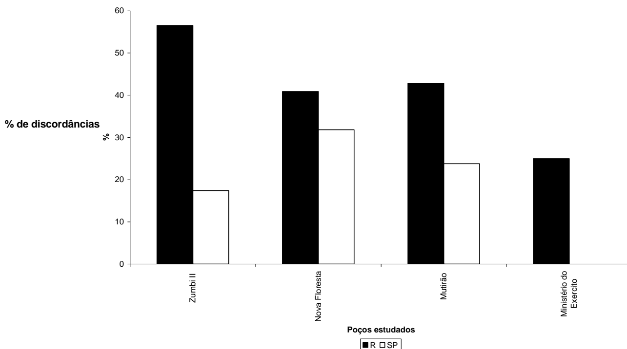
Gráfico 9 – Quantitativo das discordâncias observadas nos perfis geofísicos estudados considerando o fluido misto.
