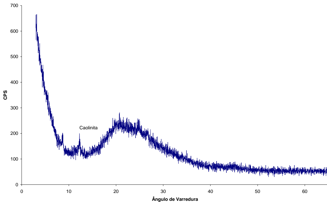
Gráfico 5- Difractometria de raios X do fluido misto.
