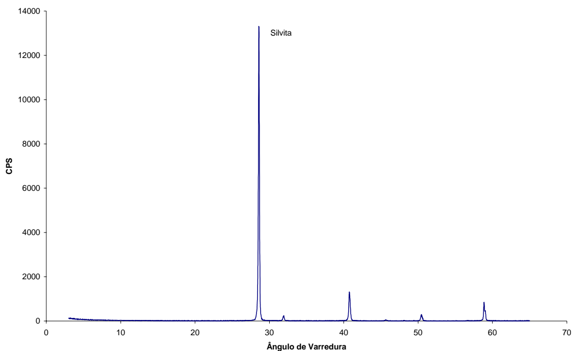
Gráfico 3 - Difratometria de raios X do Drillvis a seco
