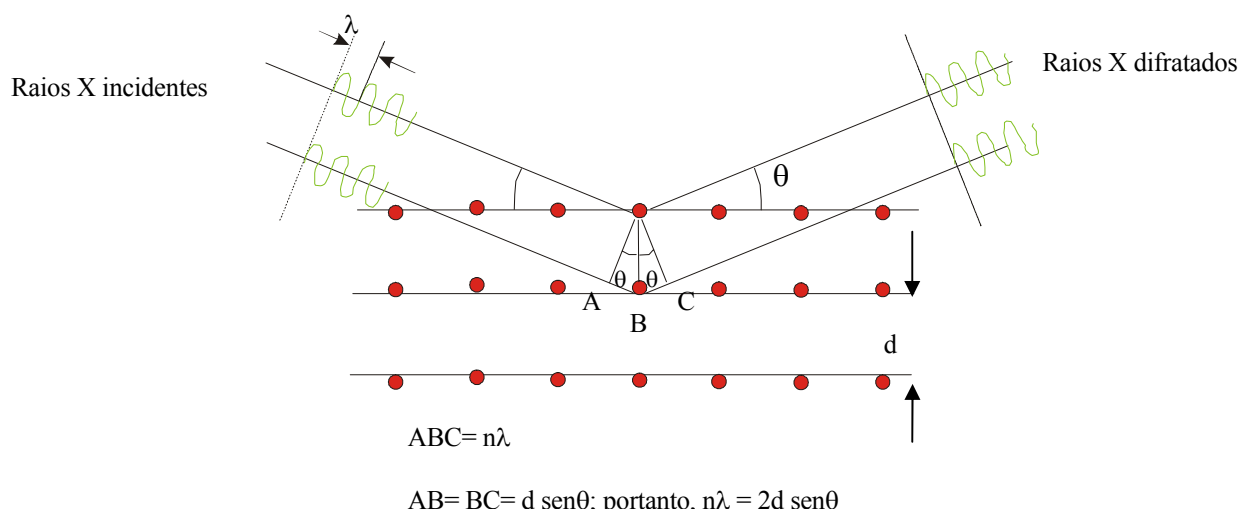
Figura 6 – Geometria da difração de raios X – Lei de Braag. Fonte: UNIVERSIDADE FEDERAL DE SANTA MARIA, 2006.
