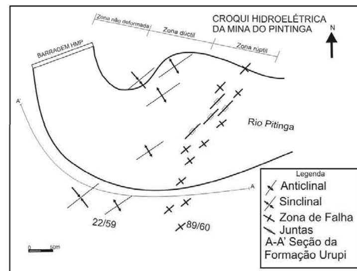
Figura 4.5. Perfil ao longo do Rio Pitinga, área da HMP, representada pela seção (A-A', associação de lençóis arenosos/ wadi ) e sua fotointerpretação. Medidas de juntas, falhas e eixo de dobras são mostrados respectivamente nos diagramas A, B e C. A foto acima as dobras são encontradas na estrada para Vila do Pitinga (ponto 5) com direção dos planos axiais similares aos encontrados na HMP. Ao lado, o mapa da HMP, indicando a seção A-A' e posicionamento das estruturas geológicas.
