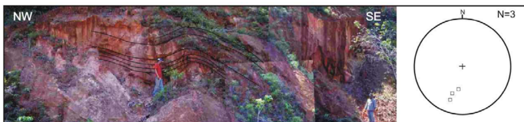
Figura 4.5. Perfil ao longo do Rio Pitinga, área da HMP, representada pela seção (A-A', associação de lençóis arenosos/ wadi ) e sua fotointerpretação. Medidas de juntas, falhas e eixo de dobras são mostrados respectivamente nos diagramas A, B e C. A foto acima as dobras são encontradas na estrada para Vila do Pitinga (ponto 5) com direção dos planos axiais similares aos encontrados na HMP. Ao lado, o mapa da HMP, indicando a seção A-A' e posicionamento das estruturas geológicas.
